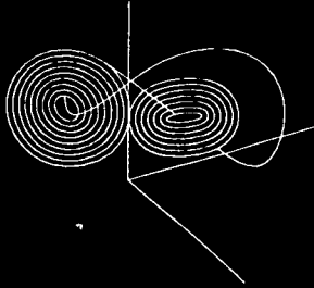
FIGURA 9. UNA LÍNEA DEL ATRACTOR DE LORENZ
