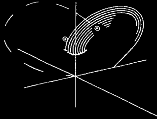
FIGURA 10. LOS PUNTOS CLAVES PARA INICIAR EL EFECTO MARIPOSA A LA INVERSA
