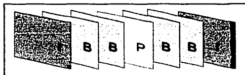
Figura 2.9 Estructura típica de un grupo de imágenes empleando las tramas I, B y P.
