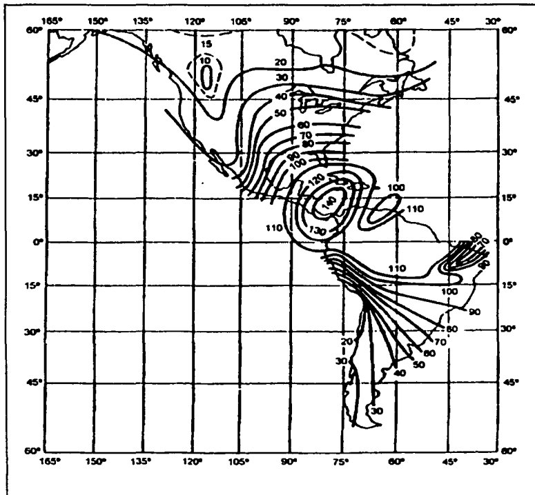
Figura A.3 Contornos de intensidad de lluvia en mm/h que es excedida durante 0.01% del tiempo en un año según la CCIR.
