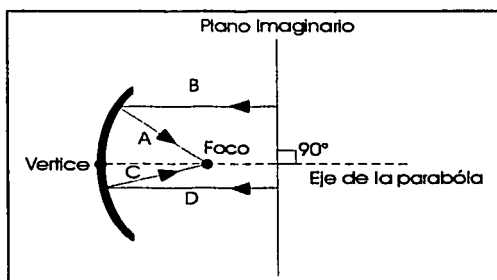
Figura 4.1 Estructura del un plato parabólico. La distancia A + B es la misma que la distancia C + D .
