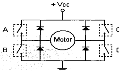
Fig. II.5.-Esquema del puente H
