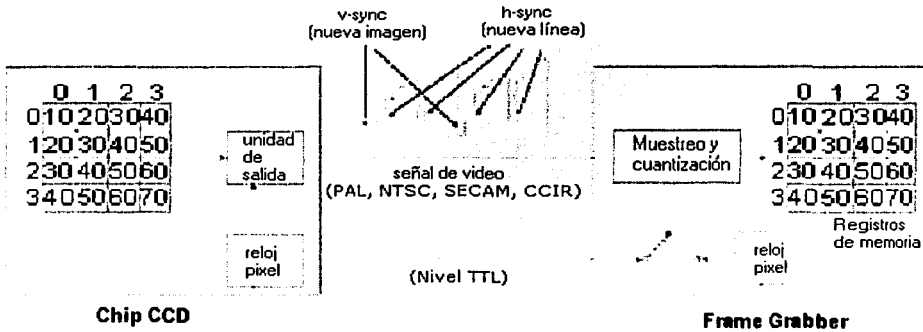
Fig. II.13.-Esquema del conjunto CCD-FrameGrabber
