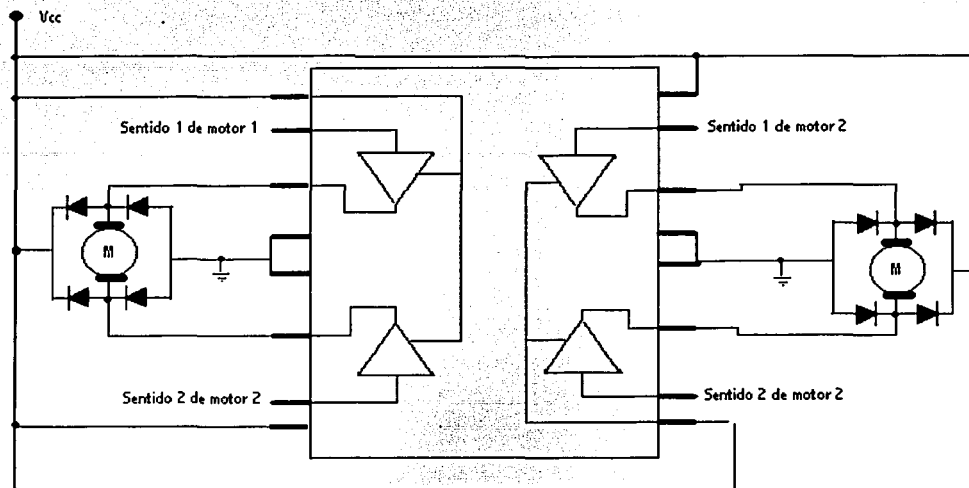
Fig. III.15.-Diagrama de la etapa de potencia (puentes H L293B) para el zoom y foco.
