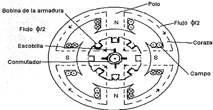
Fig. II.2.- Trayectorias del flujo dentro de una máquina de CD de 4 polos(B2).
