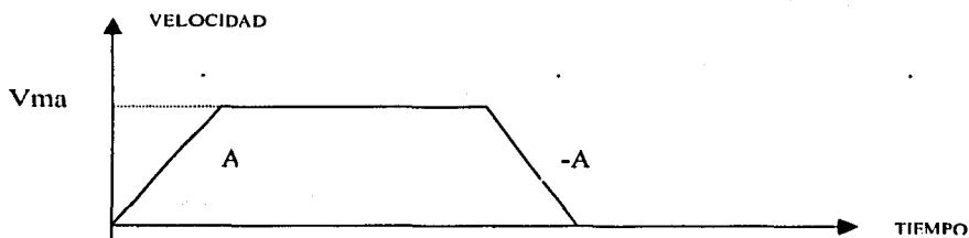
Fig. III.4.- Perfil de velocidad generado por el LM629
