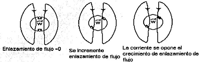
Fig. II.3.- Determinación de polaridades de la FEM generada por medio de la ley de Lenz
