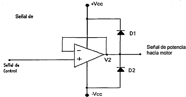
Fig. II.7.-Amplificador operacional de potencia
