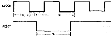
FIG 3. TIEMPO DE RELOJ Y RESET
