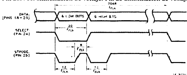
FIG 8. TIEMPO DE SALIDA DE BIT MULTIPLEXADO
