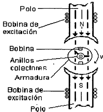
Fig. II.1- Configuración básica del motor de CD(B2).
