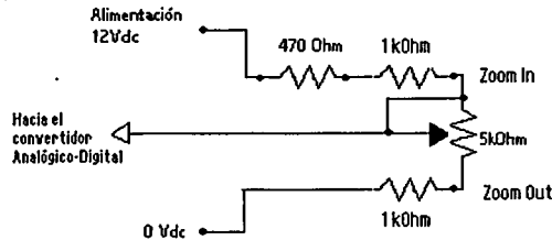
Fig. III.13.- Circuito usado para conocer la posición del zoom.
