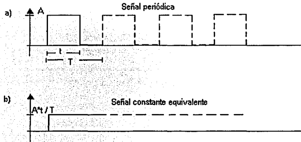
Fig.II.4 Modulación por Ancho de Pulso
