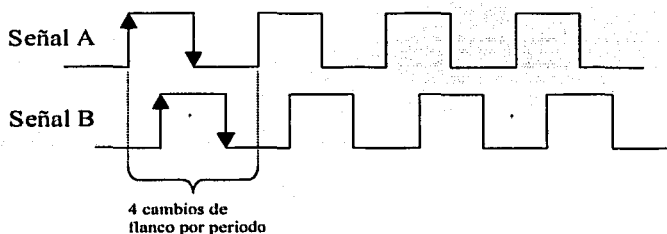
Figura II.7.-Salidas del codificador de posición incremental Accu-Codder
