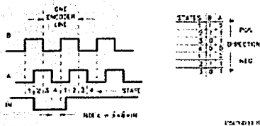
FIG 9. SEÑALES DEL CODIFICADOR EN CUADRATURA
