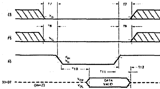
FIG 4. TIEMPO DEL BYTE DE ESTADO
