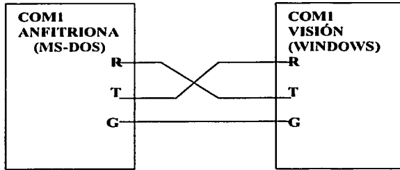
Fig.IV.1.-Conexión serial entre computadoras
