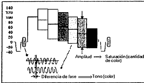
Fig. II.12.-Forma de onda de video compuesto: barras de color
