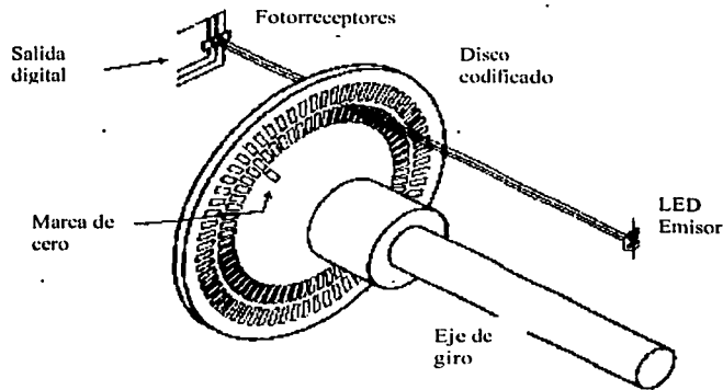
Fig. II.8.-Codificador Incremental (E9)
