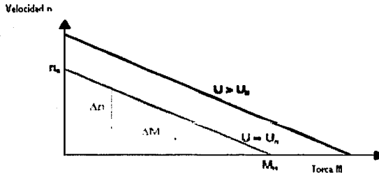
Fig.III.3.-Línea Velocidad-Torca
