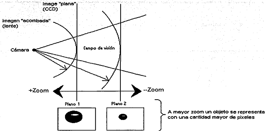
Fig.IV.13.-Consideraciones de posicionamiento automático
