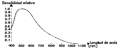
Fig. II.10.-Respuesta Espectral de un sensor CCD
