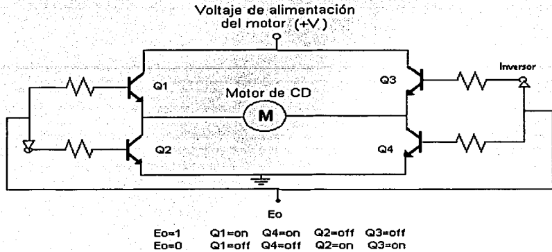
Fig.II.6.-Implementación con transistores de un Puente H
