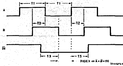
FIG 2. TIEMPO DE CUADRATURA DEL CODIFICADOR
