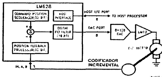
FIG 1. DIAGRAMA DE BLOQUES
