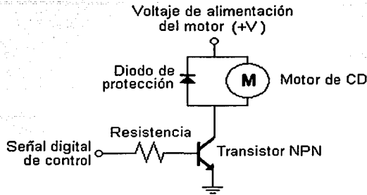
Fig.II.5.-Circuito básico para encender un motor de DC
