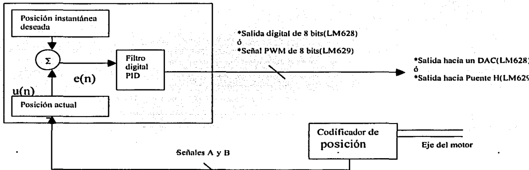
Fig. III.5.- Esquema de control del LM629
