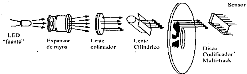
Fig. II.9.-Codificador Absoluto (E9)
