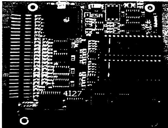
Fig. II.6.- Tarjeta controladora 4127
