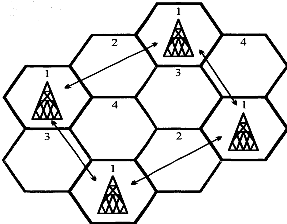
Figura I.12: Ilustración de la Interferencia de Canal Propio en un Arreglo Celular típico.
