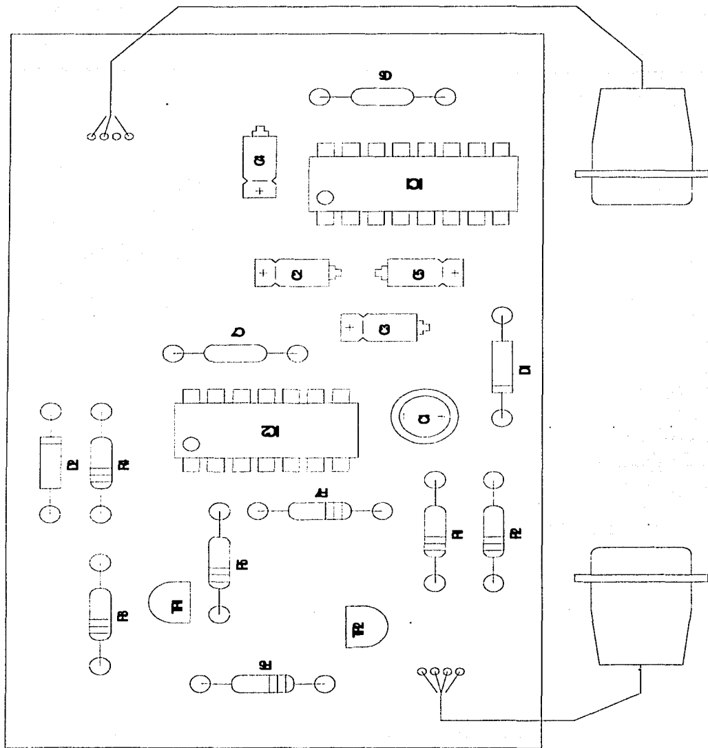
Figura IV.6: Circuito Impreso V/I.
