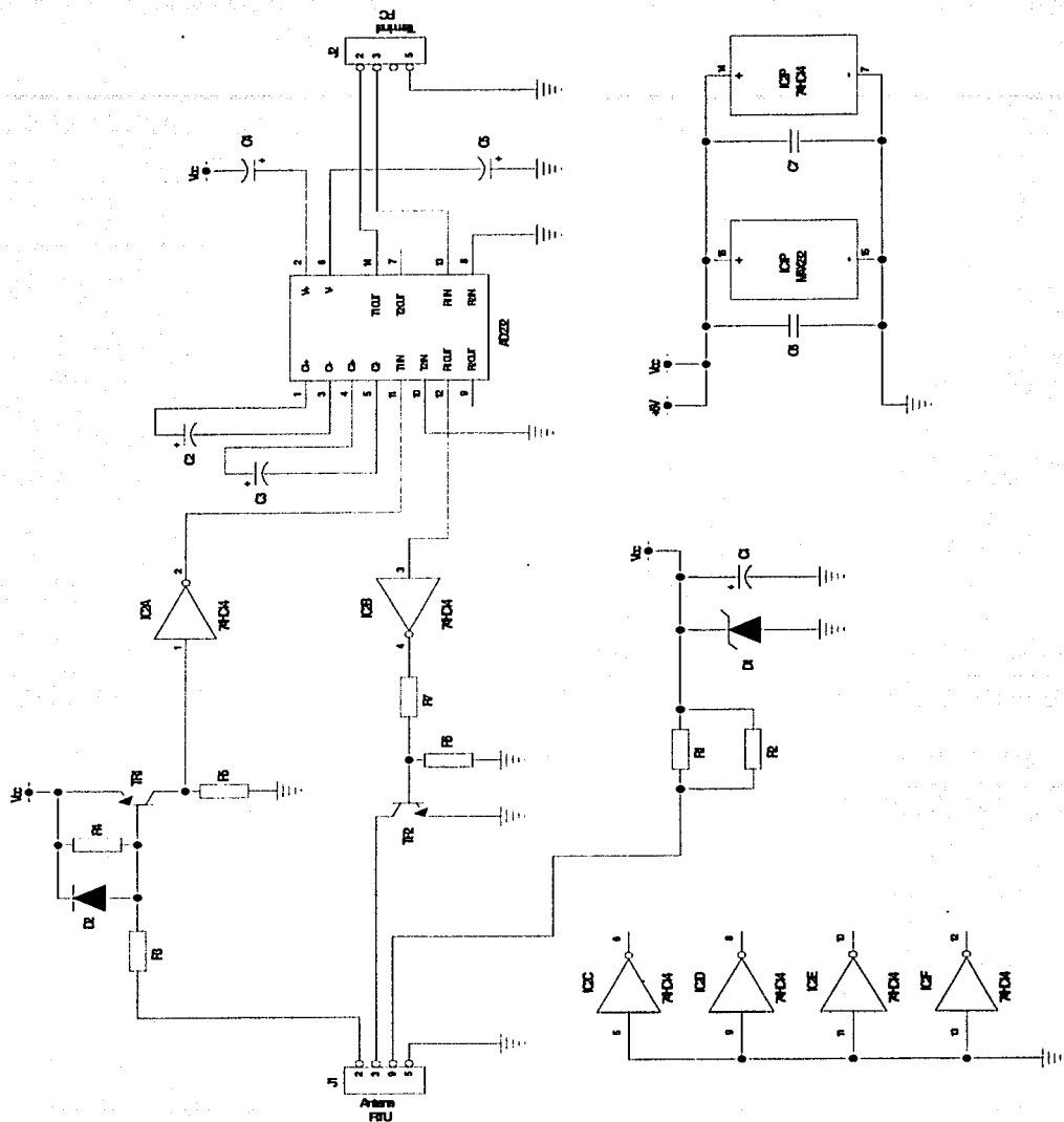
Figura IV.5: Diagrama Esquemático del circuito V/I
