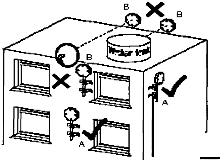
Figura II.14: Colocación de la RTU.
