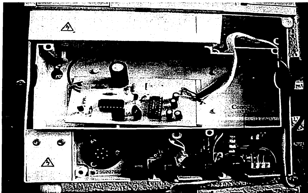
Figura IV.8: Circuito V/I en la RPCU.
