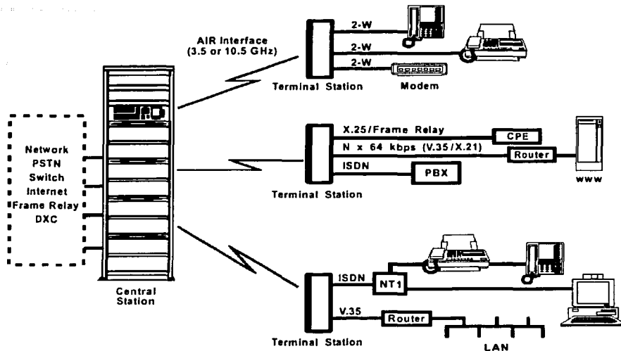
Figura II.2: Elementos / Interfaces del Sistema de Acceso Fijo Inalámbrico.
