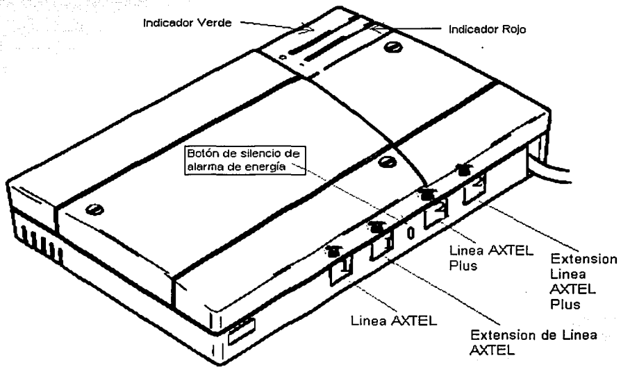
Figura II.5: Fuente de Poder (RPCU).
