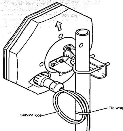
Figura II.3: Antena (RTU).
