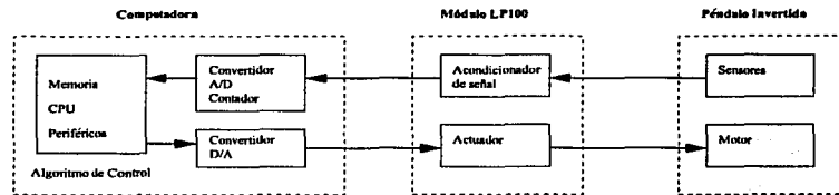
Figura 1.2: Flujo de señales entre la PC y el péndulo
