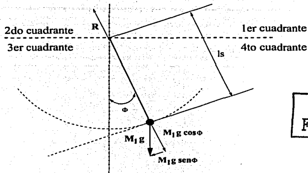
Figura 4.1: Esquema de un péndulo fijo sin fricción
