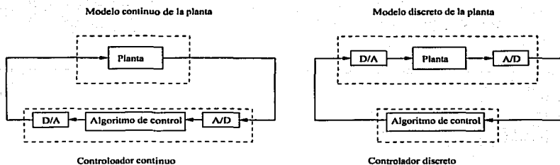
Figura 2.4: Esquemas para diseñar en el tiempo continuo (izquierda) y en el discreto (derecha)
