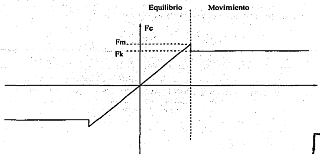
Figura 2.3: Fricción seca o de Coulomb
