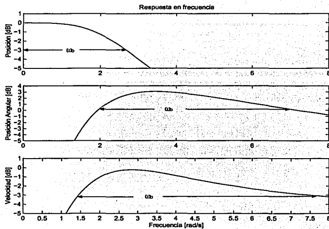
Figura 3.2: Respuesta en frecuencia de las diferentes salidas del sistema en lazo cerrado cuando se considera la referencia en la posición como la entrada del sistema.
