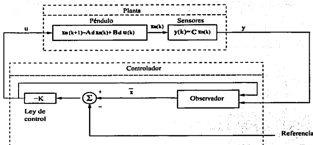
Figura 3.1: Diseño en espacio de estados
