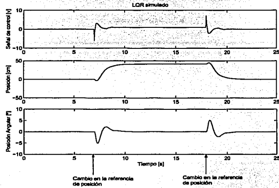
Figura 3.8: Simulación del algoritmo de control usando LQR estimando la fricción
