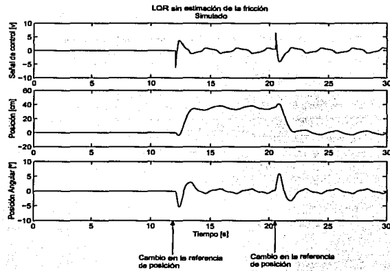
Figura 3.10: Simulación del algoritmo de control usando LQR sin estimar la fricción
