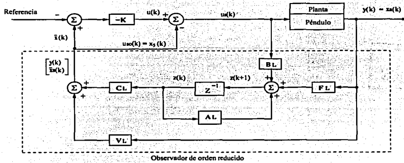
Figura 3.4: Esquema del controlador para estabilizar el péndulo
