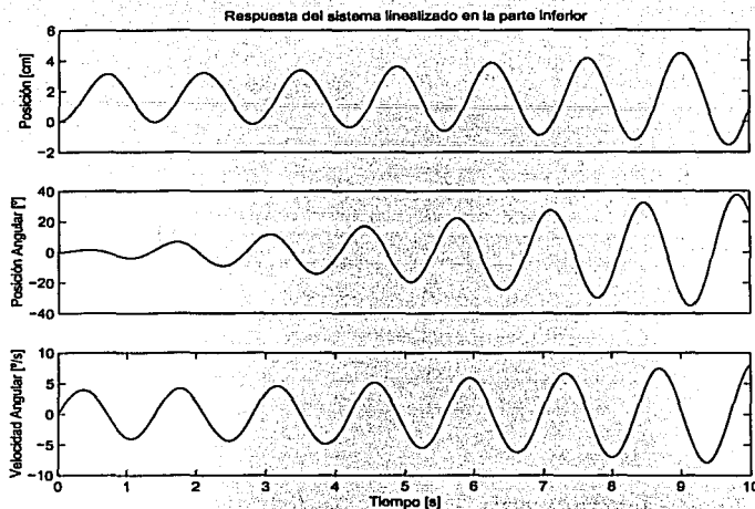
Figura 4.3: Péndulo invertido en resonancia
