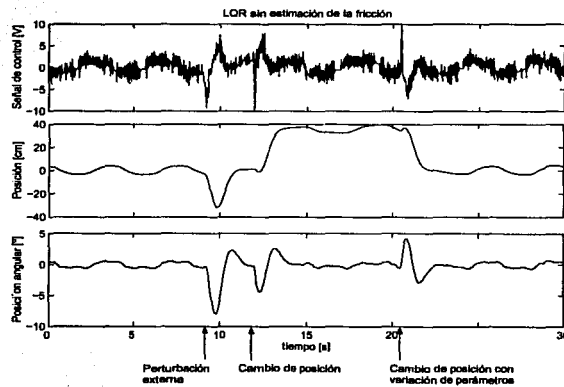
Figura 3.11: Resultados del algoritmo de control usando LQR sin estimar la fricción
