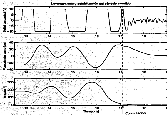
Figura 4.8: Levantamiento y estabilización del péndulo invertido usando LQR para el control del carro
