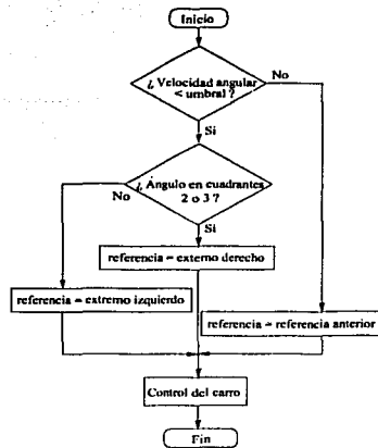
Figura 4.4: Diagrama de flujo para determinar la referencia del controlador del carro
