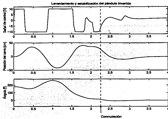
Figura 4.7: Simulación del conmutador y los controles para levantar y estabilizar el péndulo invertido
