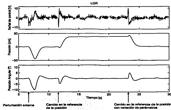
Figura 3.9: Resultados del algoritmo de control usando LQR estimando la fricción
