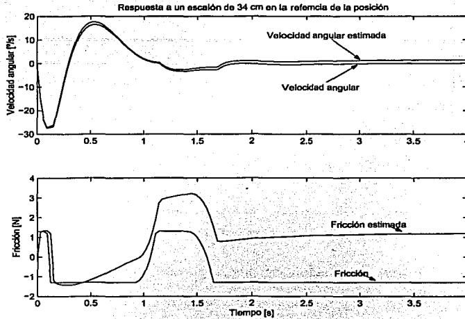
Figura 3.6: Simulación de la señales de velocidad angular, fricción y sus respectivos estimados al aplicar un escalón en la referencia de la posición
