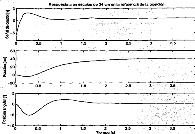
Figura 3.5: Simulación de la señal de control, la posición y la posición angular al aplicar un escalón en la referencia de la posición
