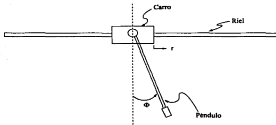
Figura 4.2: Péndulo en la posición inferior
