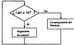
Figura 4.5: Diagrama de flujo para conmutar entre el levantamiento del péndulo y su estabilización
