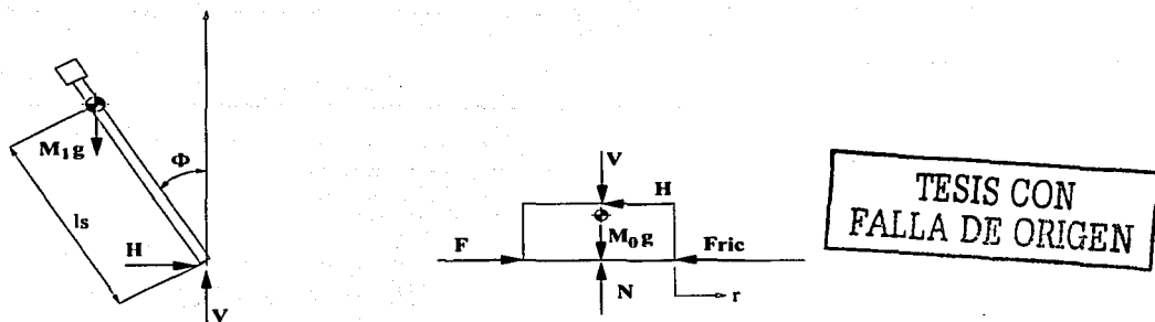
Figura 2.2: Diagramas de cuerpo libre del péndulo (izquierda) y del carro (derecha)
