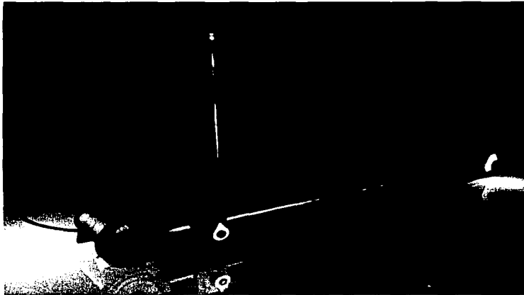
Figura 1.3: Perspectiva del péndulo invertido
