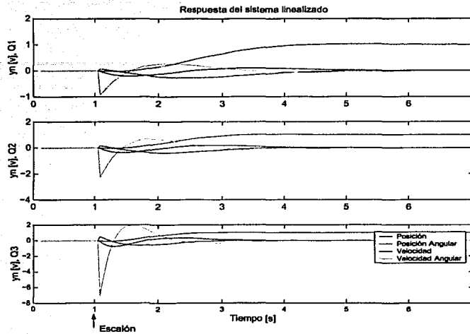
Figura 3.12: Respuestas del sistema para diferentes Q
