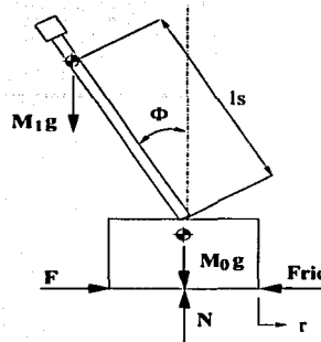
Figura 2.1: Diagrama de cuerpo libre del péndulo invertido
