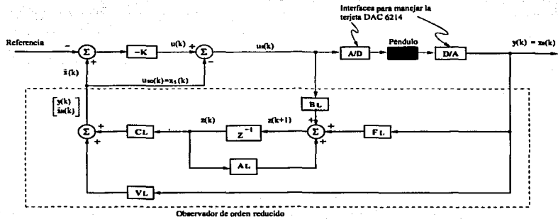
Figura 3.7: Implementación del controlador para estabilizar el péndulo
