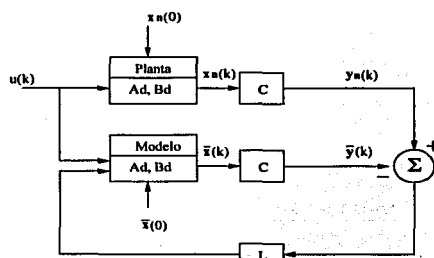
Figura 3.3: Observador de Luenberger
