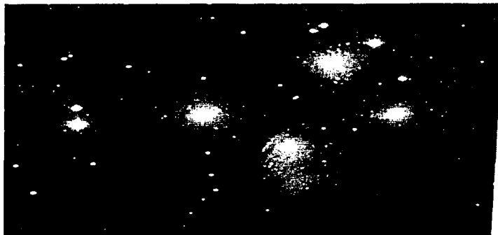
Pléyades (Sagan, 1980)
