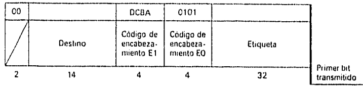
Figura 40.- Mensaje de prueba de conjunto de rutas de señalización
