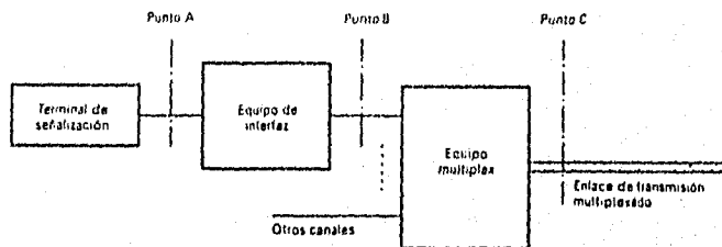
b) Ejemplo 2 - Enlace de datos de señalización (digital o analógico) mediante equipo de interfaz
