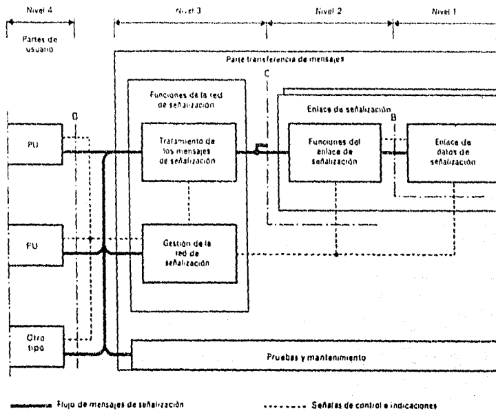
Figura 15.- Estructura general de las funciones del sistema de señalización
