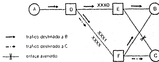
Figura 28.- Ejemplo de compartición de la carga entre conjuntos de enlaces
