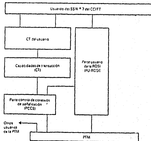
Figura 2.- Arquitectura del sistema de señalización nº 7
