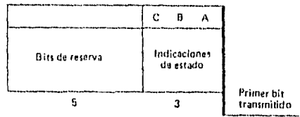
Figura 22.- Formato del campo de estado
