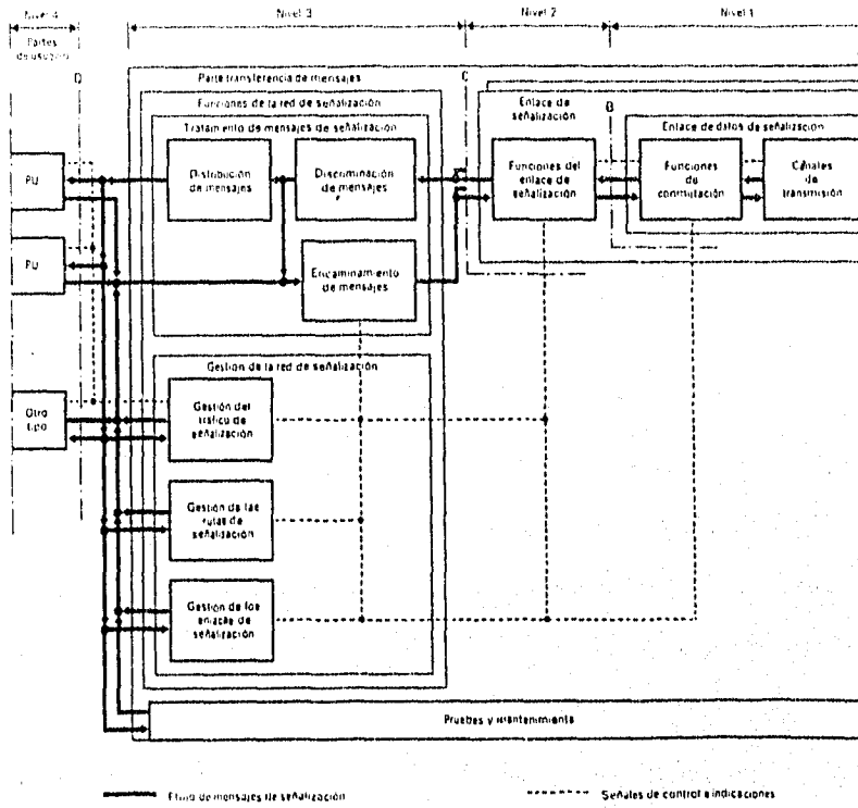
Figura 17.- Estructura detallada de las funciones del sistema de señalización
