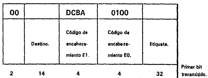
Figura 38 .- Mensaje de transferencia prohibida.
