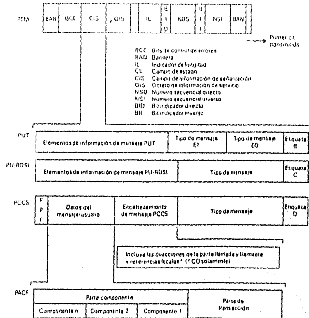
Figura 11.- Estructura del SS7
