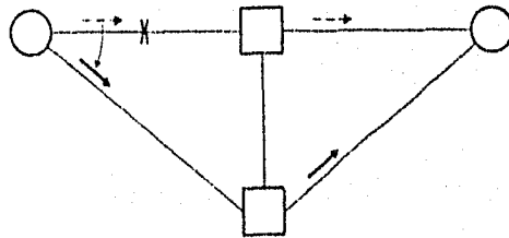
Figura 31.- Ejemplo de paso a enlace de reserva utilizando una ruta de señalización que no atraviesa el punto de señalización distante
