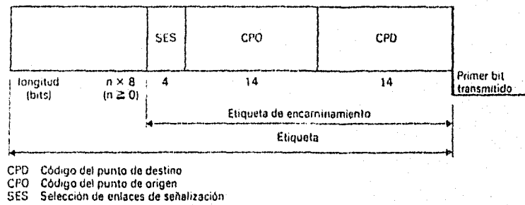
Figura 26.- Estructura de la etiqueta de encaminamiento
