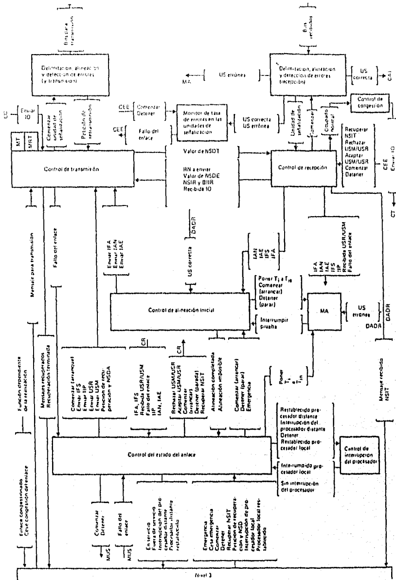
Figura 23.- Diagrama de bloques funcionales del nivel 2
