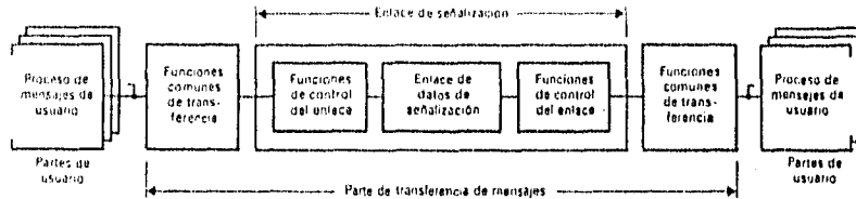
Figura 14.- Diagrama funcional del sistema de señalización por canal común
