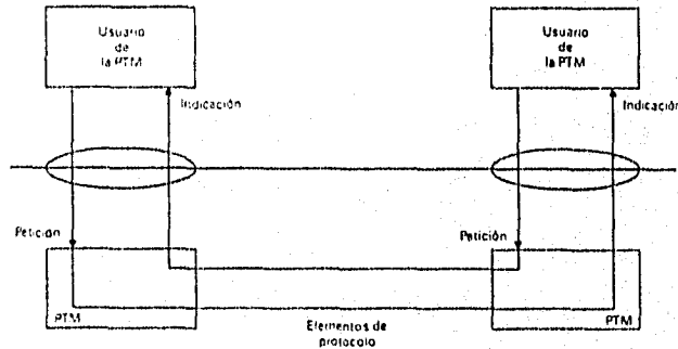
Figura 13.- Nombres específicos de las primitivas y comunicación de par a par
