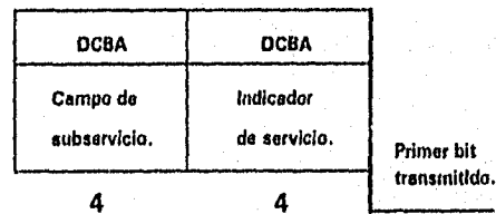
Figura 33.- Octeto de información de servicio.
