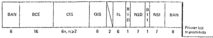
a) Formato básico de una unidad de señalización de mensaje (USM)
