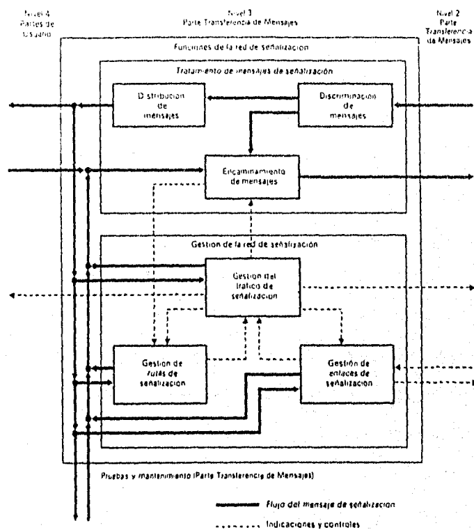
Figura 24.- Funciones de la red de señalización
