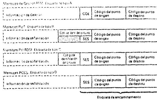
Figura 10. - Tipos de etiqueta de mensajes de SS7
