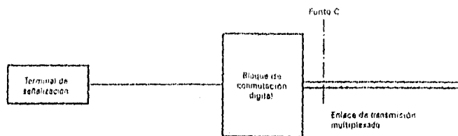
a) Ejemplo 1 - Enlace de datos de señalización digital mediante un bloque de conmutación digital
