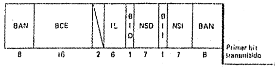
c) Formato de la unidad de señalización de relleno (USR)
