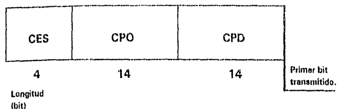
Figura 34 .- Estructura normalizada de la etiqueta.
