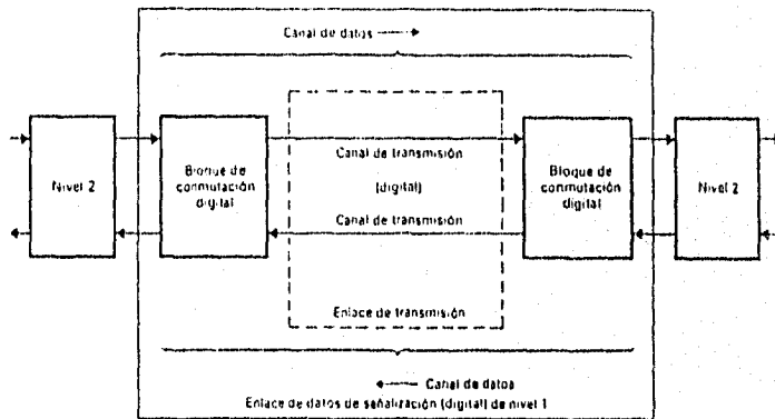
a) Ejemplo 1 - Enlace digital de datos de señalización mediante bloque de conmutación digital
