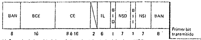
b) Formato de la unidad de señalización del estado del enlace (UEE)
