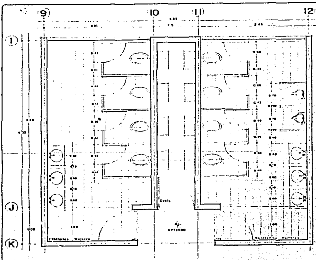
Planta Baños
