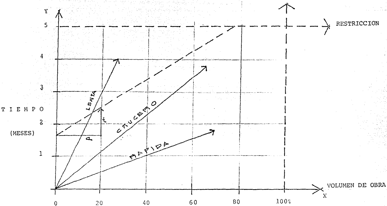
GRAFICA PARA DETERMINAR LA VELOCIDAD DE LA OBRA
