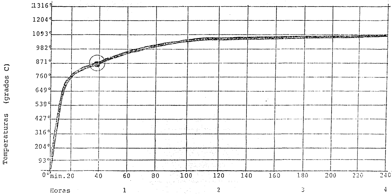
CURVA TEMPERATURA TIEMPO
