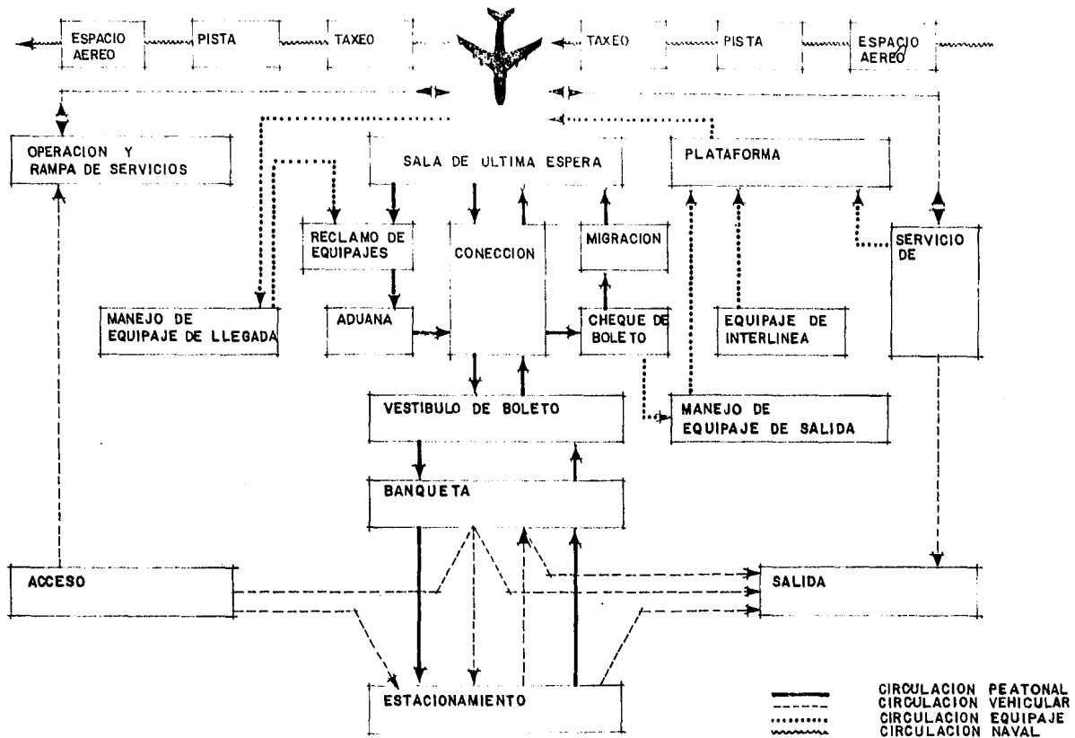
DIAGRAMA DE FLUIDOS
