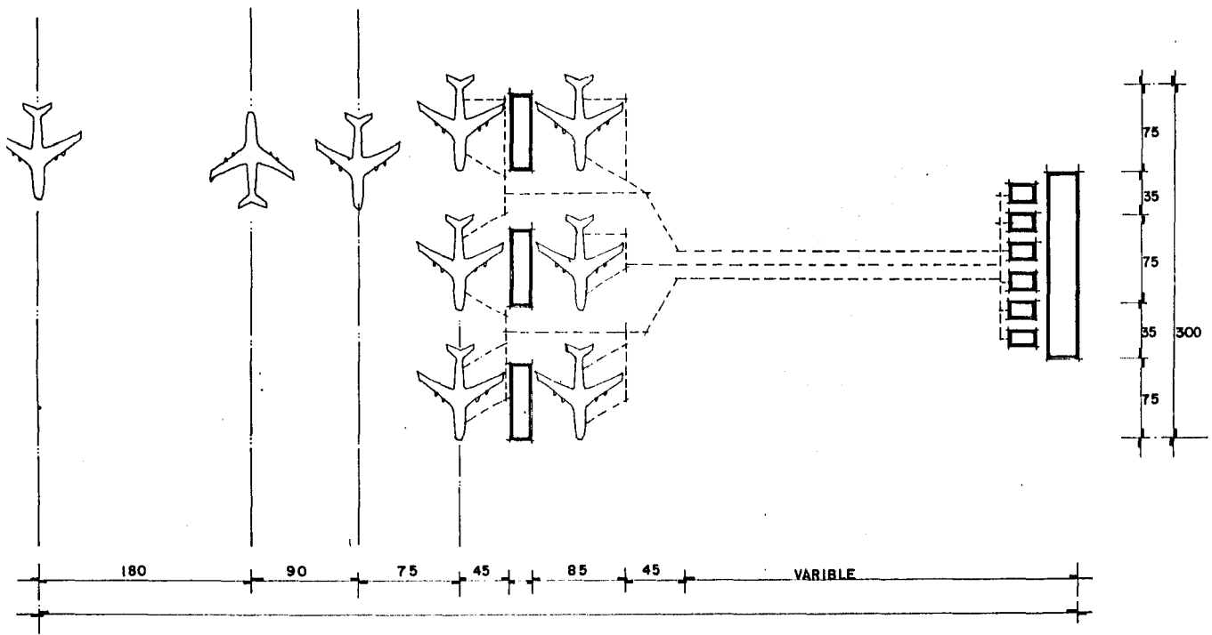
CONCEPTO TRANSPORTADOR
