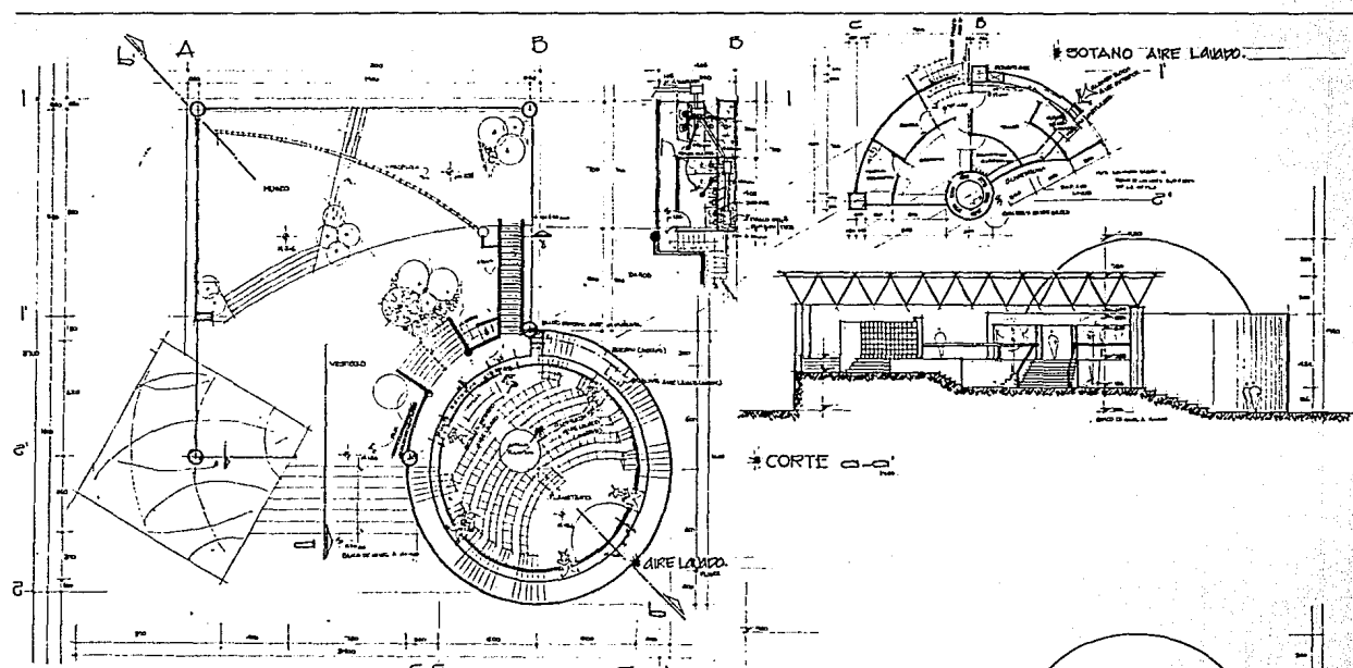
* PLANTA ARQUITECTONICA.
