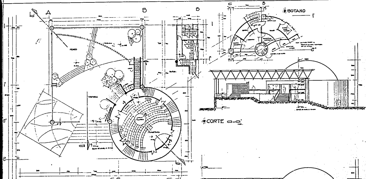
* PLANTA ARQUITECTONICA. Escala: 1:100
