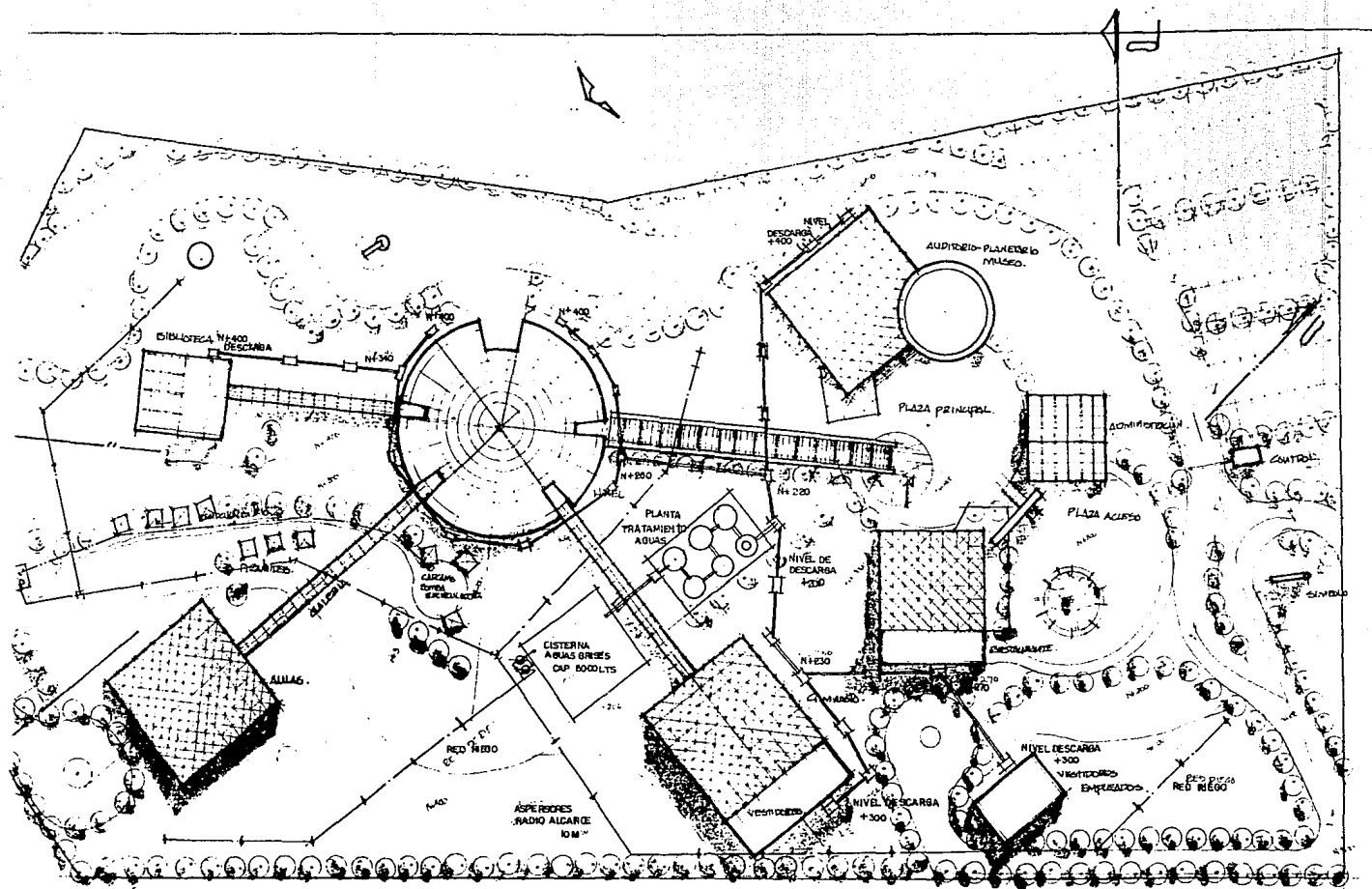
● PLANTA CONJUNTO. .modulacion conjunta.
