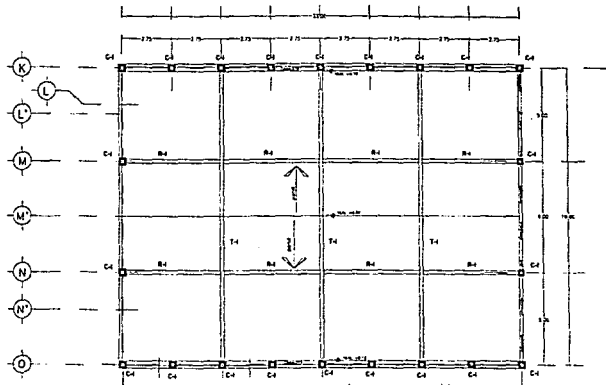
ARMADURA SALON DE USOS MULTIPLES
