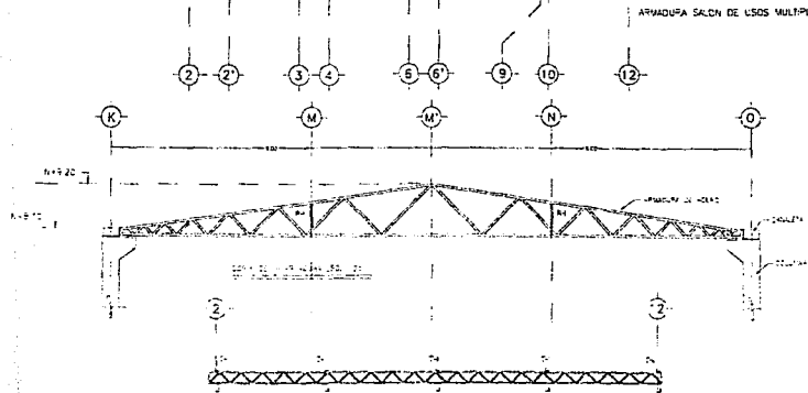
ARMADURA SALON DE USOS MULTIPLES
