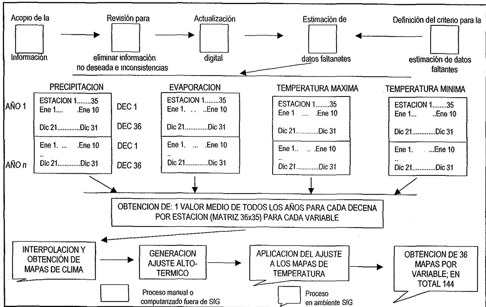
Figura 2.2. Diagrama empleado para procesar la base de datos de clima.
