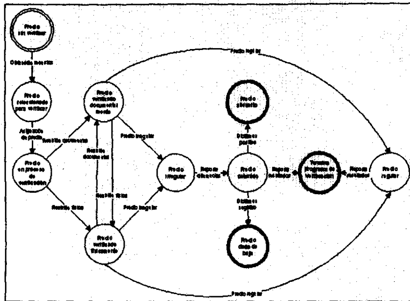
Figura 3.2.11 Diagrama de estados de la operación de un predio
