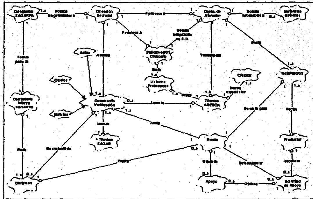
Figura 3.1.6 Diagrama de clases de la operación actual del mecanismo de verificación de predios en la Dirección Regional
