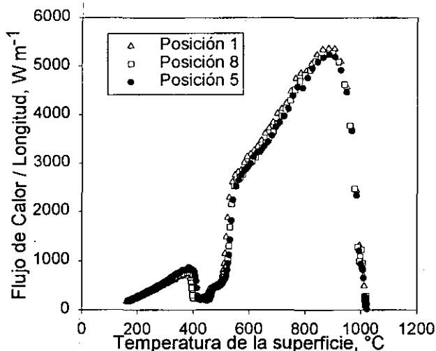
Figura 4.12 Flujo de calor por unidad de longitud en función de la temperatura para la corrida número 5. Para 2 pasos de tiempos futuros.
