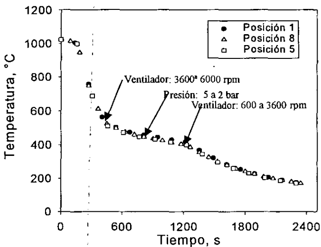
Figura 4.6 Curvas de enfriamiento en el centro de probetas de acero inoxidable de 1 in de diámetro, ubicadas en las posiciones 8, 5 y 1 (ver Figura 3.3). Corrida número 5.
