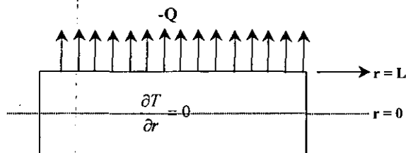
Figura 4.13 Representación esquemática de la aplicación del programa de cómputo CONDUCT en una sola dirección, en un cilindro de diámetro 2L . En x = 0 se tiene simetría ( \partial T / \partial r = 0 ), y en r = L la densidad de flujo de calor es conocida que son datos obtenidos por IHCP.
