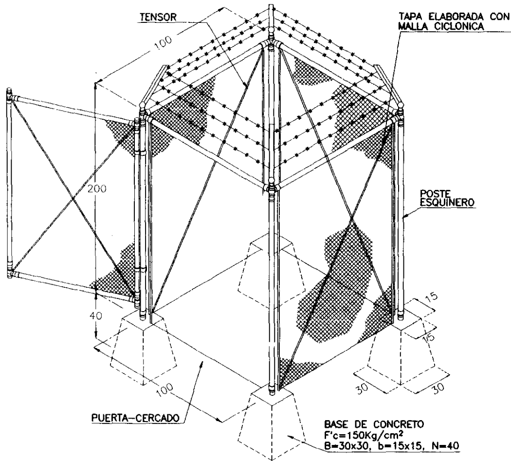
ISOMÉTRICO ( PROTECCION TIPO PARA VALVULA V.A.E.A. )
