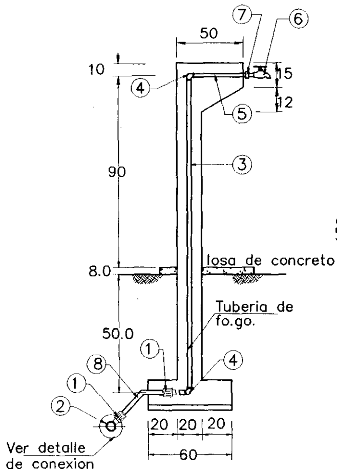
SECCION LATERAL
