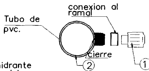
DETALLE DE CONEXION
