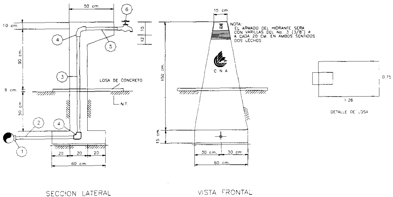
Figura 4.6 HIDRANTE PUBLICO.
