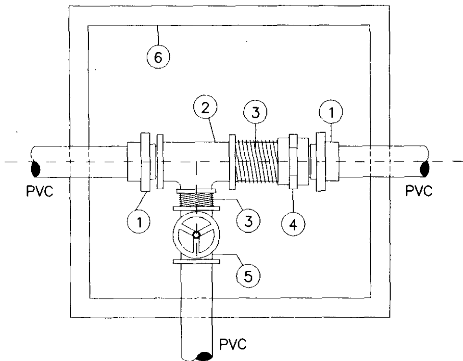
DETALLE DE INSTALACION DE DESAGÜE
