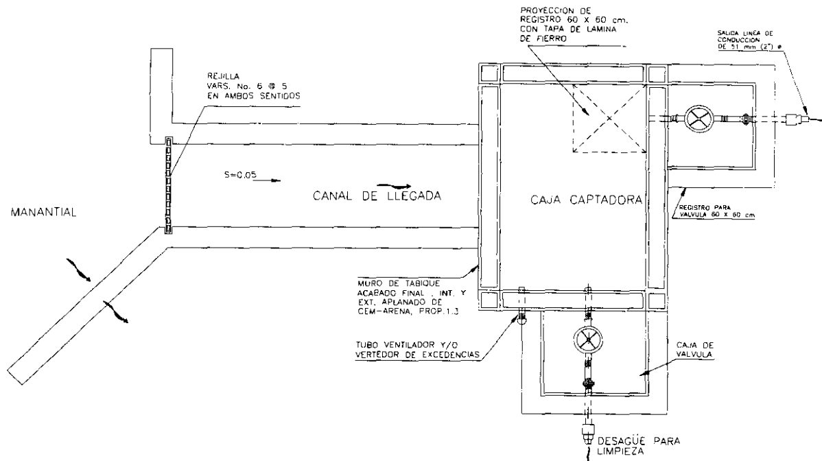
PLANTA
