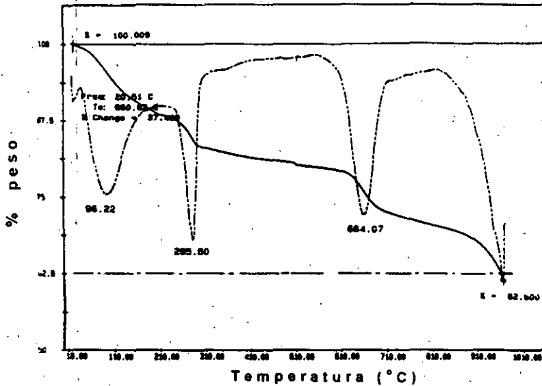
Figura III.1. Análisis termogravimétrico (TG) de la muestra ZrB(10)-5
