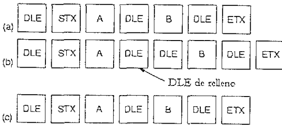
(a) Datos enviados por la capa superior (b) Datos después del relleno de caracteres por la capa de enlace de datos (c) Datos pasados a la capa superior del lado receptor
