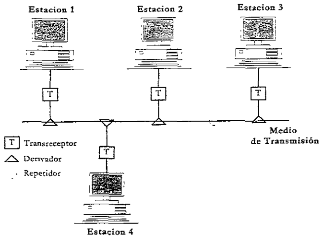
Figura 1-11 Componentes de una red de cable coaxial
