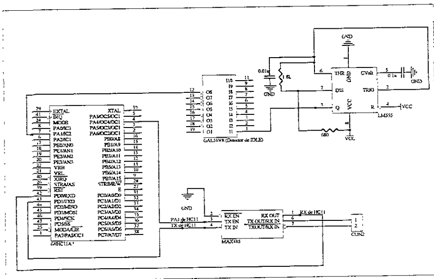
Figura 3-8 Circuito del detector de IDLE
