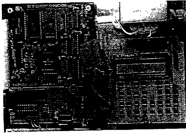
Figura 4-2 Estación "2" HC11
