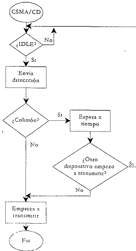
Figura 3-14 Algoritmo CSMA/CD
