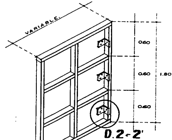
BASTIDOR Y ANGULO DE SOPORTE. Esc. 1:25
