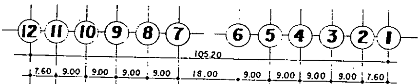
FACHADA SUR-OESTE.
