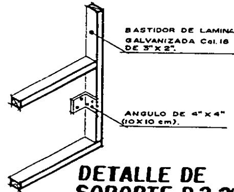
BASTIDOR Y ANGULO DE SOPORTE. Esc. 1:25
