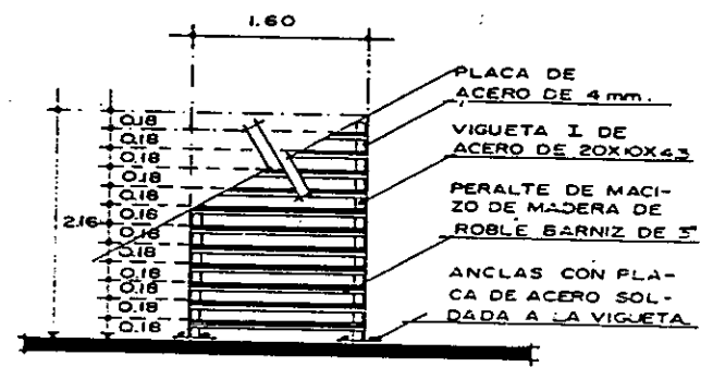
ALZADO. Esc. 1:50
