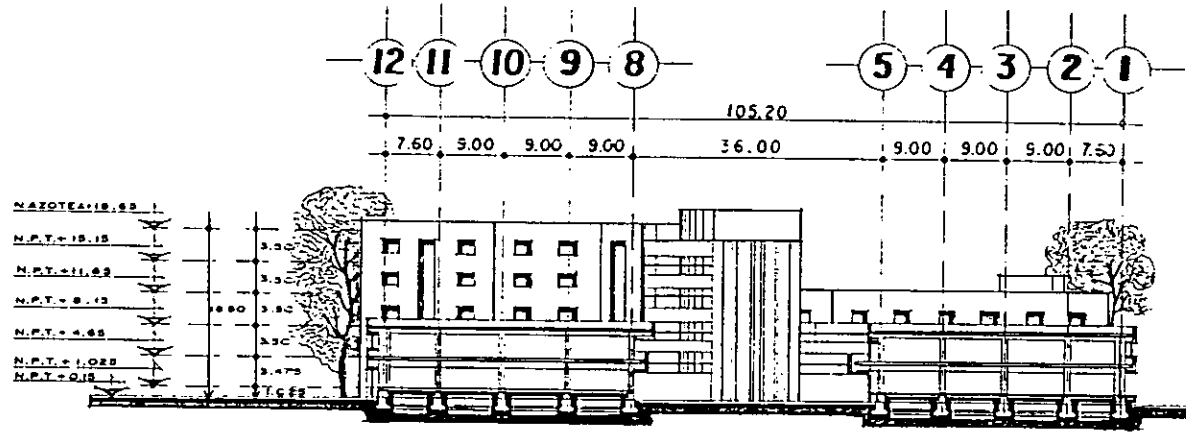
CORTE LONGITUDINAL. A-A'
