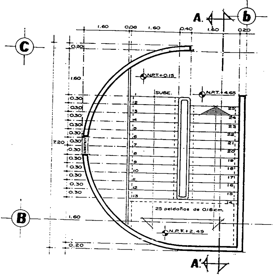
PLANTA DE ESCALERA.
