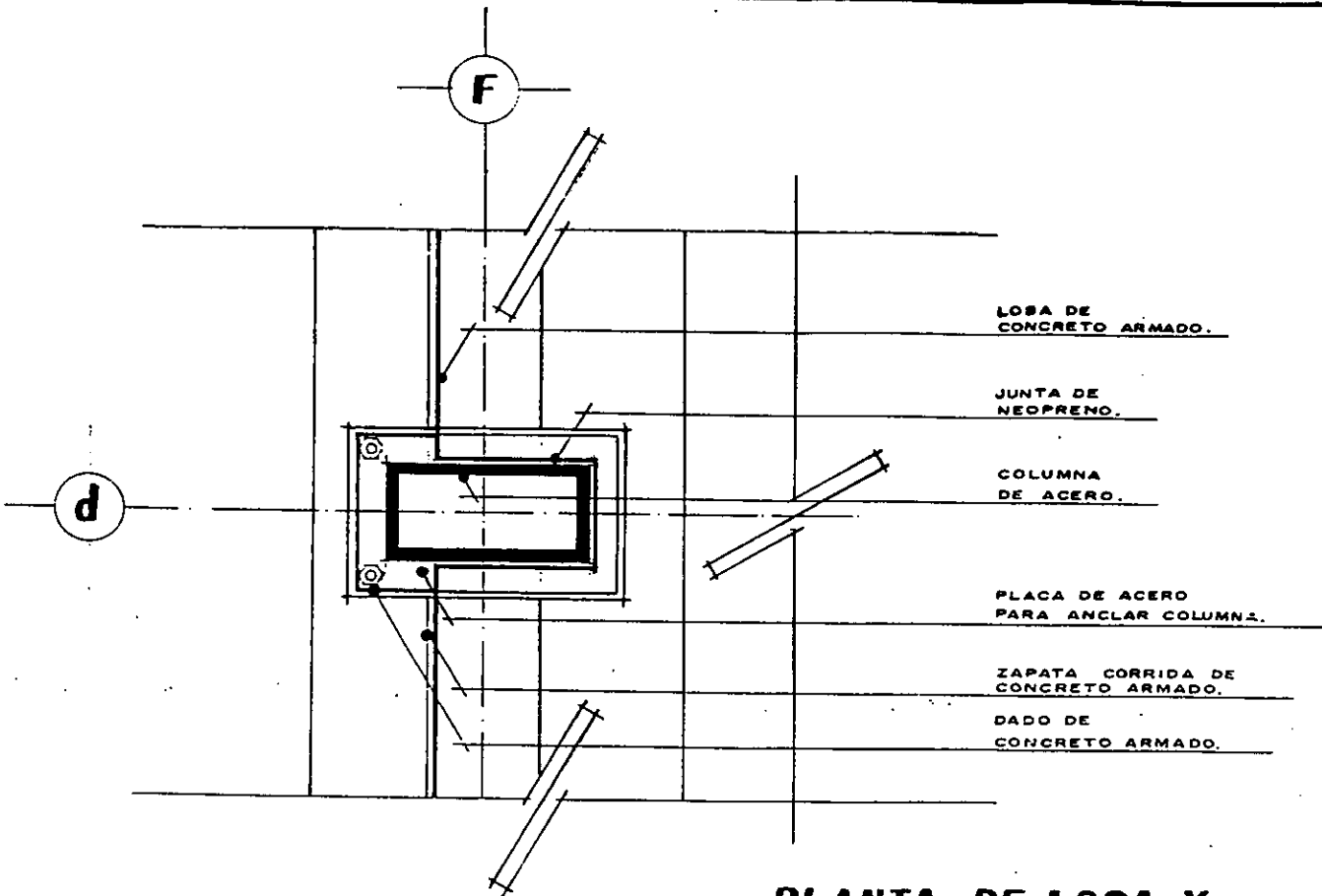
PLANTA DE LOSA Y COLUMNA. Esc. 1:20
