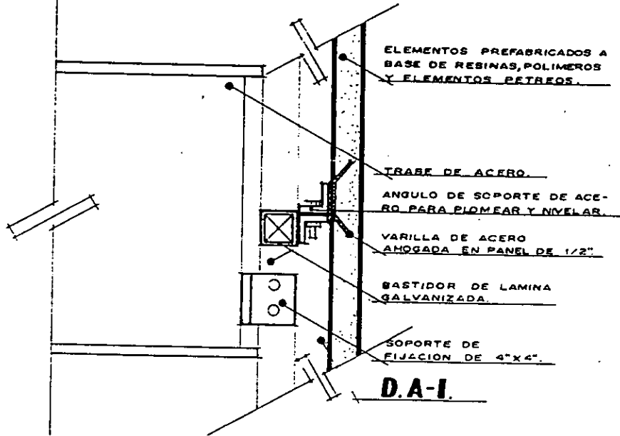
DETALLE DE FIJACION. D.A-I.
