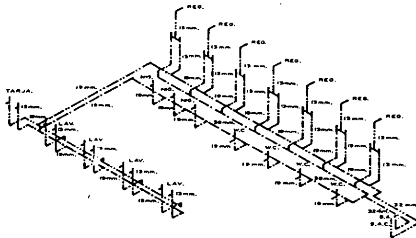
ISOMETRICO HIDRAULICO.
