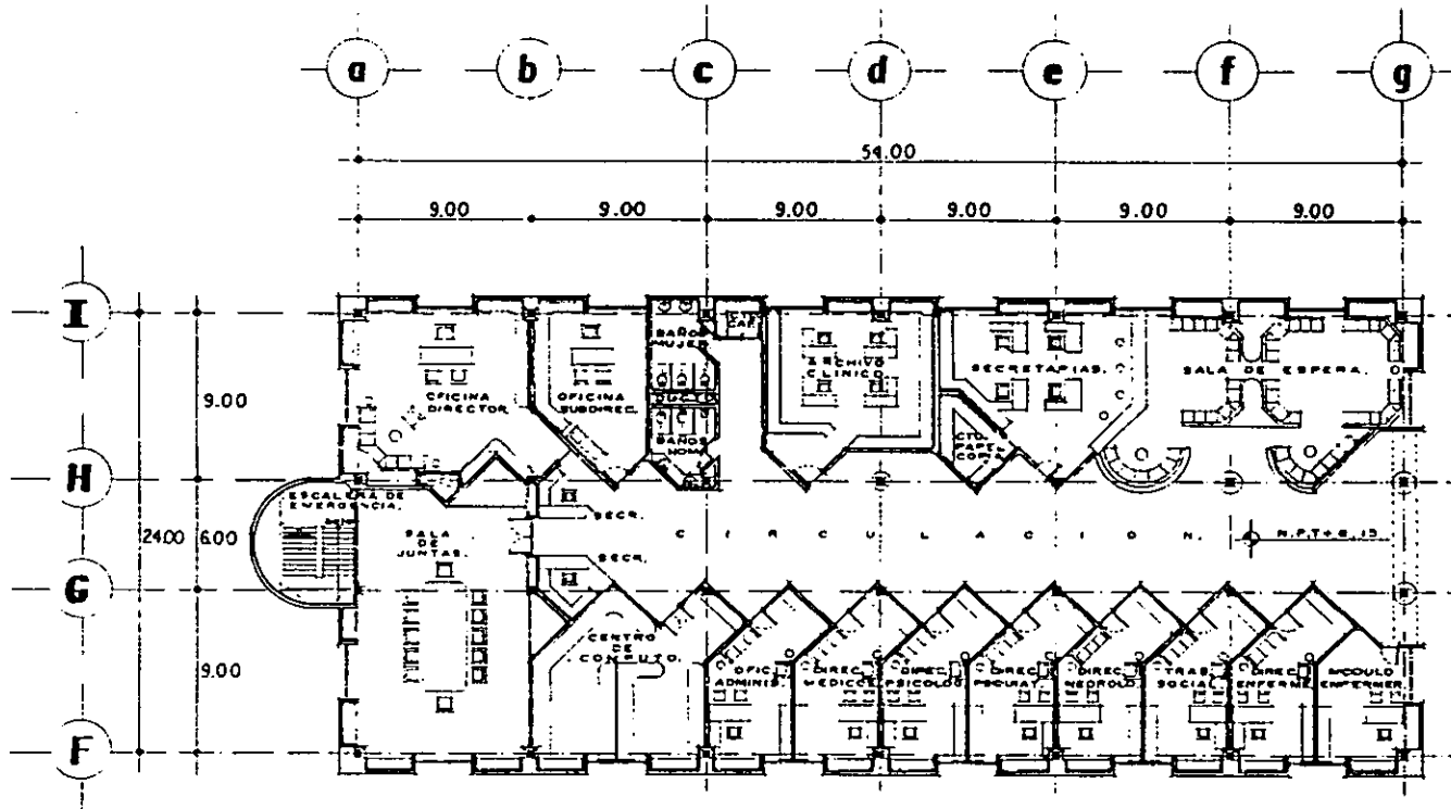
PLANTA DE ADMINISTRACION.
