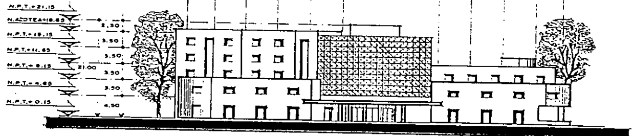
FACHADA SUR-ESTE.
