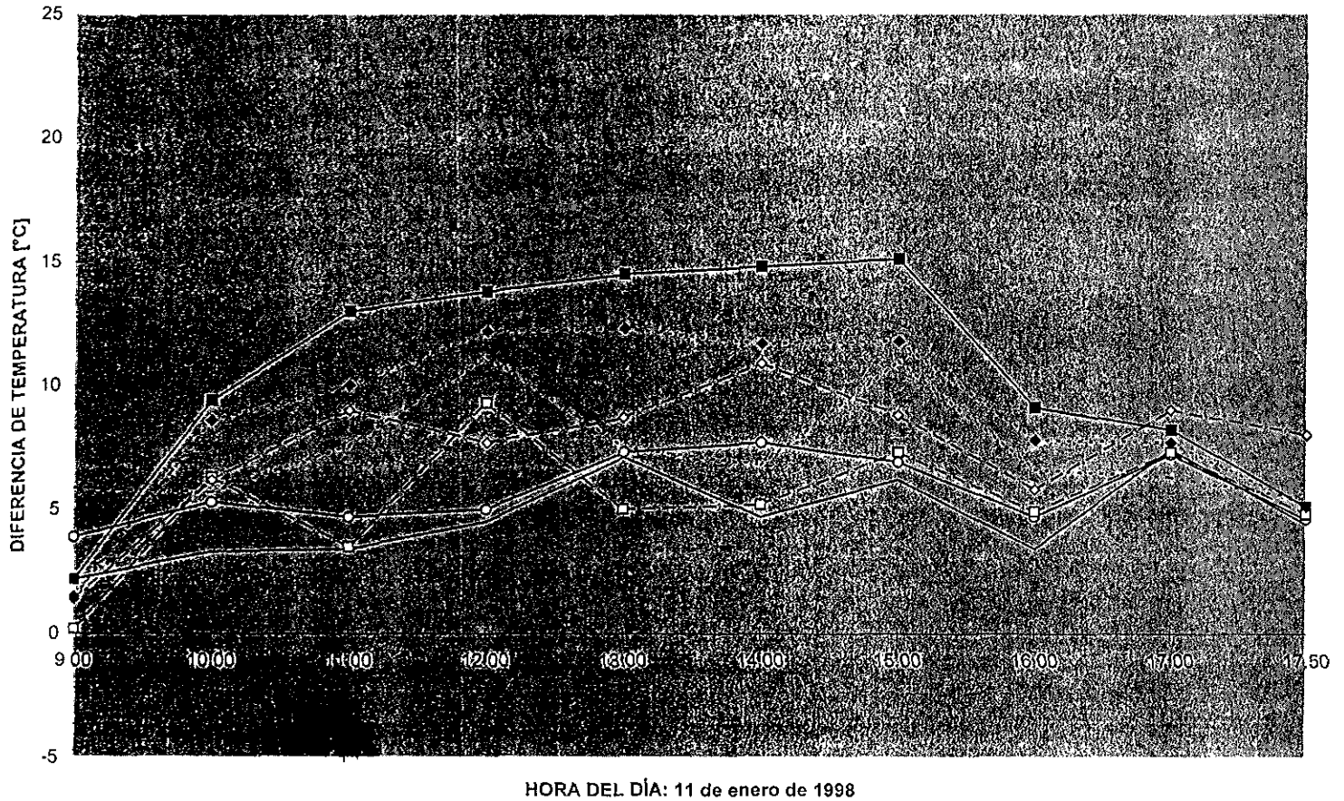
Figura 3.9. INVIERNO: Diferencia de temperatura entre la superficie exterior del techo y el ambiente exterior.
