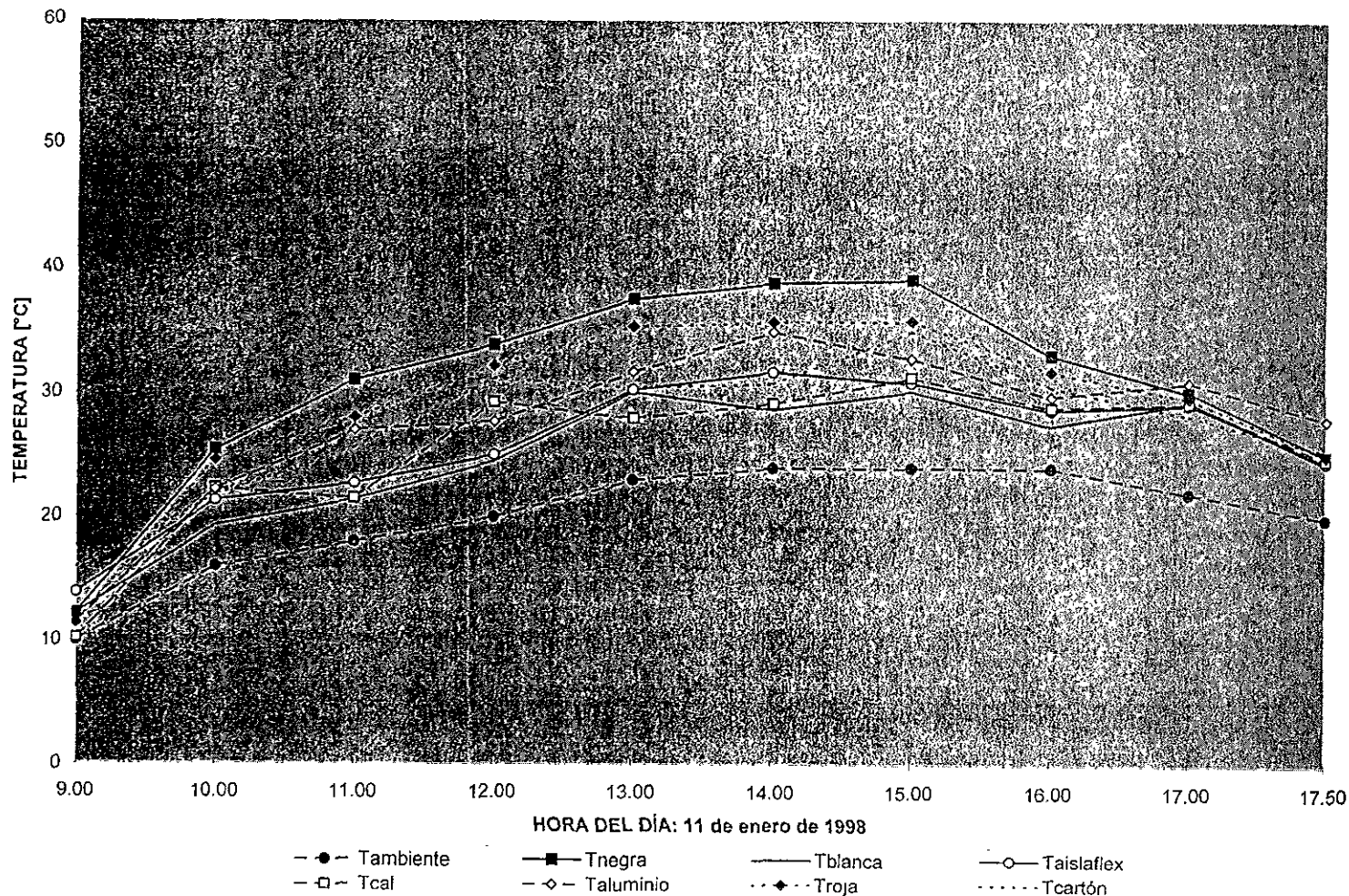
Figura 3.8. INVIERNO: Temperatura de la superficie exterior de los techos.
