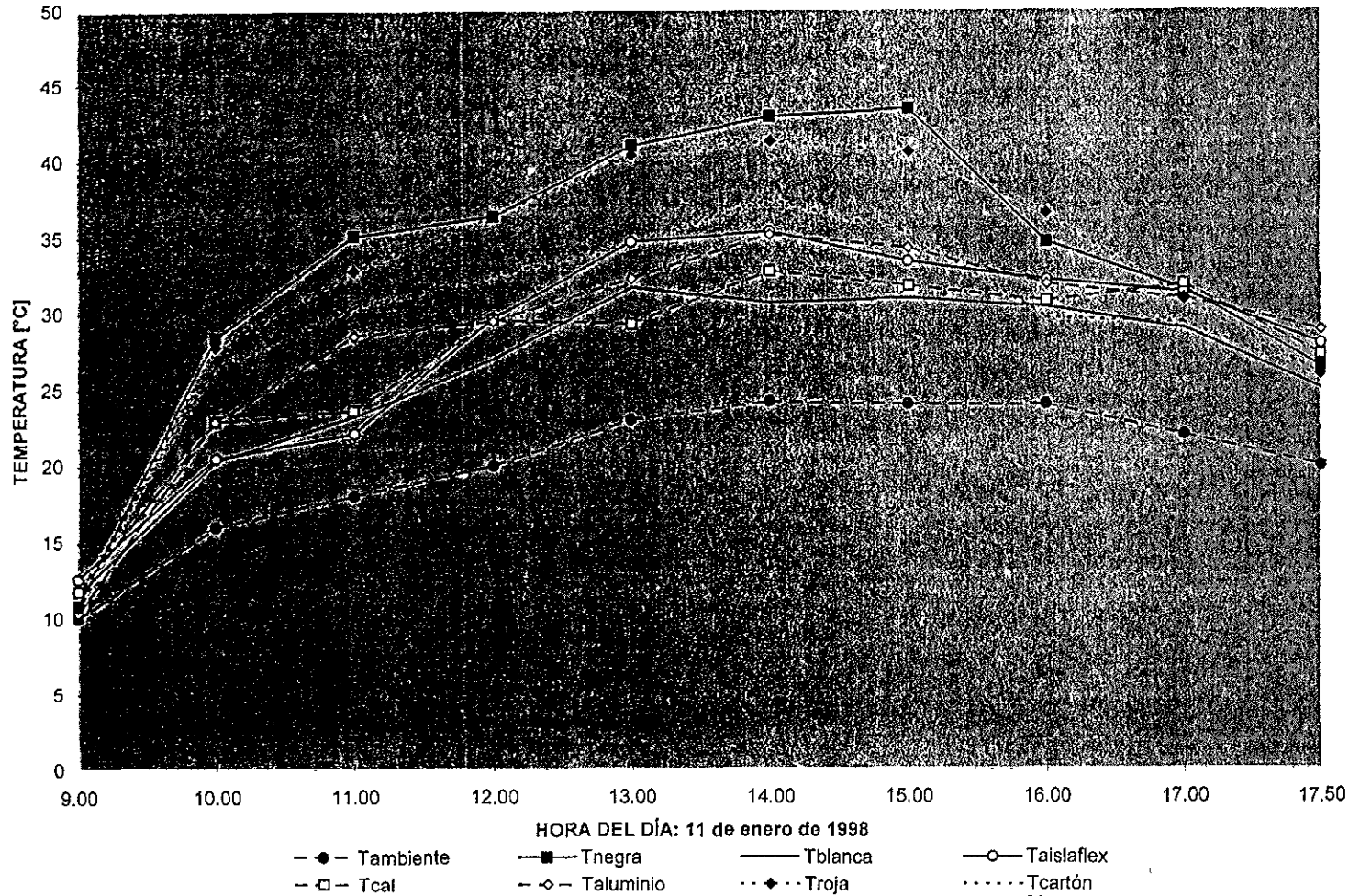
Figura 3.10. INVIERNO: Temperatura de interiores.
