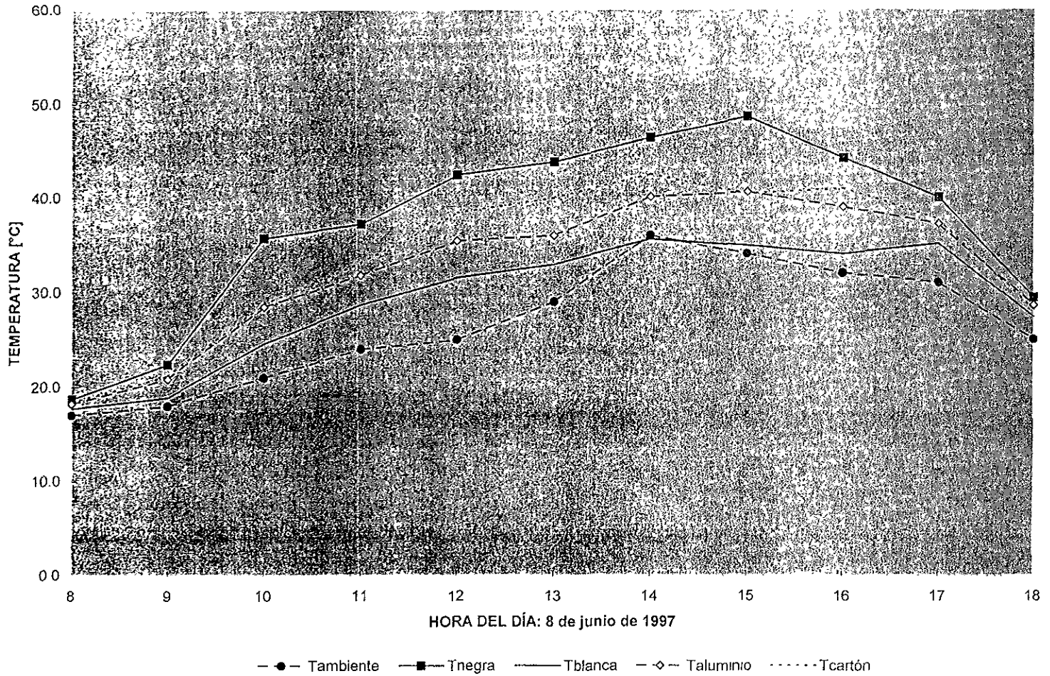
Figura 3.7. VERANO: Temperatura de interiores.
