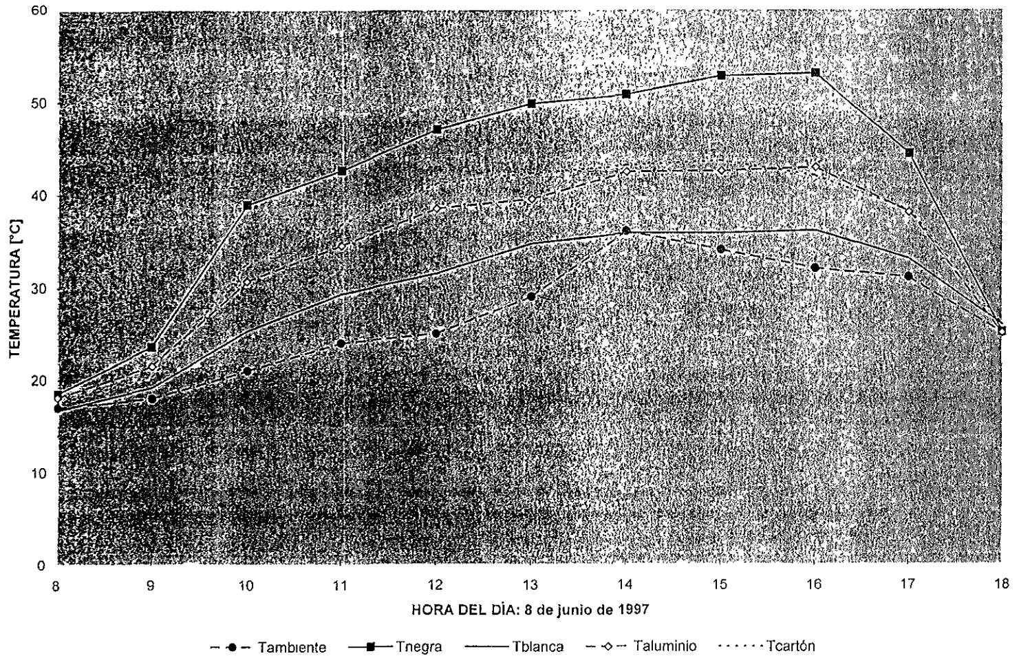
Figura 3.5. VERANO: Temperatura de la superficie exterior de los techos.
