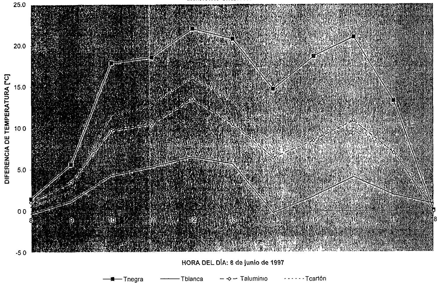
Figura 3.6. VERANO: Diferencia de temperatura entre la superficie exterior del techo y el ambiente exterior.
