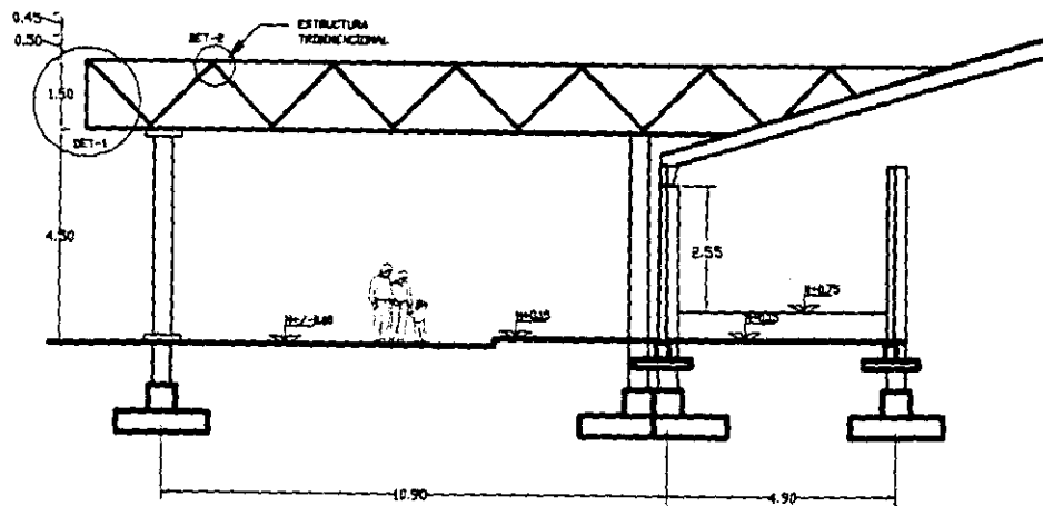
CORTE TRANSVERSAL
