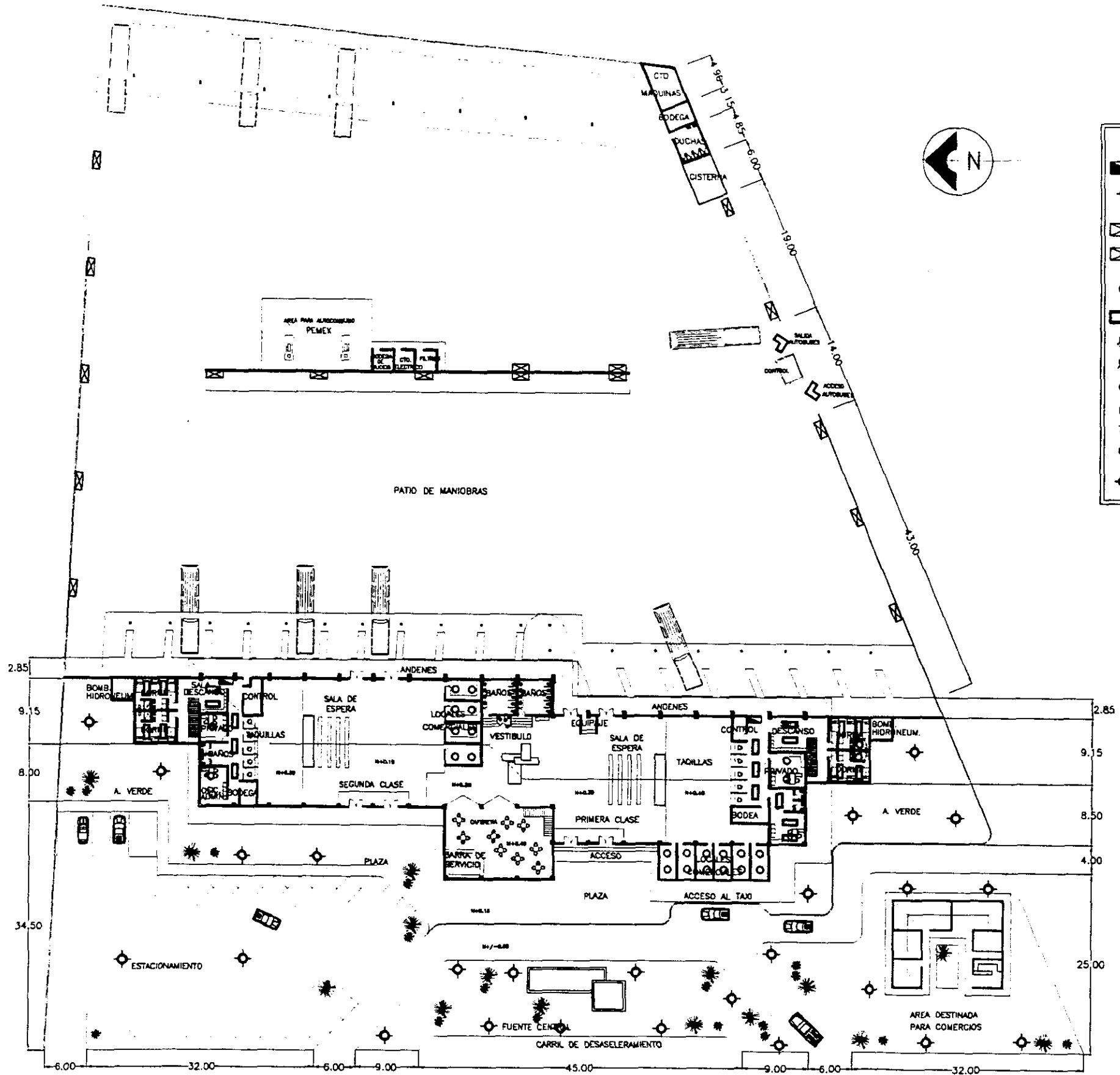
PLANTA ARQUITECTONICA
