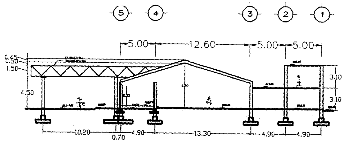
CORTE TRANSVERSAL
