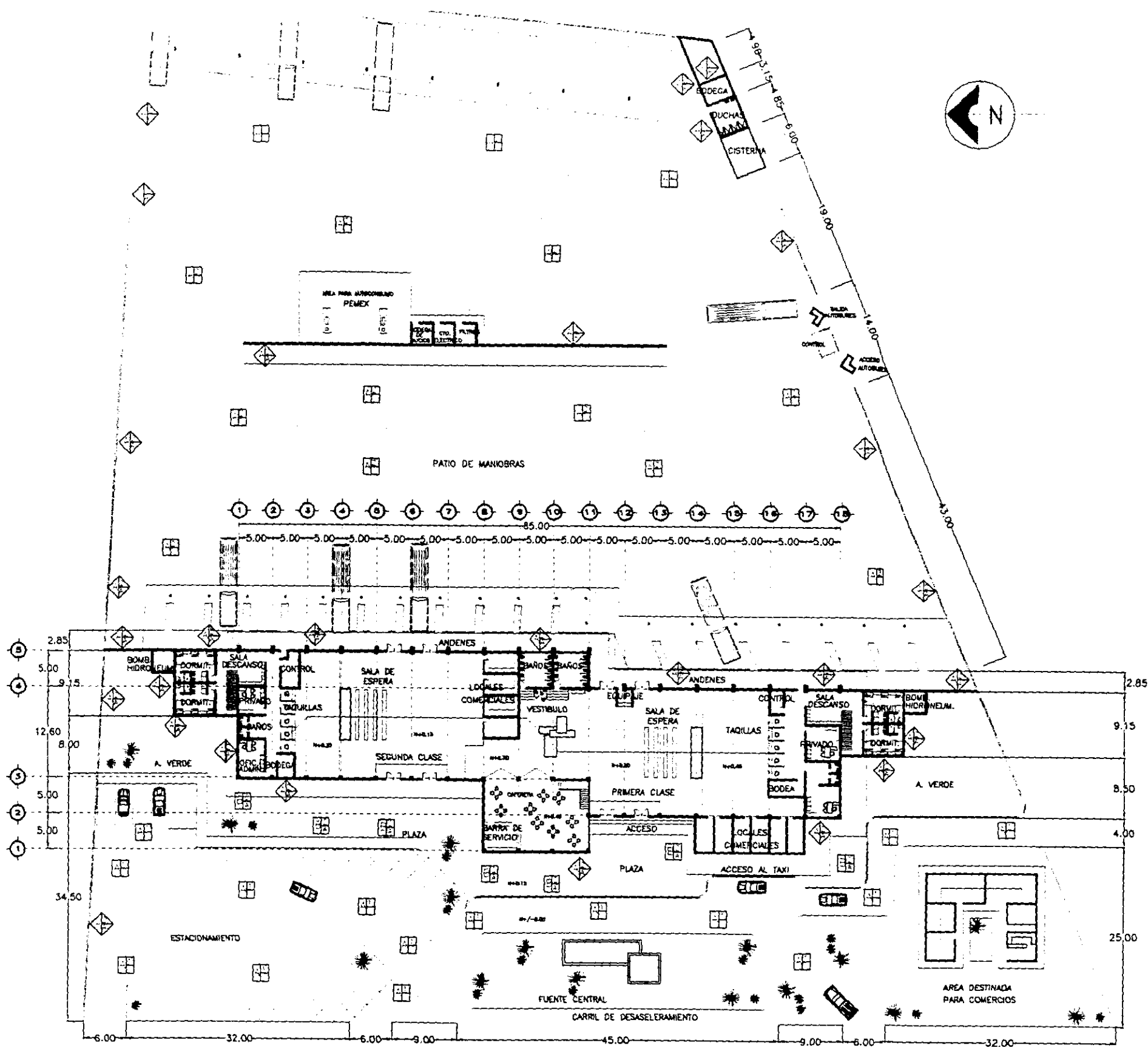
PLANTA ARQUITECTONICA
