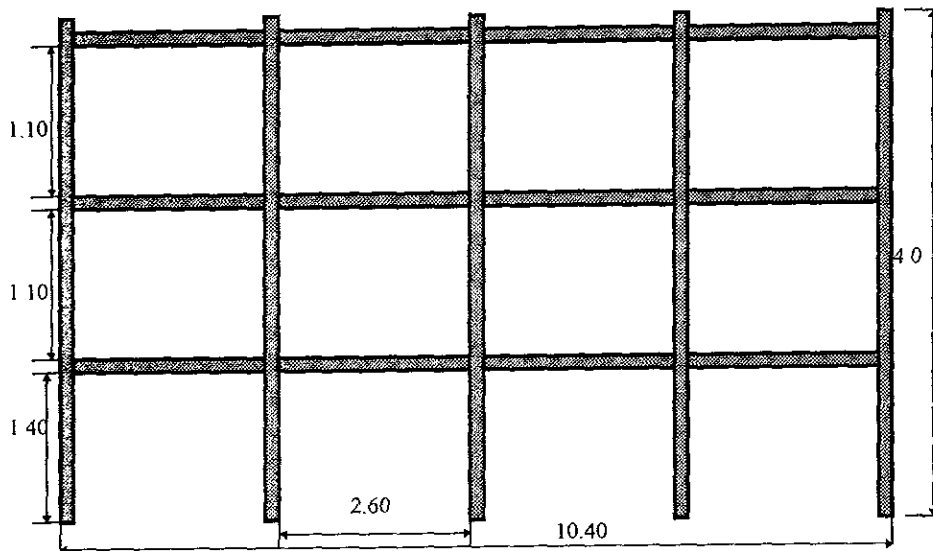
( Figura 3.3 A) RACK PARA PRODUCTO TERMINADO ( vista lateral, acotación m)
