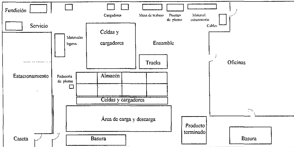
FIGURA 3.2 DISTRIBUCIÓN DE PLANTA
