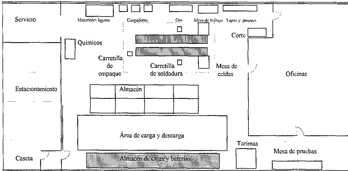
FIGURA 3.1 DISTRIBUCIÓN DE PLANTA MEJORADA
