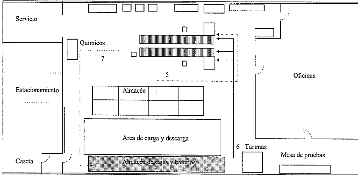
FIGURA 3 4 DIAGRAMA DE RECORRIDO MEJORADO
