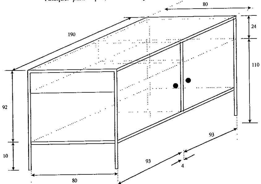
( Figura 3.14 ) Mesa de Trabajo (acotación cm)
