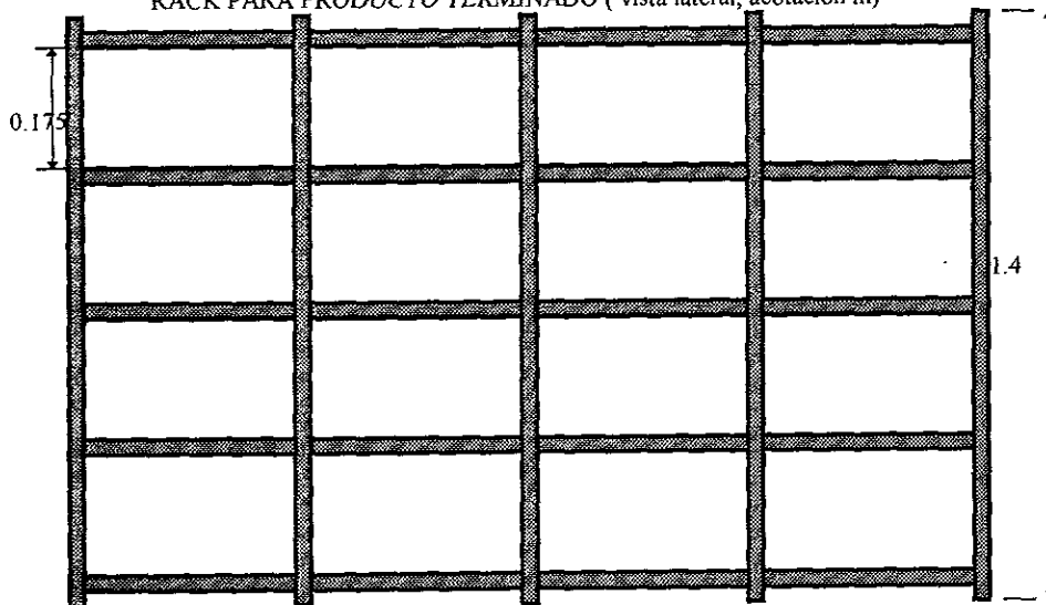
( Figura 3.3 B) RACK PARA PRODUCTO TERMINADO ( vista superior, acotación m)
