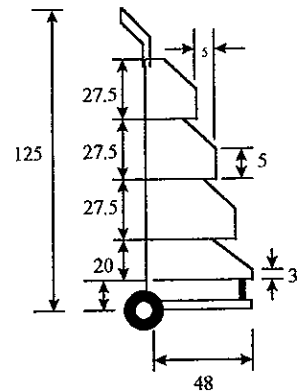
VISTA LATERAL
