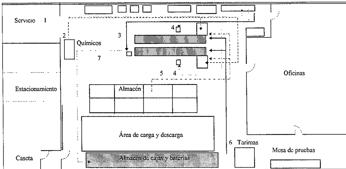
FIGURA 3.6 DIAGRAMA DE RECORRIDO MEJORADO
