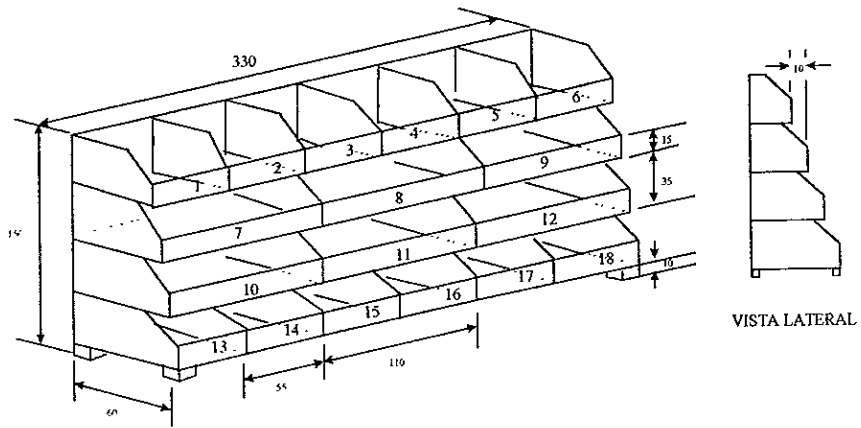
( Figura 3.13 ) Anaquel para Tapas, Conectores y Puentes (acotación cm)
