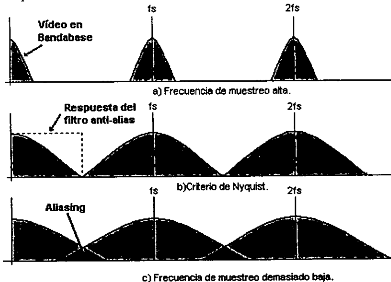
Fig. I-2.7 Límite de Nyquist sobre el espectro en frecuencia.
