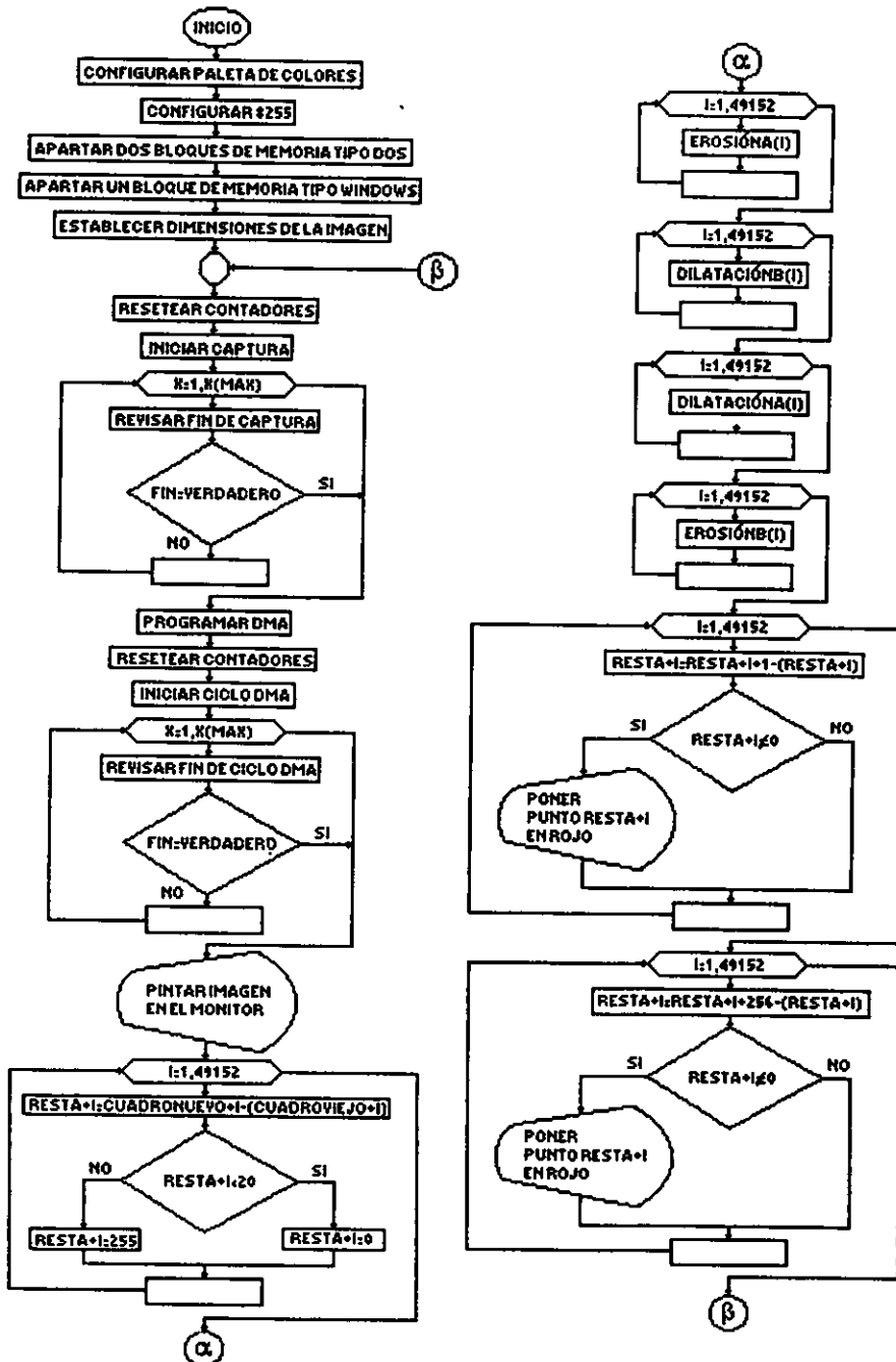
Fig. III-1.18. Diagrama de flujo del programa de contorno.
