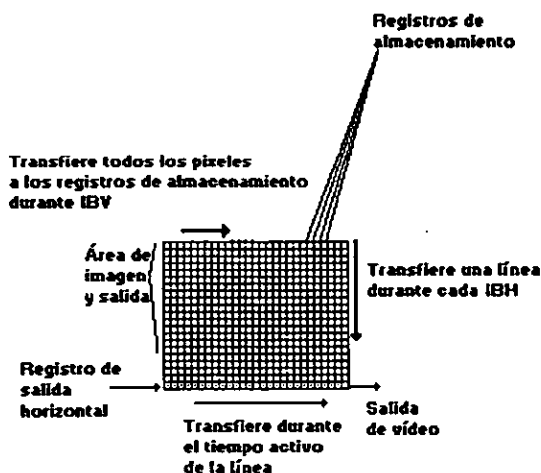
Fig. I-3.5 Arquitectura de Transferencia Interlínea.
