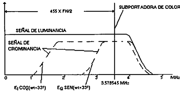
Fig. I-1.6 Espectro de la señal de vídeo compuesto.
