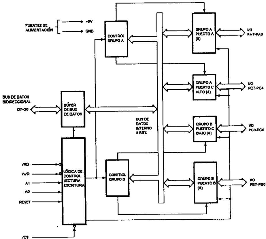
Fig. II-2.20. El 8255.
