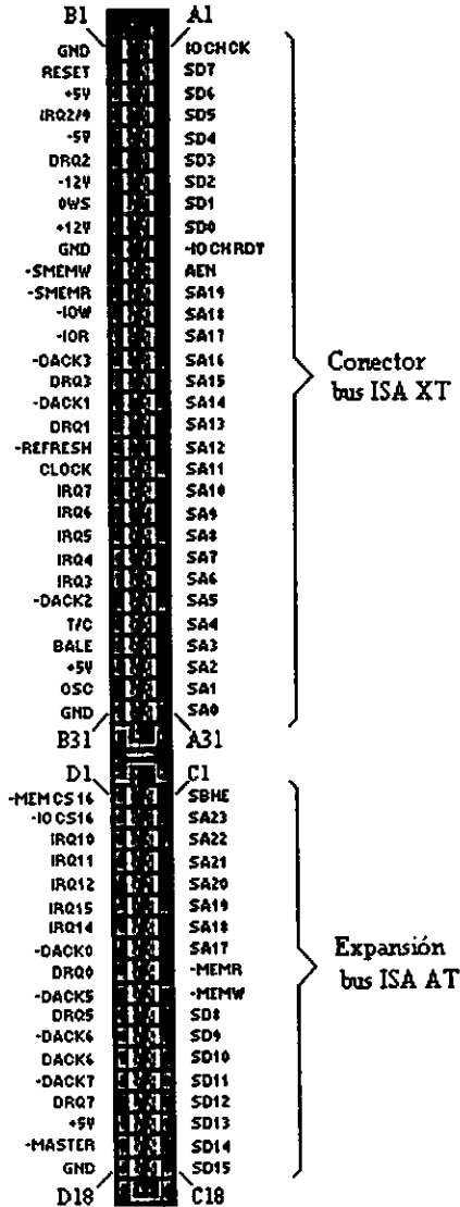
Fig. II-2.19. Conector ISA.
