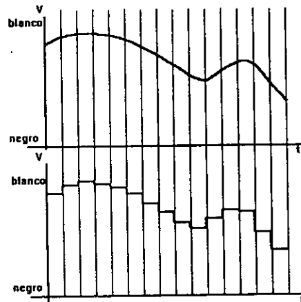
Fig. I-2.3 Conversión Analógica/Digital.
