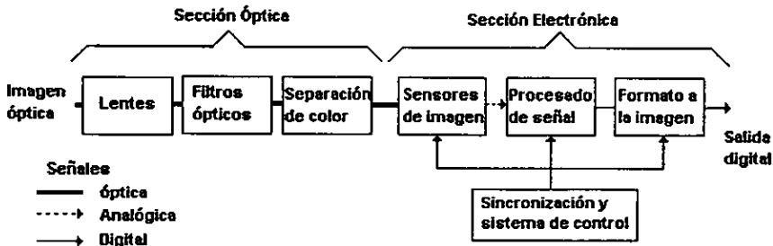
Fig. I-3.1 Diagrama de funcionamiento de una vídeo cámara.
