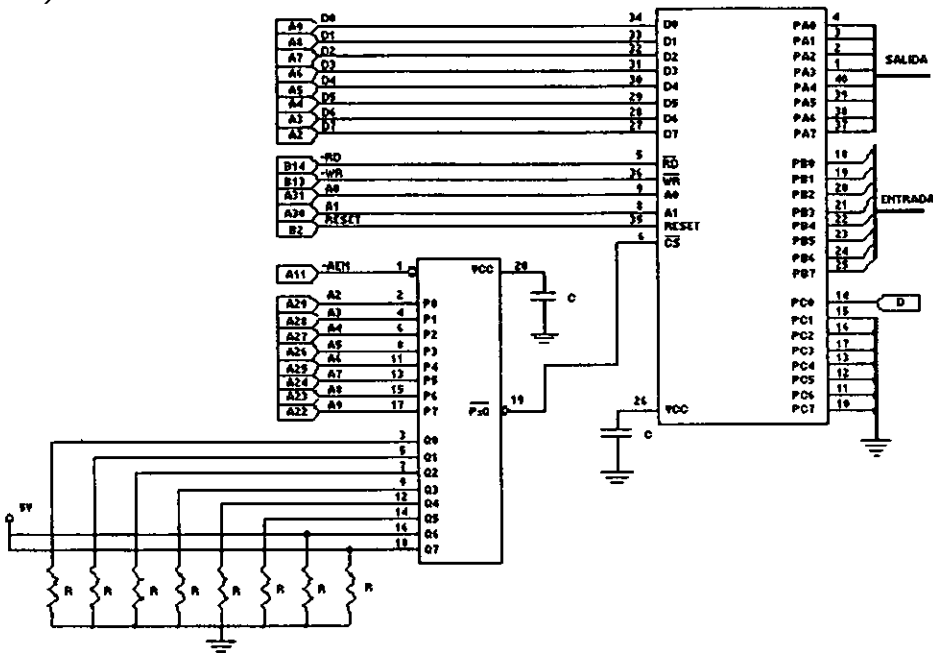
Fig. II-2.22. Implementación de la interface paralela.
