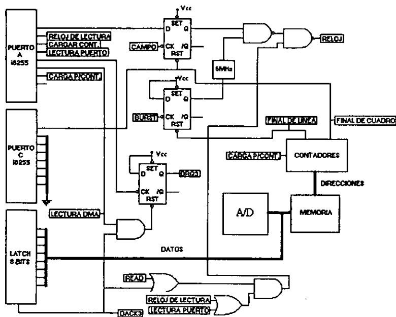
Fig. II-2.28. Sección DMA de la tarjeta.
