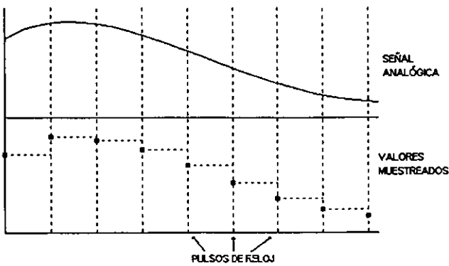
Fig. I-2.4 Muestreo.
