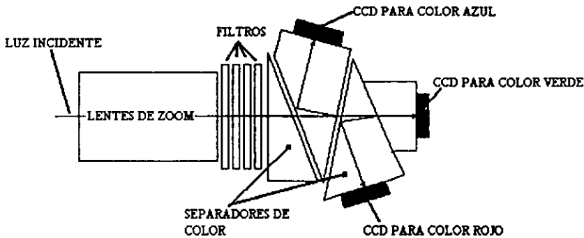
Fig. I-3.10 Sistema Óptico de las cámaras.
