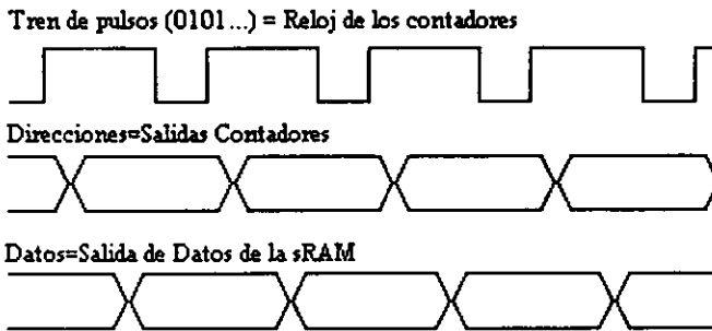
Fig. II-2.29 Diagrama de tiempos de adquisición mediante lectura a puertos.
