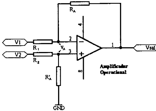
Fig. II-2.2 Amplificador de entrada diferencial.
