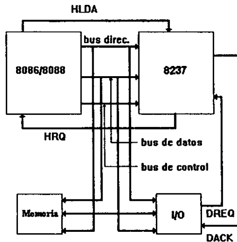
Fig. II-2.27 Diagrama de bloques básico de la interface DMA.
