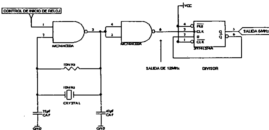
Fig. II-2.13. Reloj implementado.
