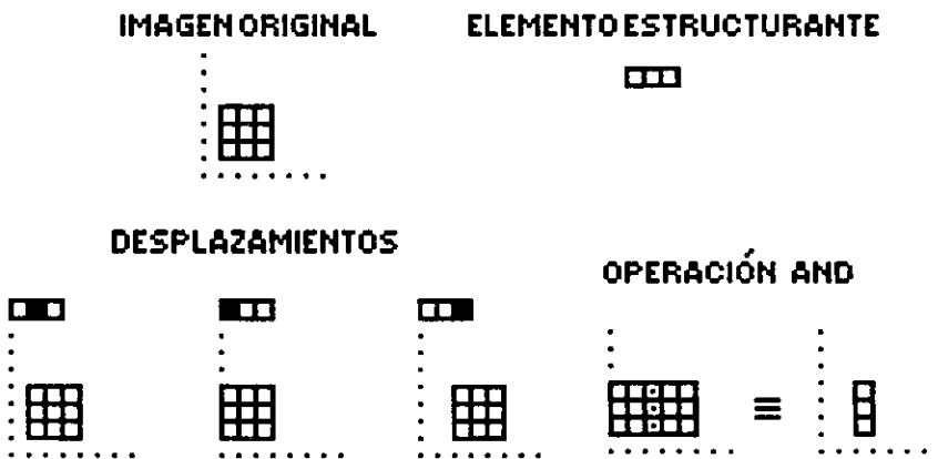
Fig. III-1.15 Erosión.
