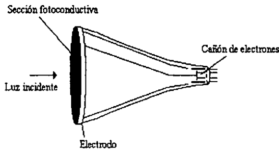
Fig. I-3.2 Construcción de un tubo fotoconductor.
