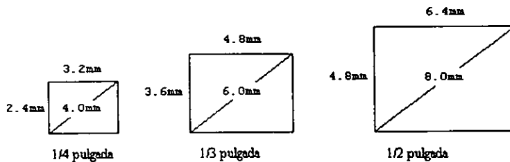
Fig. I-3.13 Formato CCD.
