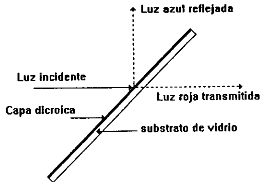
Fig 1-3.12 Operación de un filtro Dicroico.
