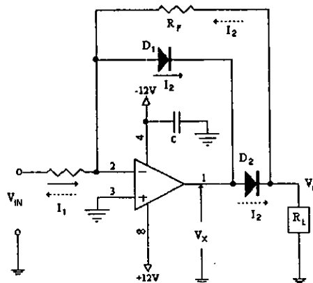
Fig. II-2.8 Rectificador de precisión de media onda.
