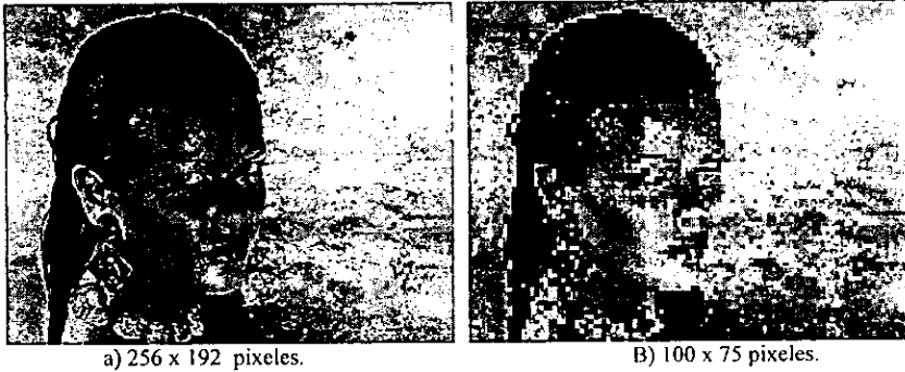
Fig. I-2.10 Pixelización.
