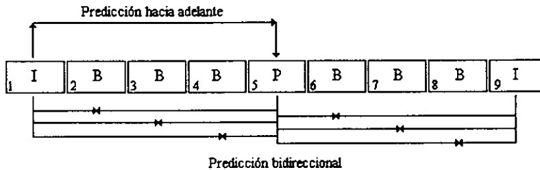
Fig. I-4.16 Predicción bidireccional.
