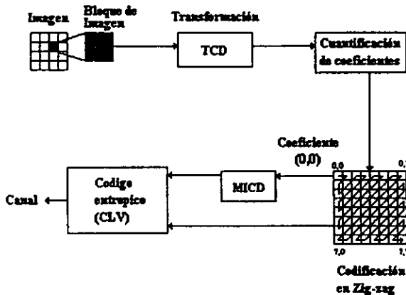
Fig. I-4.12 Codificación JPEG.
