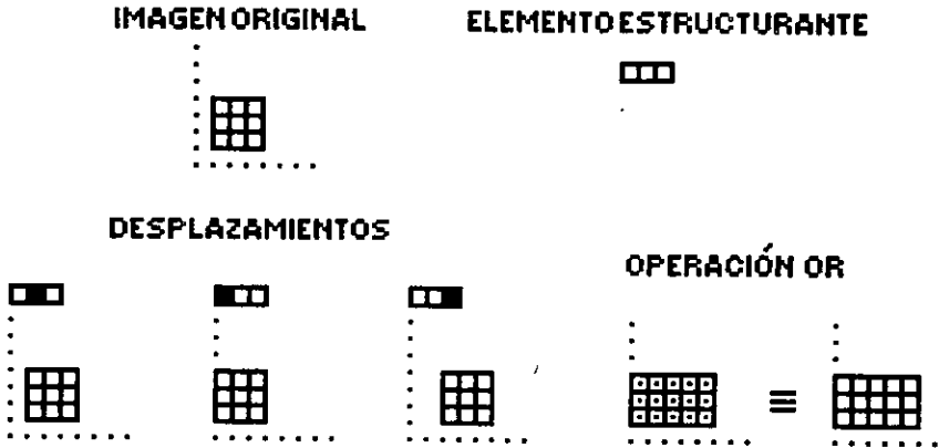
Fig. III-1.16 Dilatación.
