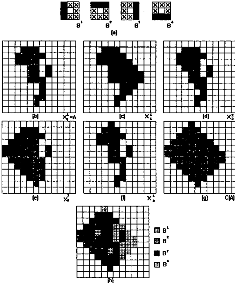
Fig. I-4.8 Corteza convexa.
