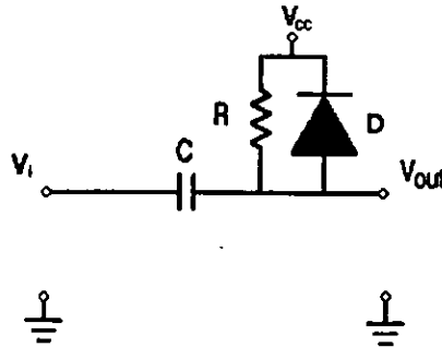
Fig. II-2.15. Circuito diferenciador.
