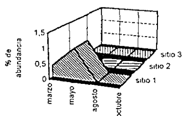
Gomphonema minutum
