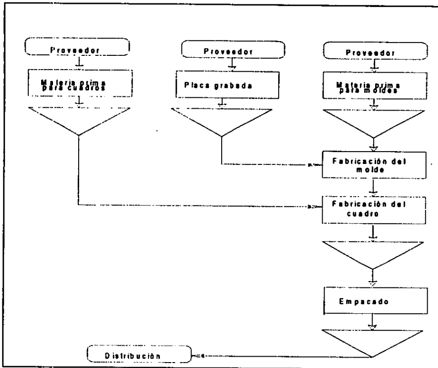
Figura 3: Diagrama de Flujo del Proceso en General
