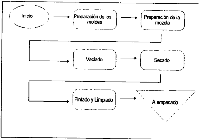
Figura 5: Flujo del Proceso de Fabricación de los Cuadros
