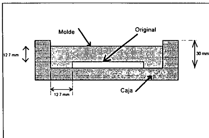
Figura 4: Montaje de la Caja para Moldear
