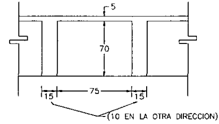
SECCION TRANSVERSAL
