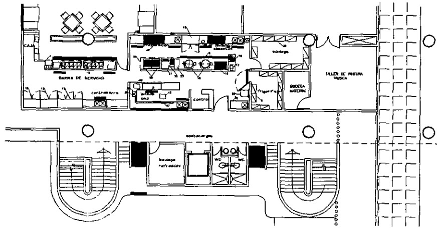
PLANTA BAJA
