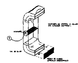
VISTA LATERAL DE DUCTO DE SALIDA DE UMA
