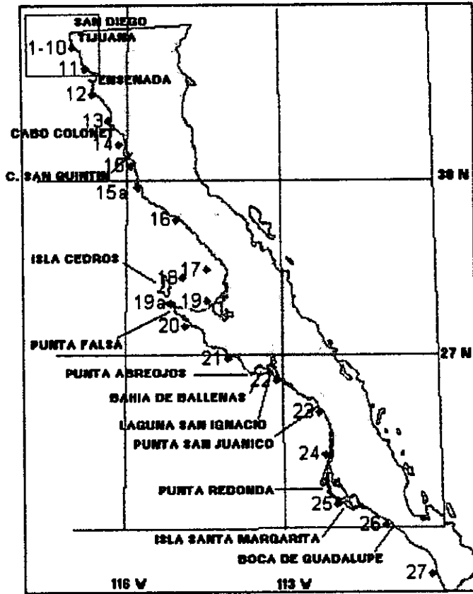
Mapa 1. Área de Estudio y Estaciones de Muestreo
