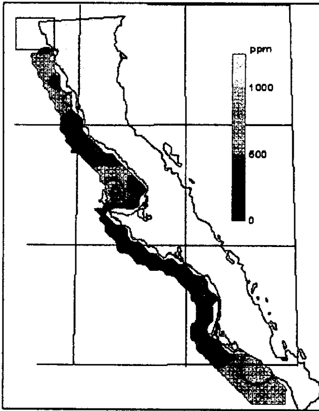
Mapa 12. Concentración de Hidrocarburos Totales en Sedimentos Primer Muestreo
