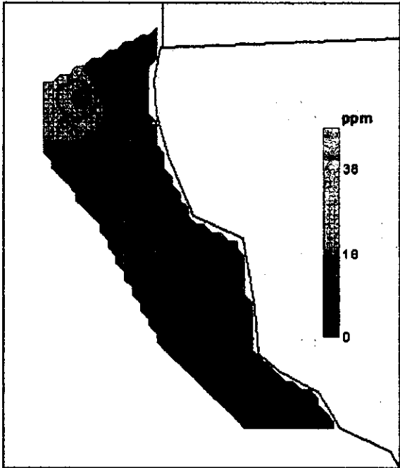
Mapa 9. Concentración de Hidrocarburos Aromáticos en Sedimentos Zona Norte Primer Muestreo
