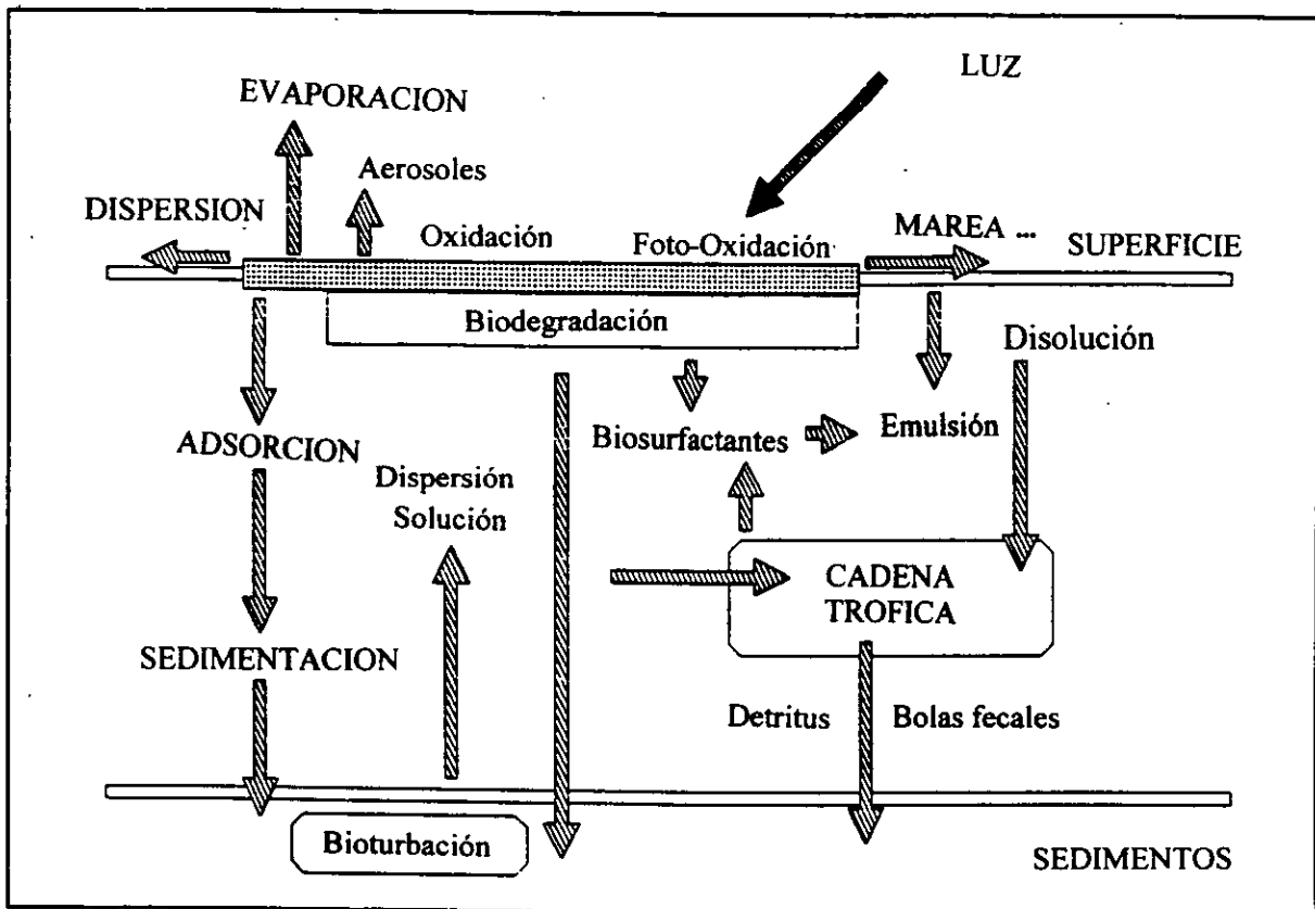
Figura 1. Procesos físico-químicos y biológicos que intervienen en la evolución de una mancha de petróleo en el medio marino. (Poulicek, 1994)
