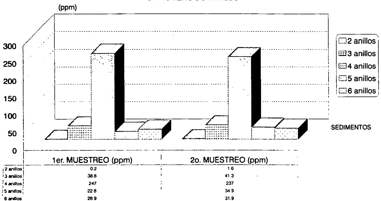
GRAF.10 HIDROCARBUROS AROMATICOS POLICICLICOS TOTALES POR NUMERO DE ANILLOS
