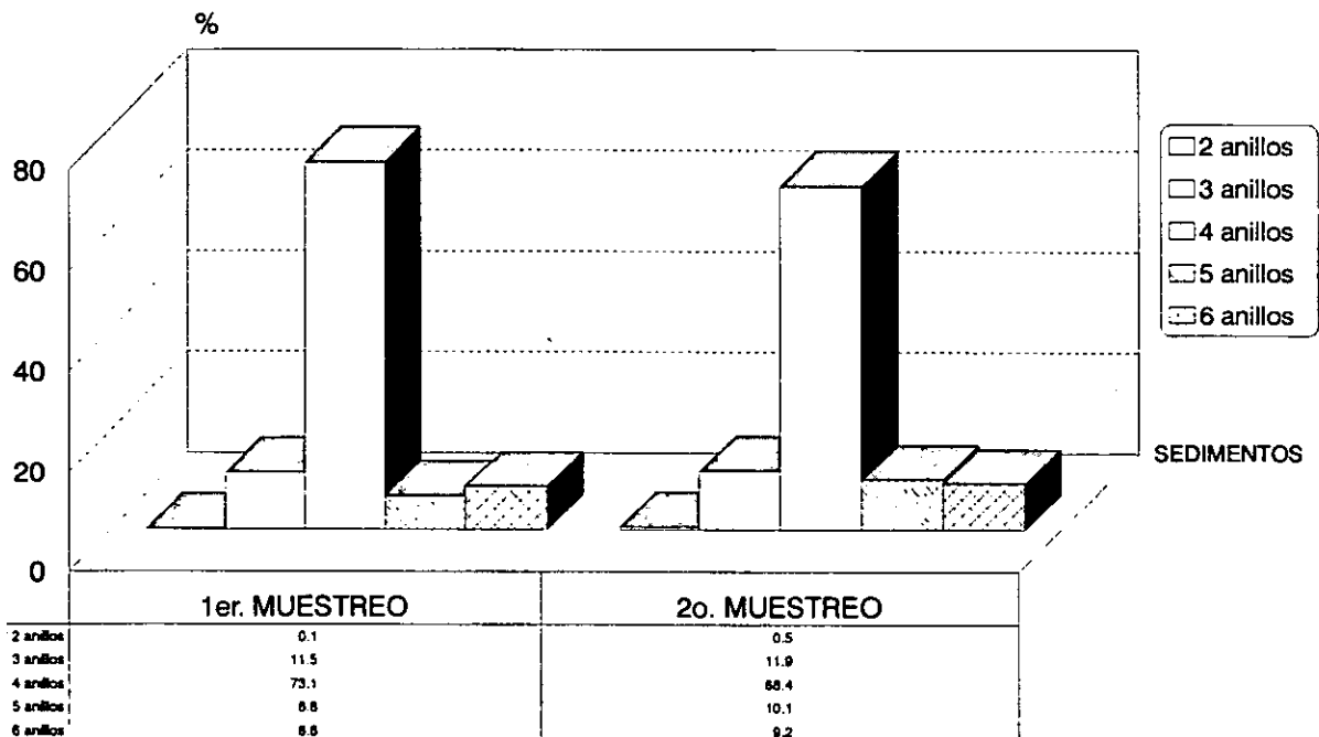
GRAF.11. % DE HIDROCARBUROS AROMATICOS POLICICLICOS TOTALES POR NUMERO DE ANILLOS
