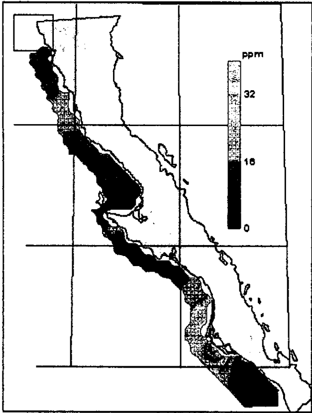
Mapa 8. Concentración de Hidrocarburos Aromáticos en Sedimentos Primer Muestreo
