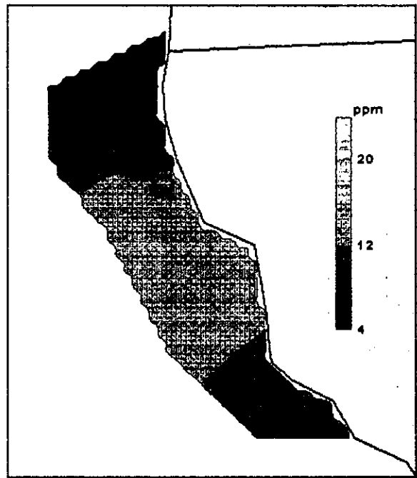
Mapa 11. Concentración de Hidrocarburos Aromáticos en Sedimento Zona Norte Segundo Muestreo
