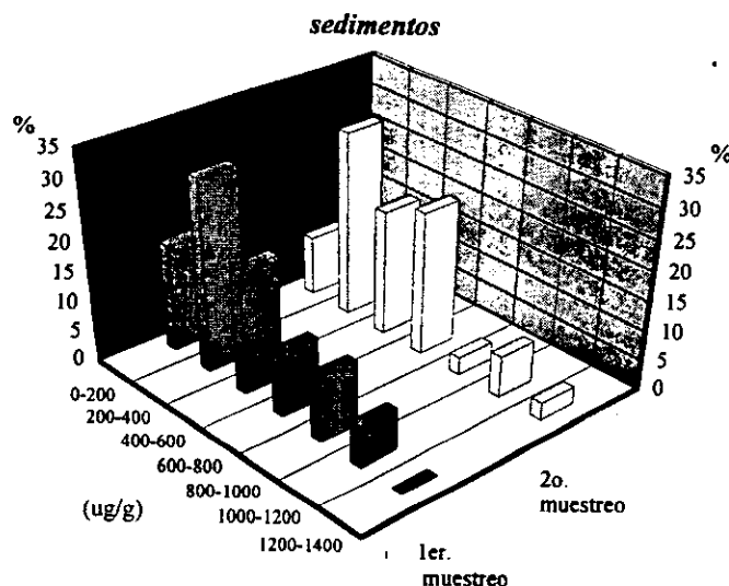
GRAF. 13. % DE HIDROCARBUROS TOTALES
