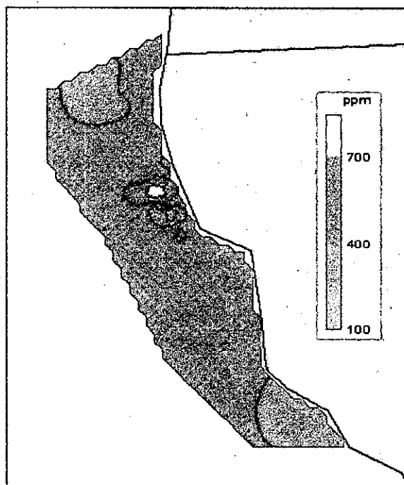
Mapa 15. Concentración de Hidrocarburos Totales en Sedimento Zona Norte Segundo Muestreo
