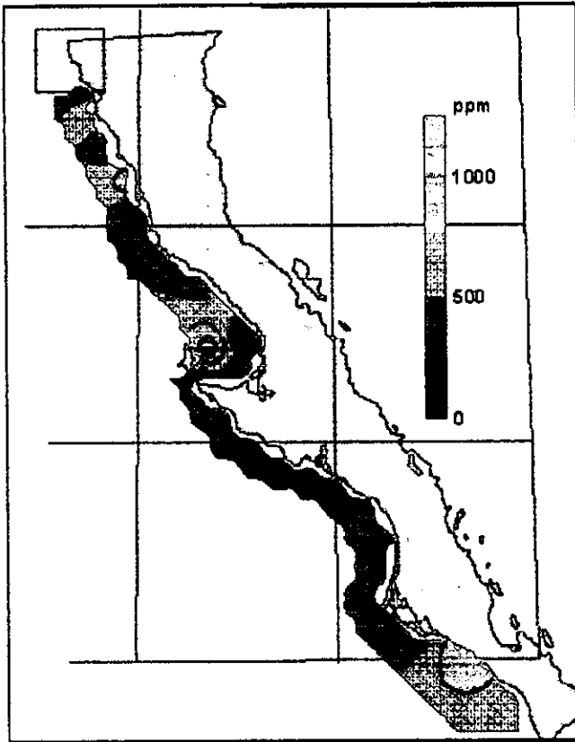
Mapa 4. Concentración de Hidrocarburos Alifáticos en Sedimentos Primer Muestreo
