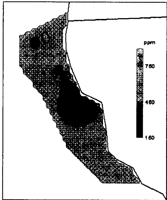
Mapa 13. Concentración de Hidrocarburos Totales en Sedimentos Zona Norte Primer Muestreo
