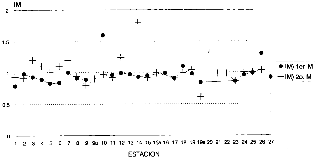
GRAF.6 INDICE DE MADUREZ 1er. Y 2o. MUESTREO
