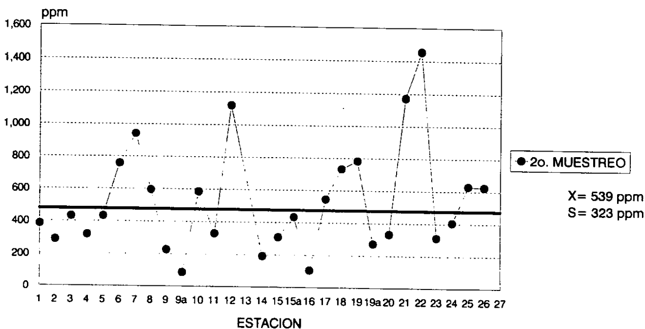
GRAF.2 NIVELES DE HIDROCARBUROS ALIFATICOS TOTALES EN SEDIMENTOS
