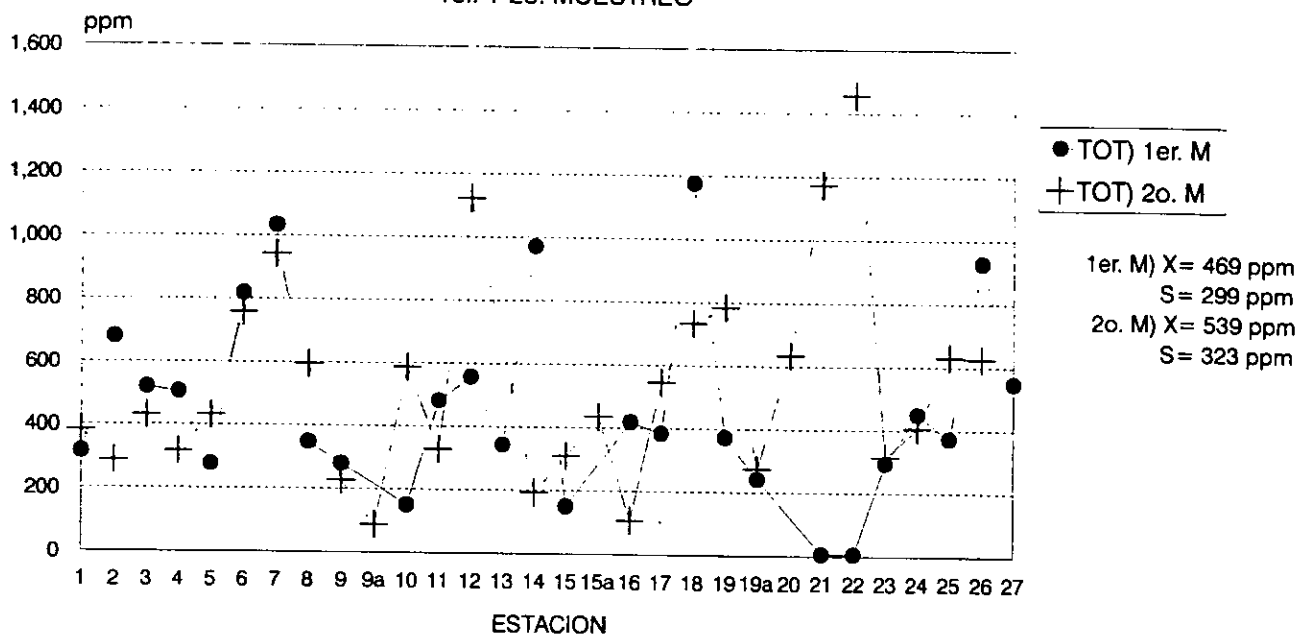
GRAF.8 HIDROCARBUROS ALIFATICOS TOTALES EN SEDIMENTOS 1er. Y 2o. MUESTREO
