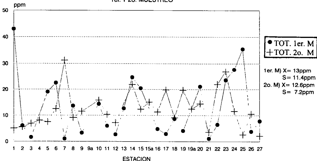
GRAF.9 HIDROCARBUROS AROMATICOS POLICICLICOS 1er. Y 2o. MUESTREO
