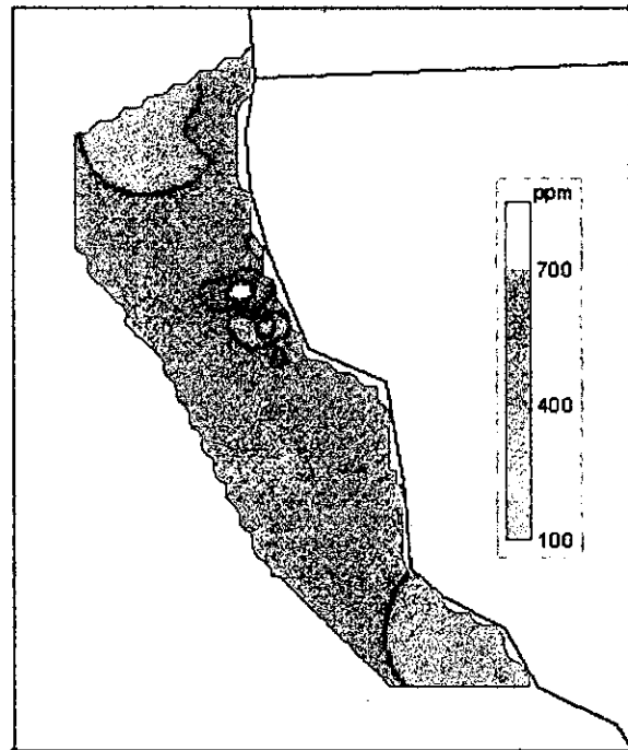
Mapa 7. Concentración de Hidrocarburos Alifáticos en Sedimento Zona Norte Segundo Muestreo
