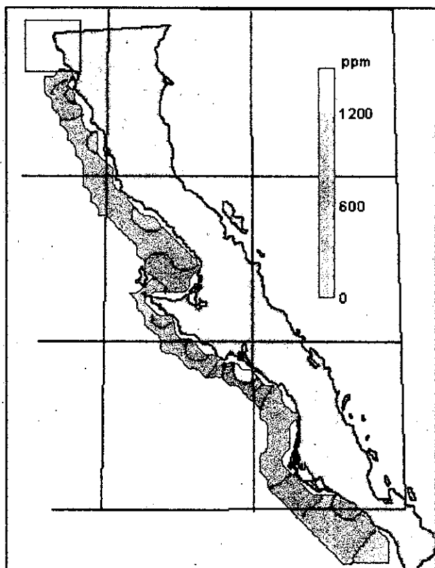
Mapa 14. Concentración de Hidrocarburos Totales en Sedimentos Segundo Muestreo
