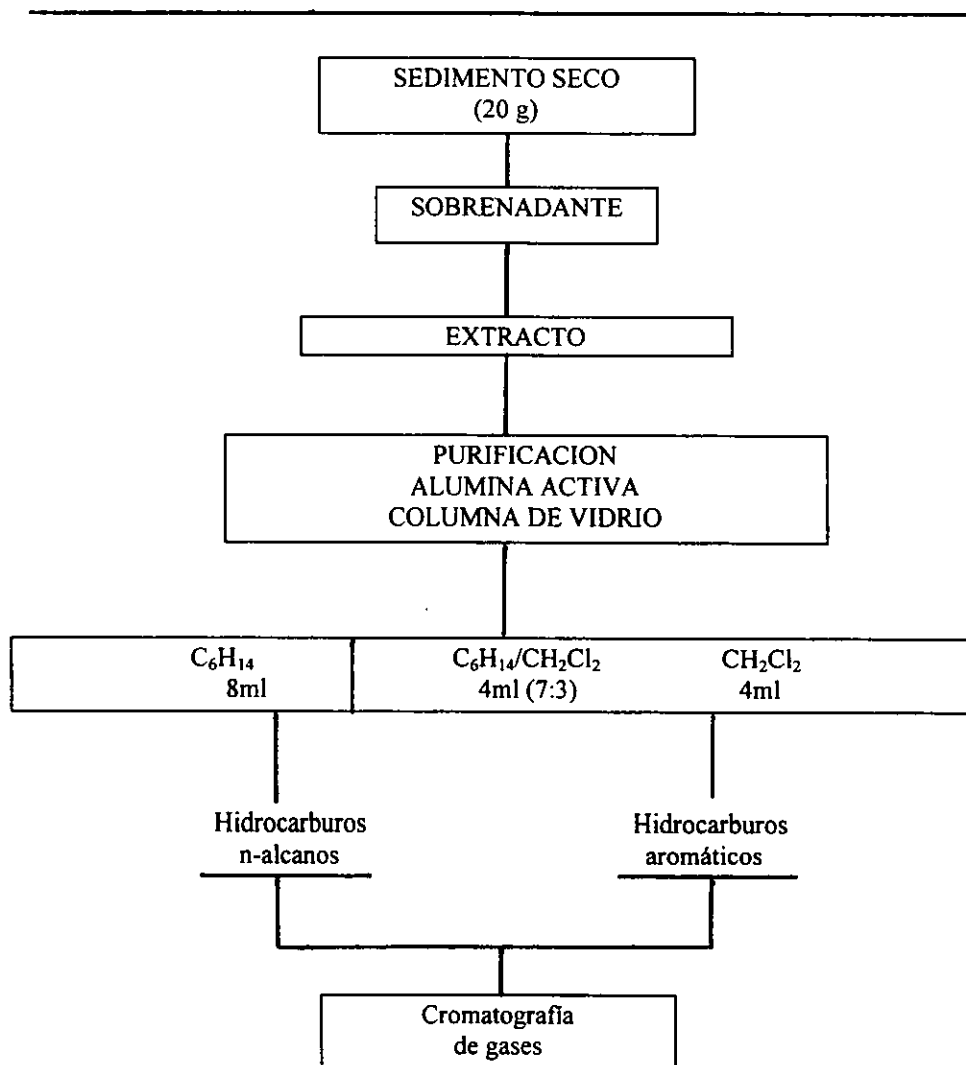
Cuadro No.3. Método para el análisis de hidrocarburos (CARIPOL - Iocaribe, 1986).
