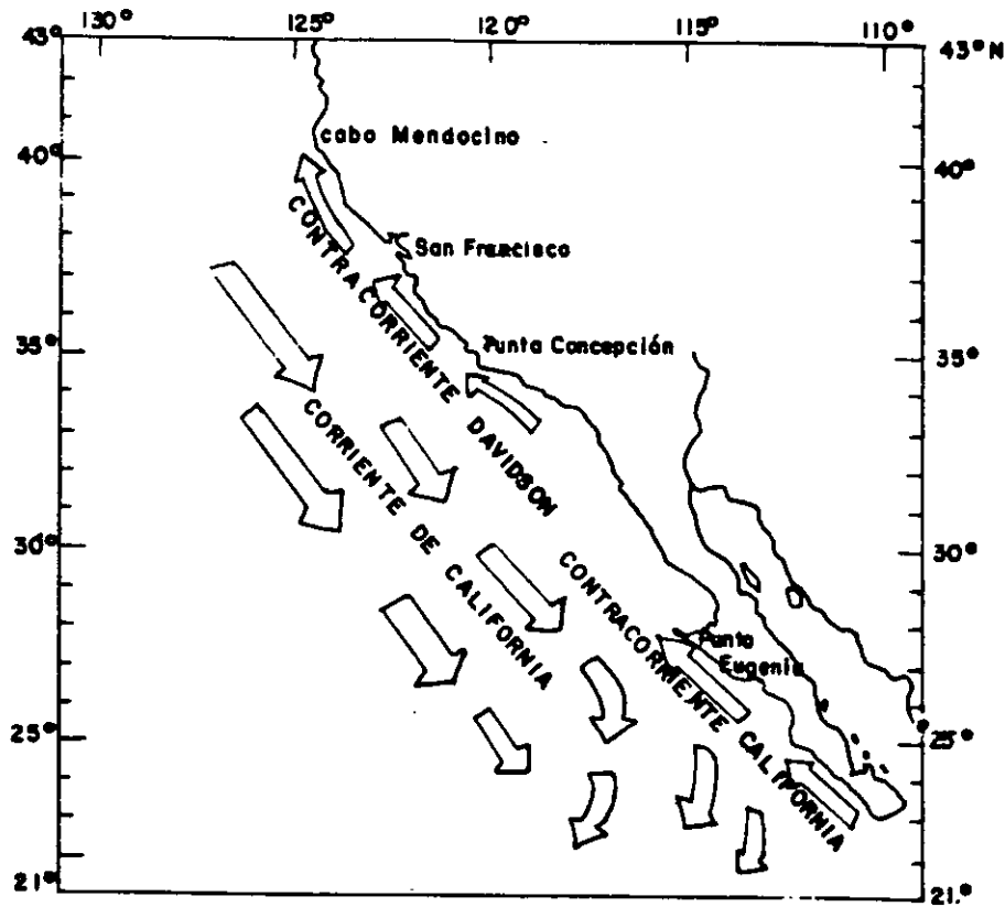
Figura 2. Corriente de California (Lanza , E.G. de la., 1991)
