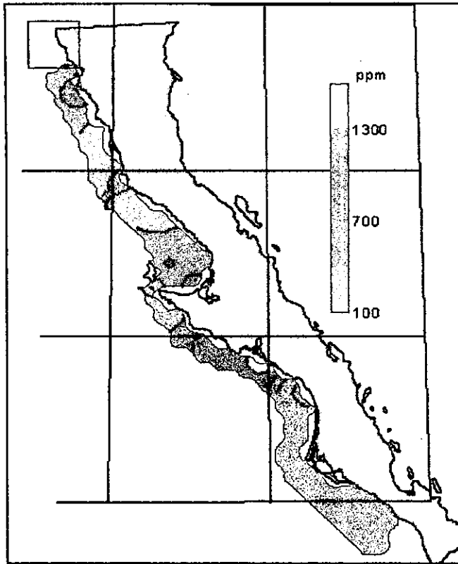
Mapa 6. Concentración de Hidrocarburos Alifáticos en Sedimentos Segundo Muestreo
