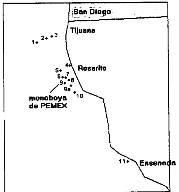
Mapa 2. Localización Estaciones Zona Norte
