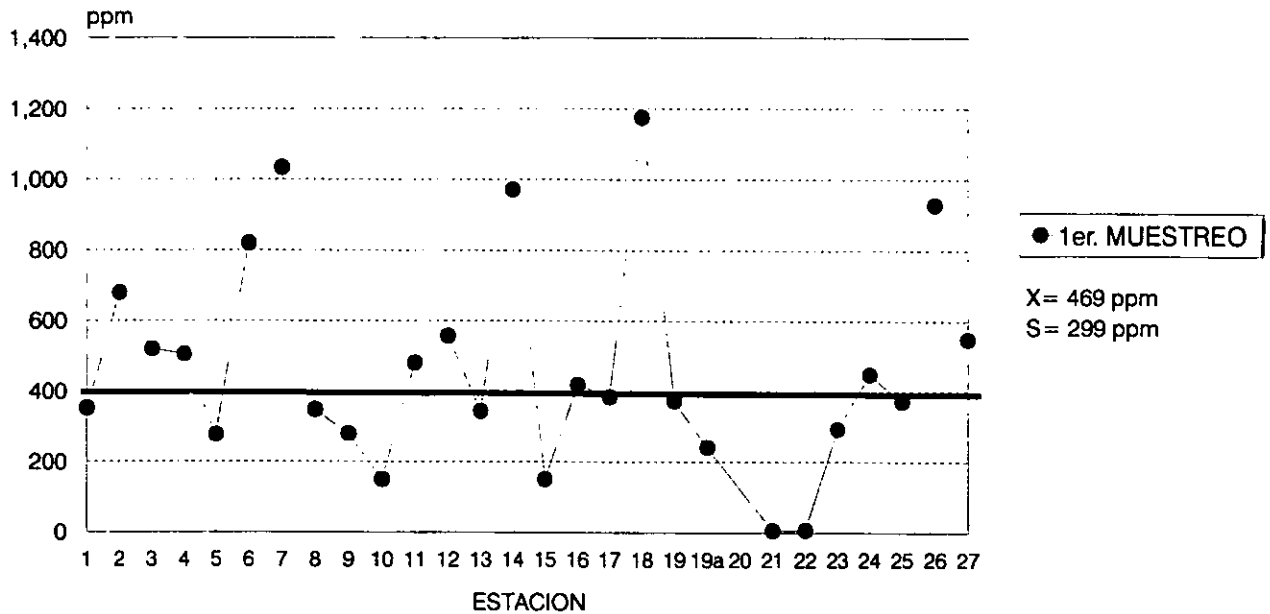
GRAF.1 NIVELES DE HIDROCARBUROS ALIFATICOS TOTALES EN SEDIMENTOS
