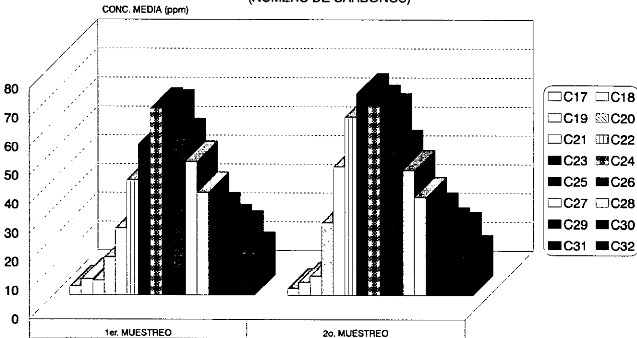
GRAF.7 HIDROCARBUROS ALIFATICOS (NUMERO DE CARBONOS)
