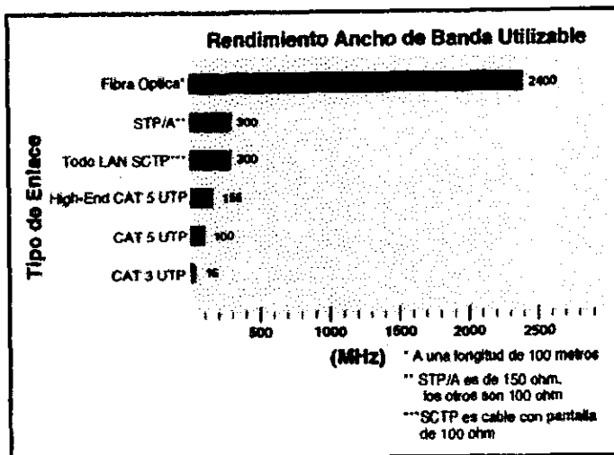
Fig. 3.5 Rendimiento de Ancho de banda Utilizable
