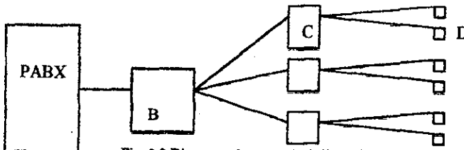
Fig. 3.2 Diagrama de una red telefónica interna
