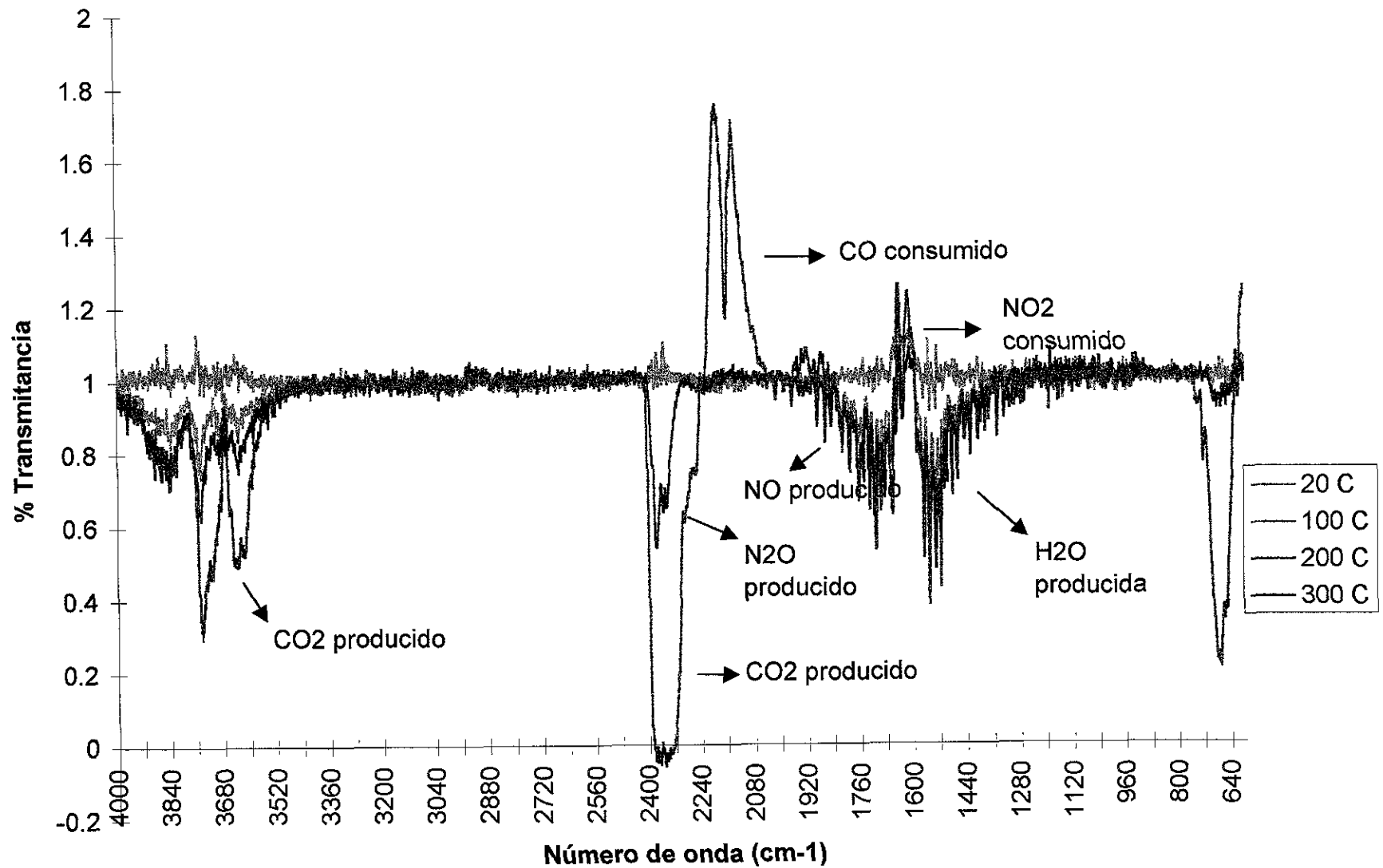
Fig. 20 Catalizador RuPt 300 (Temperatura ascendente)
