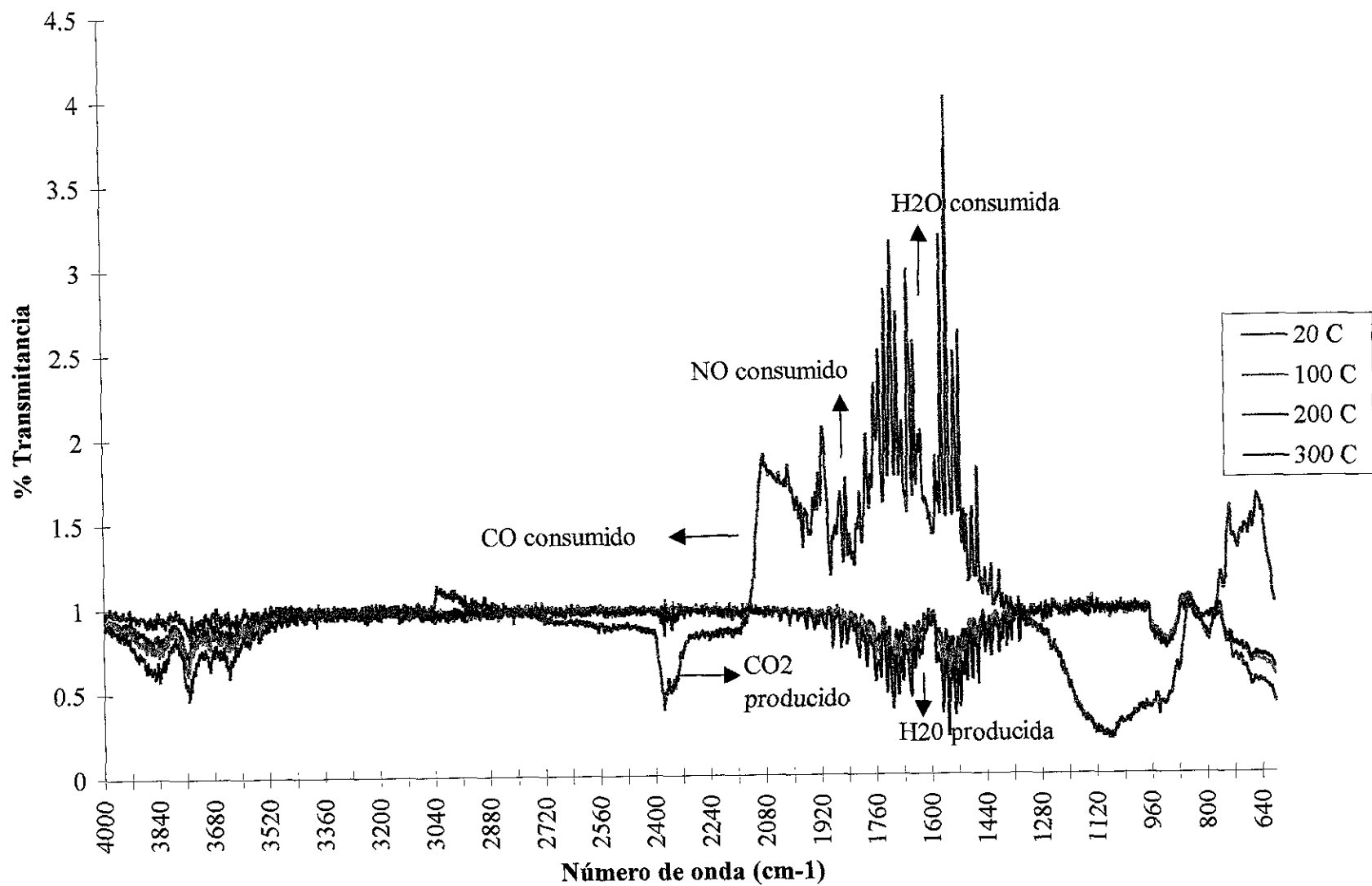
Fig. 24 Catalizador RU-300 (Temperatura ascendente)
