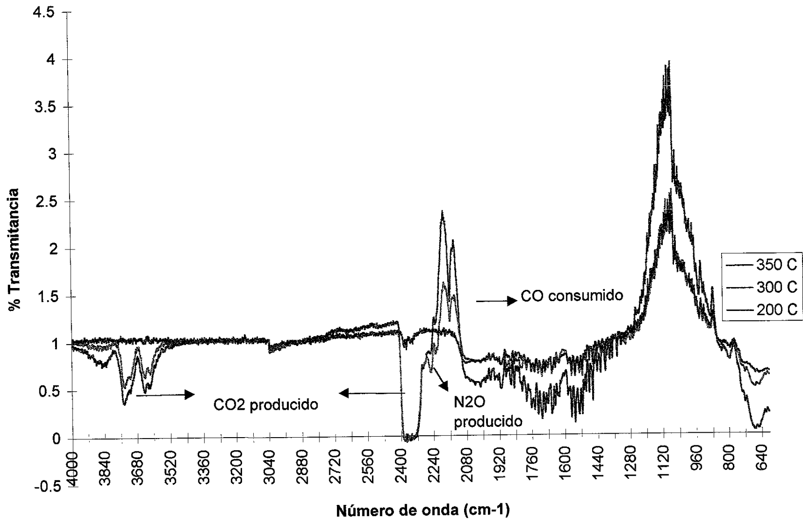
Fig. 20 Catalizador RUPt 350 (Temperatura ascendente)
