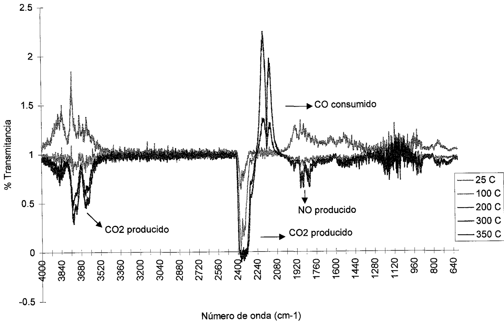
Fig. 18 Catalizador HEU-1 (Temperatura ascendente)
