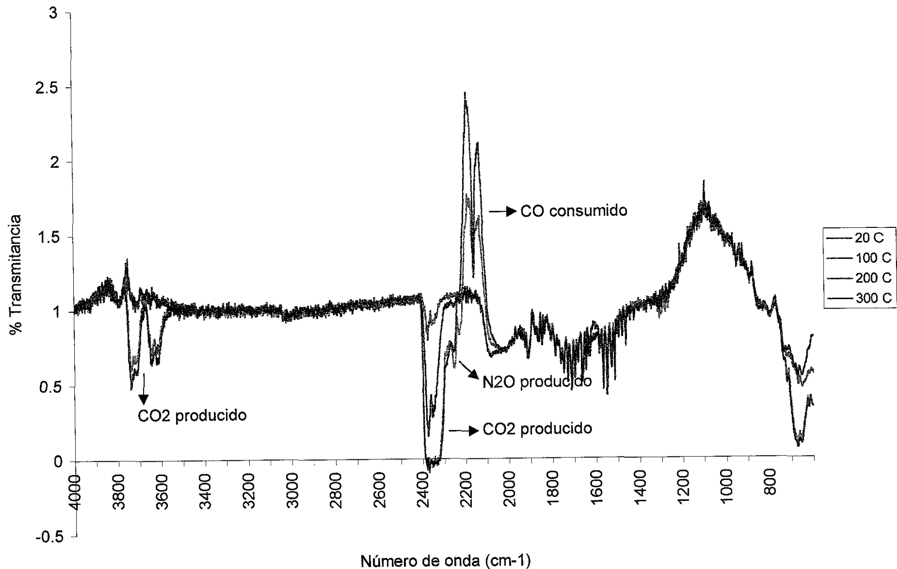
Fig. 23 Catalizador TLG3 (Temperatura ascendente)
