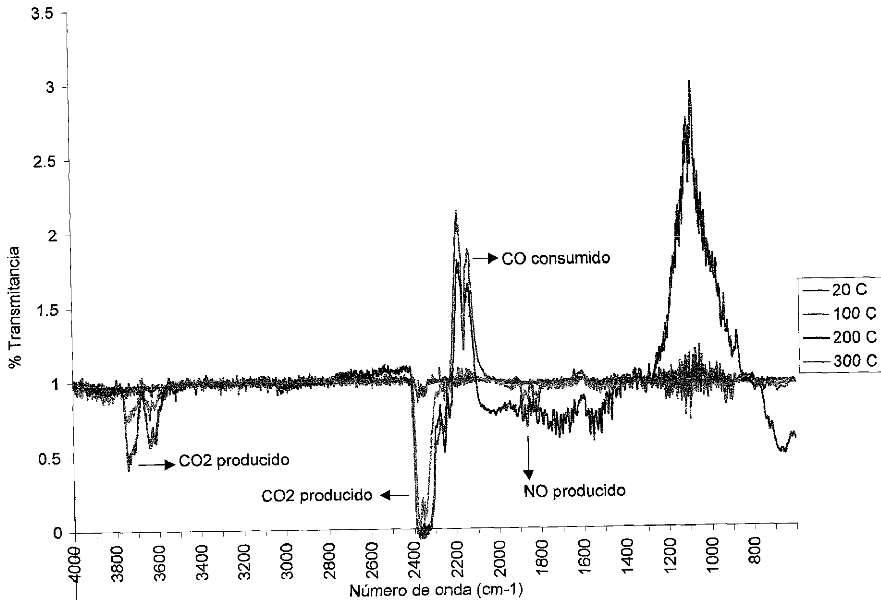
Fig. 22 Catalizador TLG3-300 (Temperatura ascendente sin aire)
