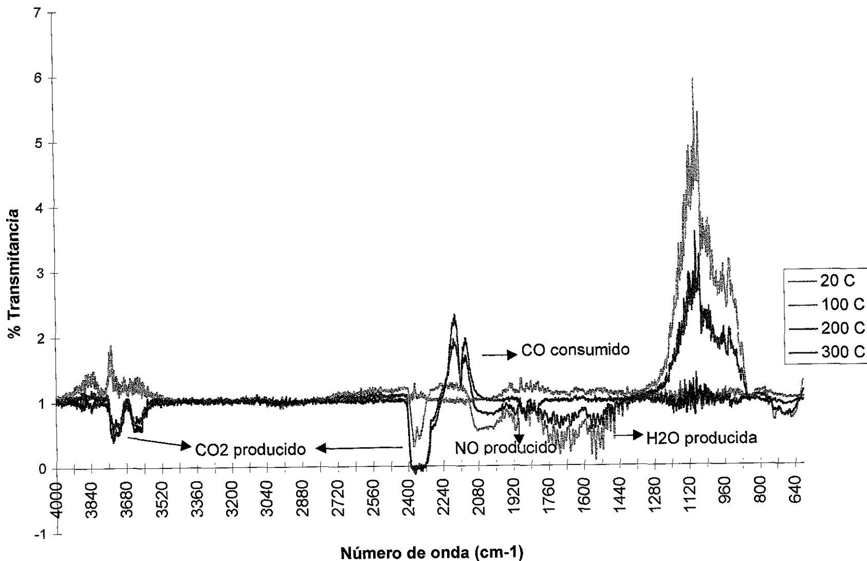
Fig. 19 Catalizador HEU-2 (Temperatura ascendente)
