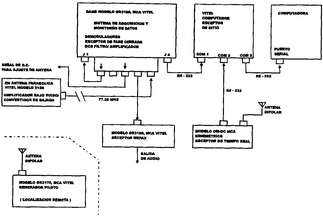
Figura 4.2 Diagrama a bloques del sistema de recepción via satélite.
