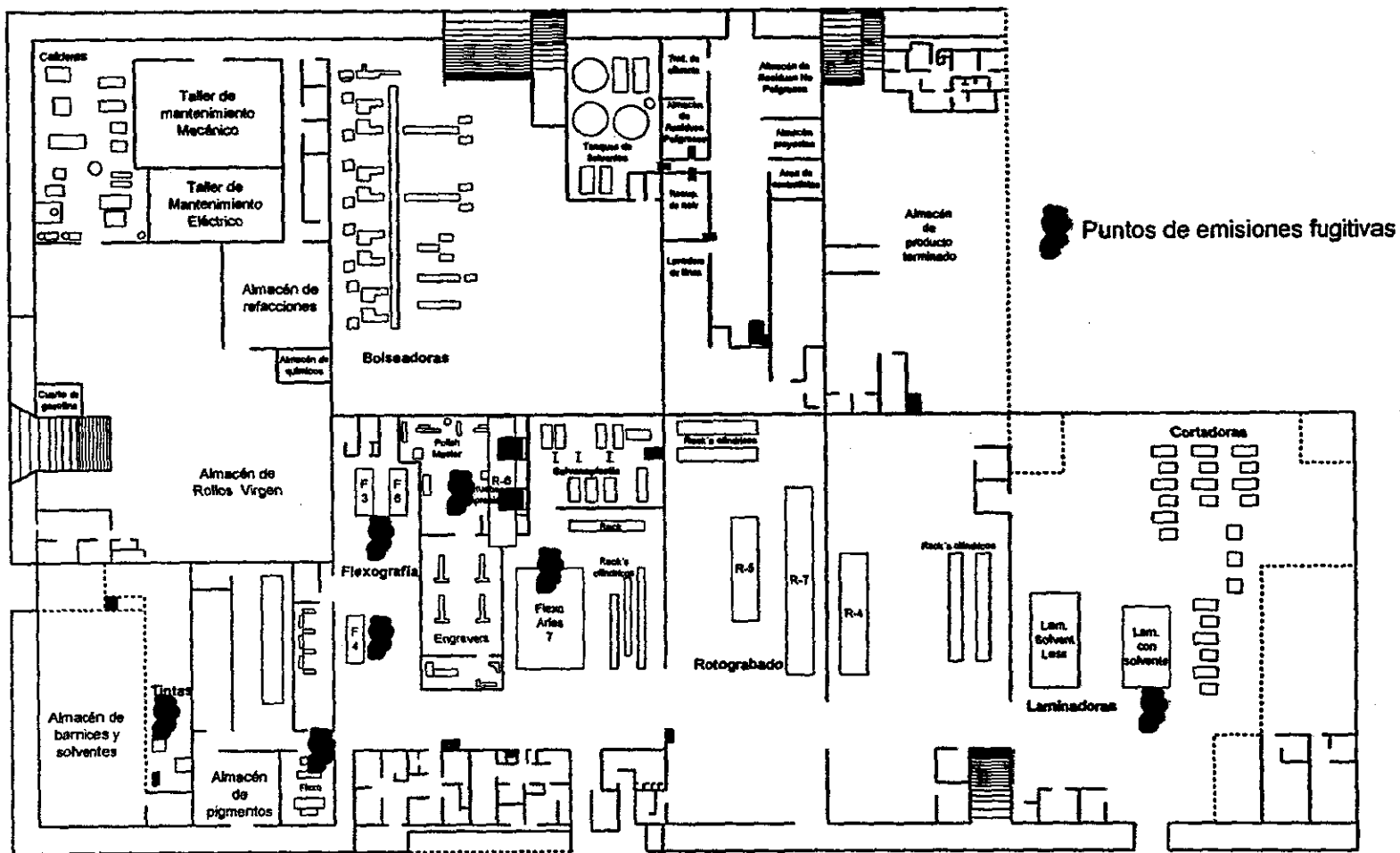
Fig. 2.5 Ubicación de las emisiones fugitivas de compuestos orgánicos volátiles
