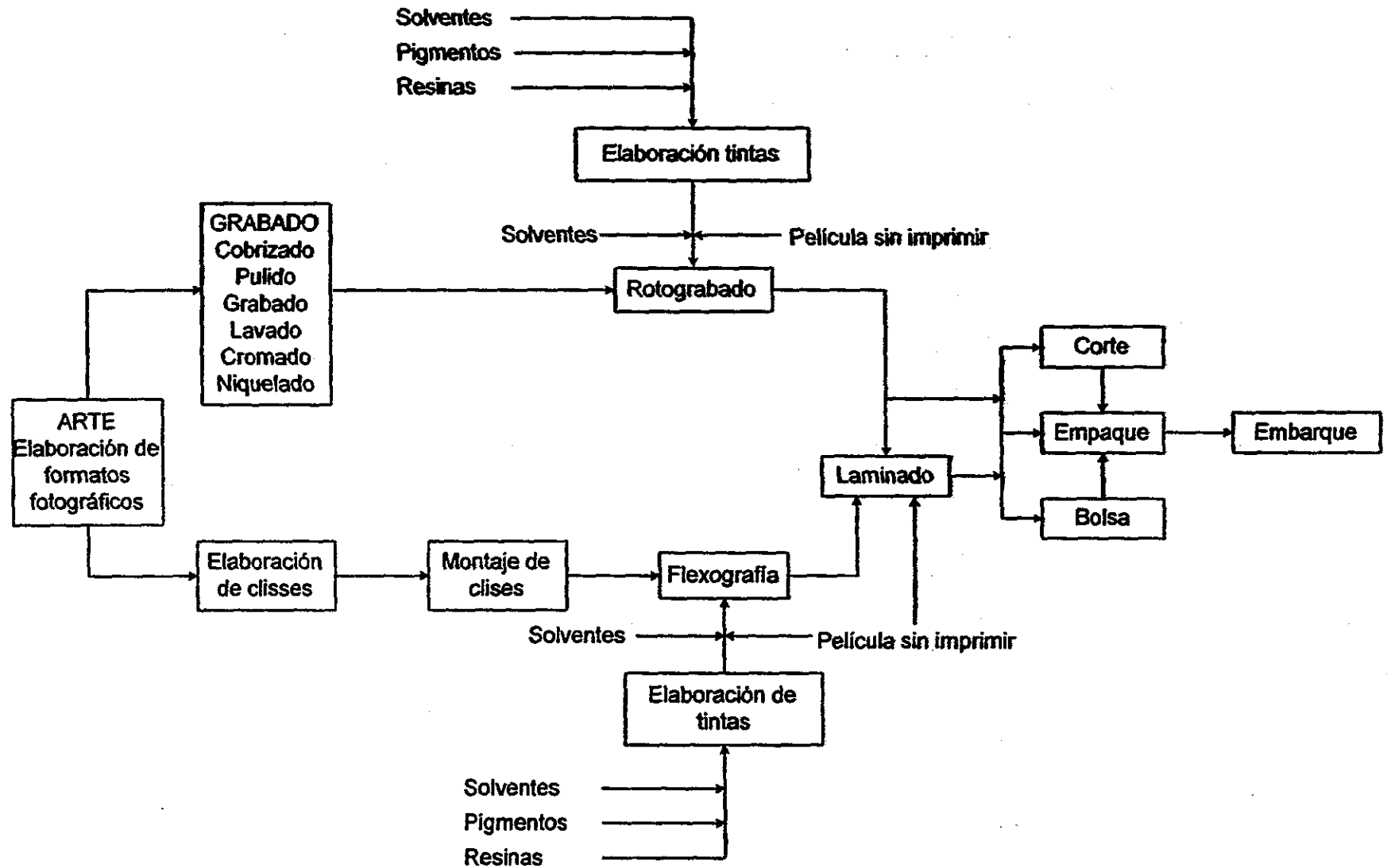
Fig. 2.1 Diagrama de bloques de proceso
