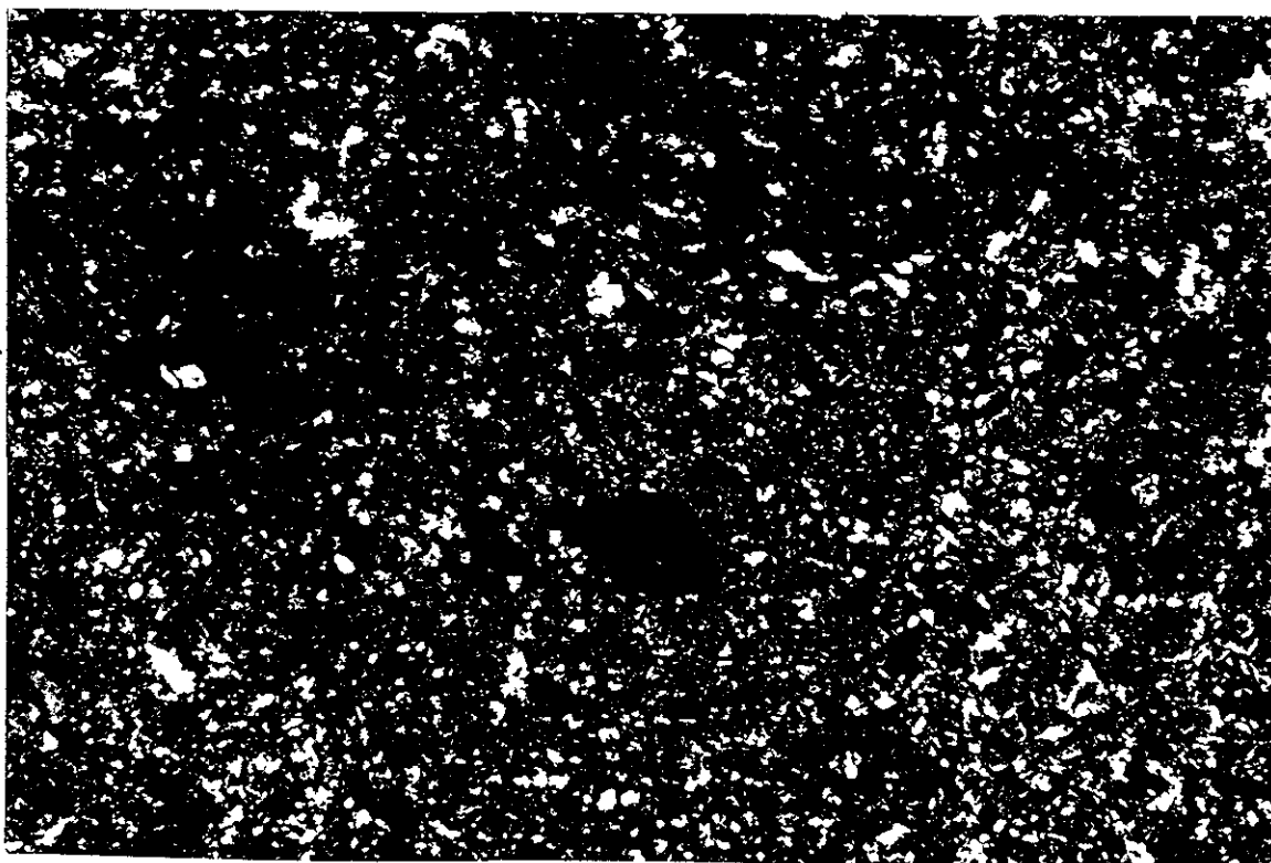
FOTOS 11 y 12.- Toba riolítica (ignimbrítica) donde se observa la vermiculosa textura soldada, tanto en fragmentos como en matriz tiende a desarrollarse un agregado cuarzo-feldespático; óxidos de hierro en negro. MUESTRA J-8, Formación Lista Blanca L.N. superior, L.P. inferior, 5X.
