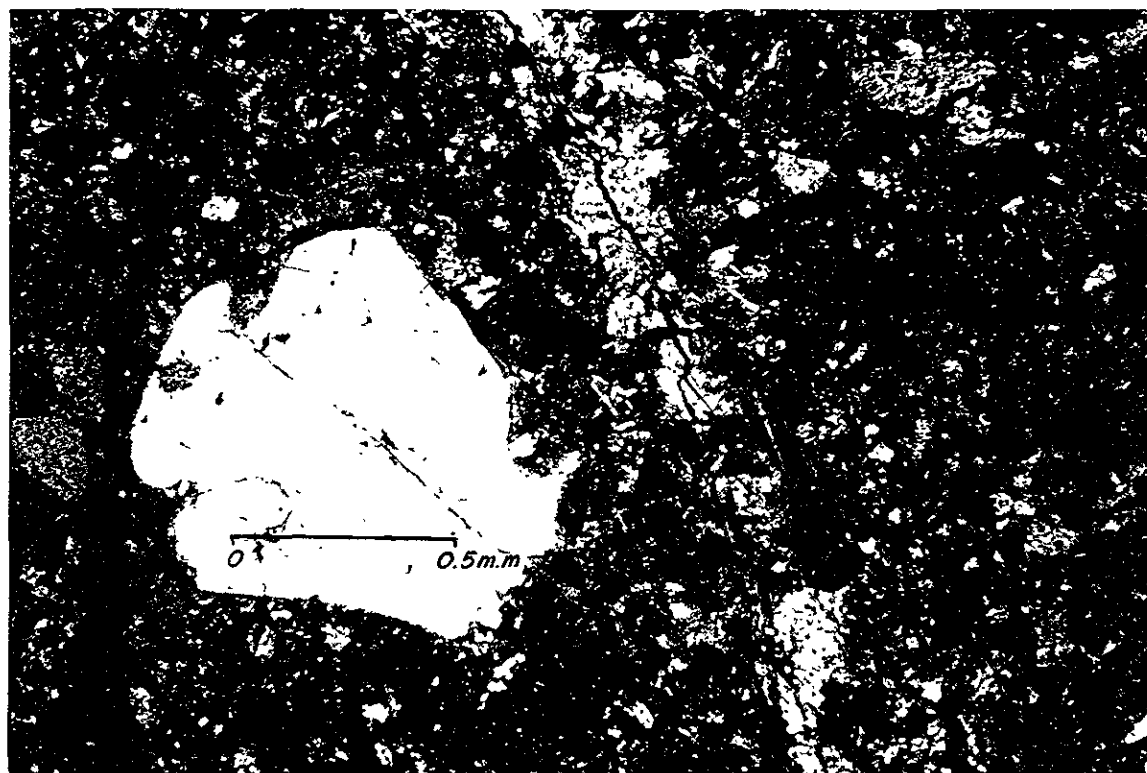
FOTOS 9 y 10.- Dos ejemplos de rocas de la Formación Tarahumara representadas por tobas de composición dacítica. de carácter Caracterizándose por cristales rotos de cuarzo y feldspatos, con biotita secundaria, epidota diseminada y de relleno de microfracturas; la matriz es cuarzo-feldespática. MUESTRAS J-23 y J-40, L.P. 5X. como
