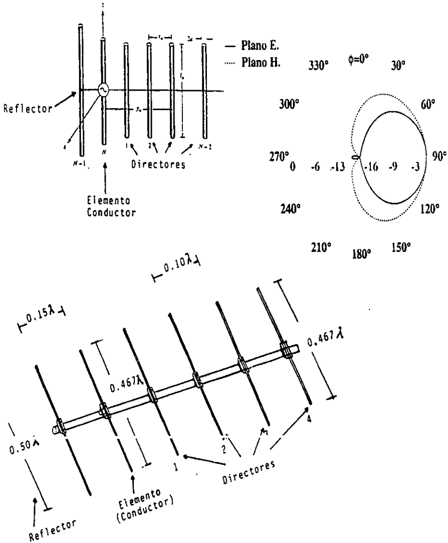
Fig. 3.7 Esquema y dimensiones básicas de la antena Yagi-Uda de 6 elementos, empleada en los radiomonitorios y su patrón de radiación asociado.
