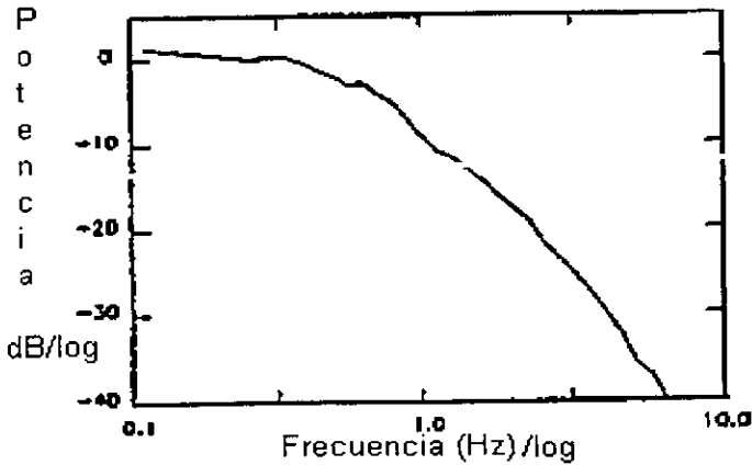
Figura 4.4 Espectro de potencia después de haber aplicado el método de promedio estadístico uniforme.
