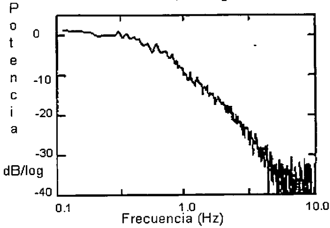
Figura 4.3 Espectro de potencia del centelleo después de haberle sustraído la contribución del ruido del sistema.
