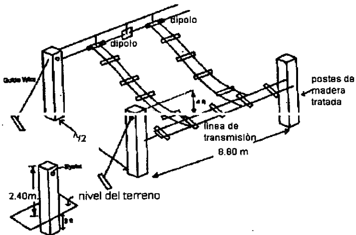
Fig. 3.4 Detalle de la configuración y dimensiones básicas de un dipolo y su acoplamiento a la línea de transmisión paralela.
