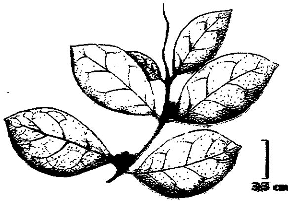
M. crassipes
