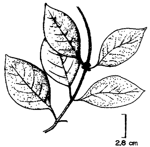
M. zimapanica
