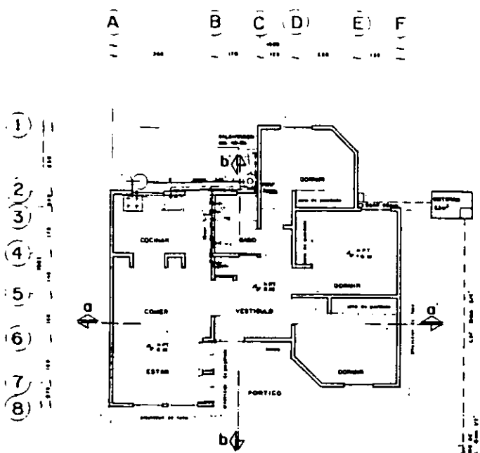
PLANTA ARQUITECTONICA
