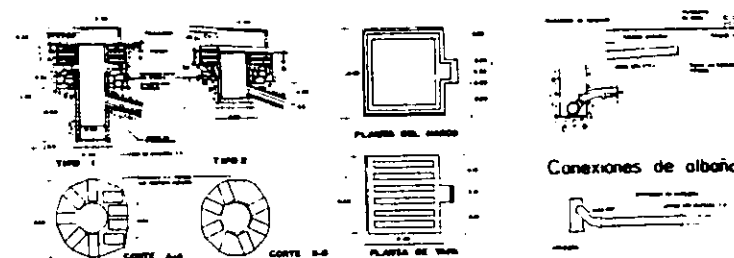
COLADERA PLUVIAL DE BANQUETA
