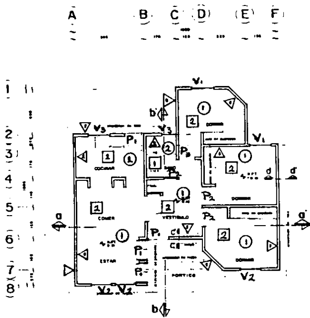
PLANTA ARQUITECTONICA
