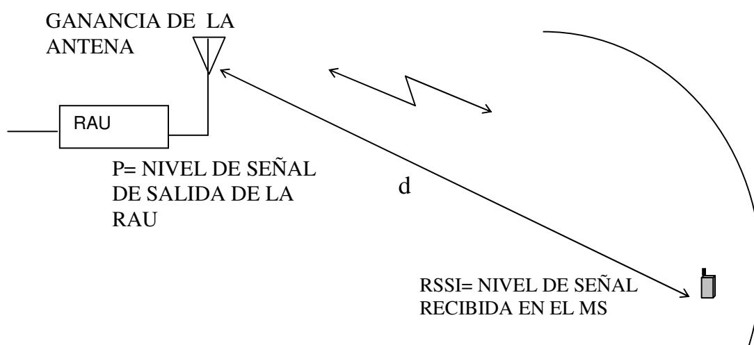
Figura IV.22. Trayectoria para determinar niveles de señal.
