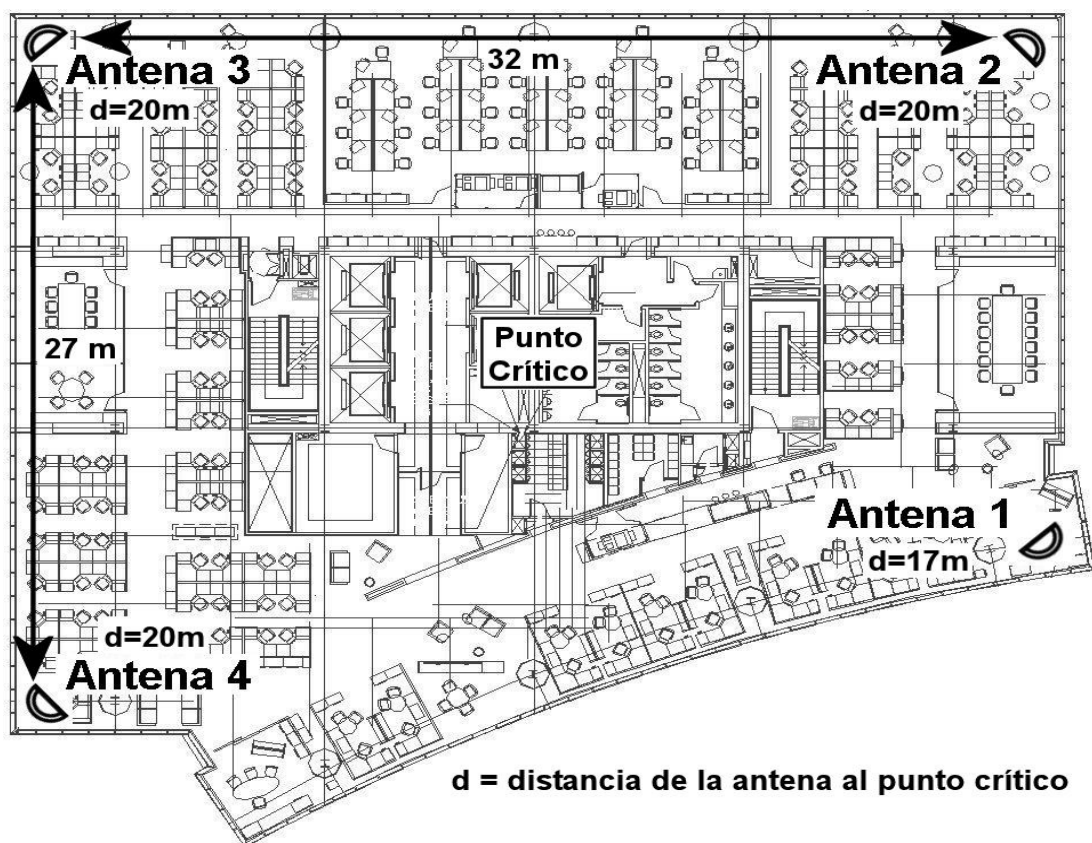
Figura IV.23. Diagrama de ubicación para 4 antenas.
