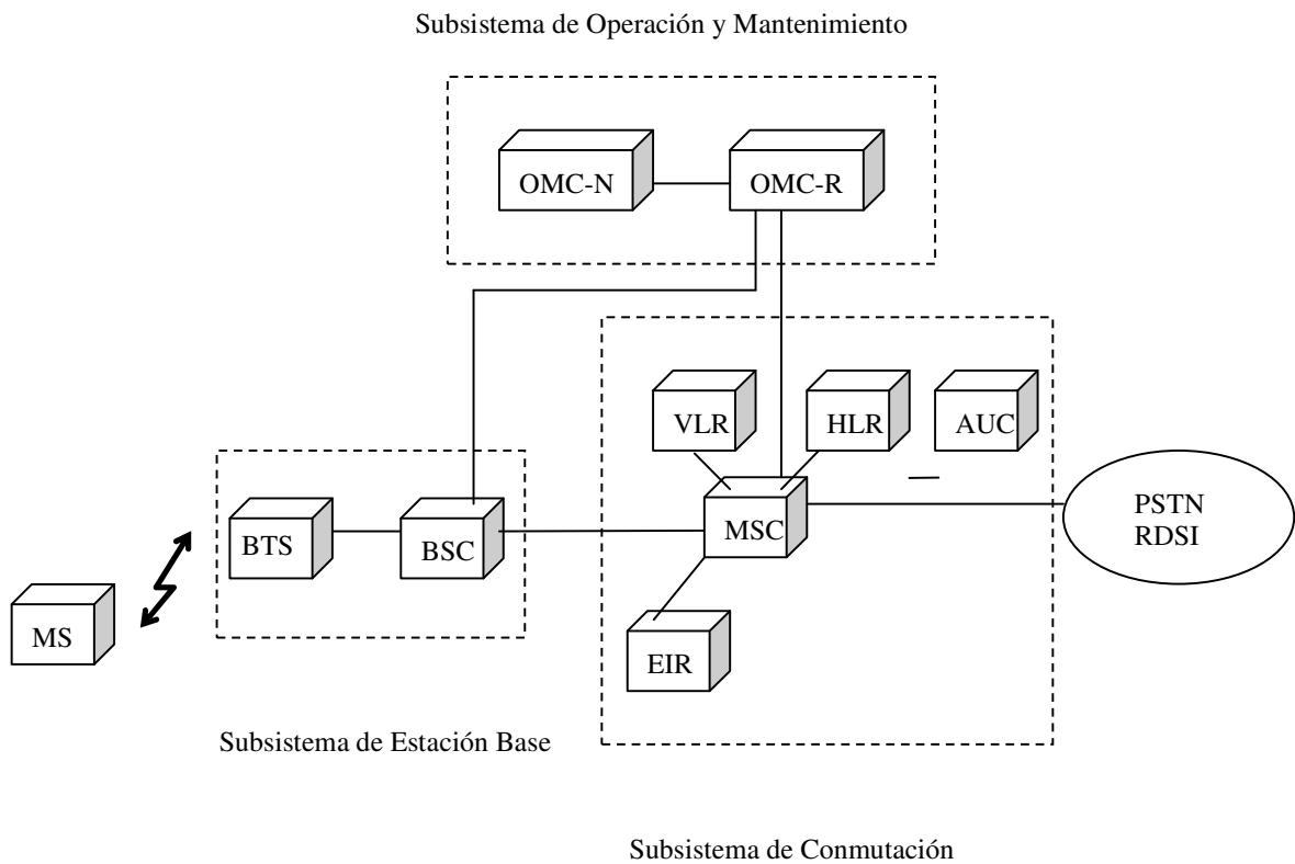
Figura II.1. Subsistemas en GSM.
