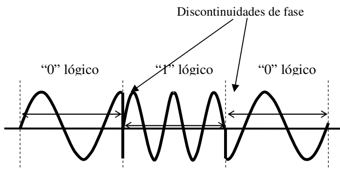
Figura II.6. Señal FSK discontinua.
