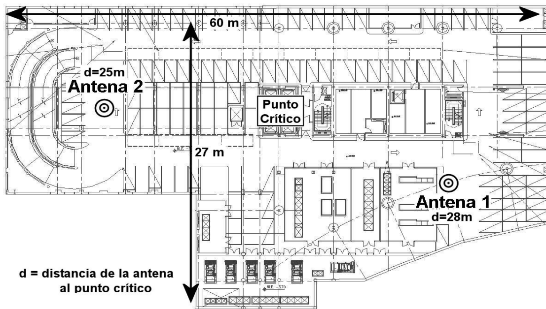
Figura IV.25. Diagrama de ubicación de antenas para los sótanos.
