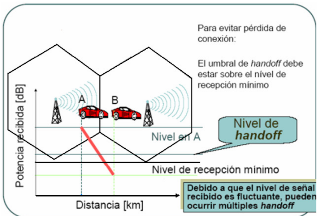
Figura III.4. Proceso de handover .
