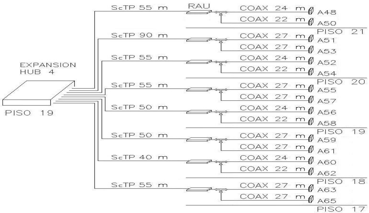
Figura V.6. Distribución de antenas conectadas al EXPANSION HUB 4.
