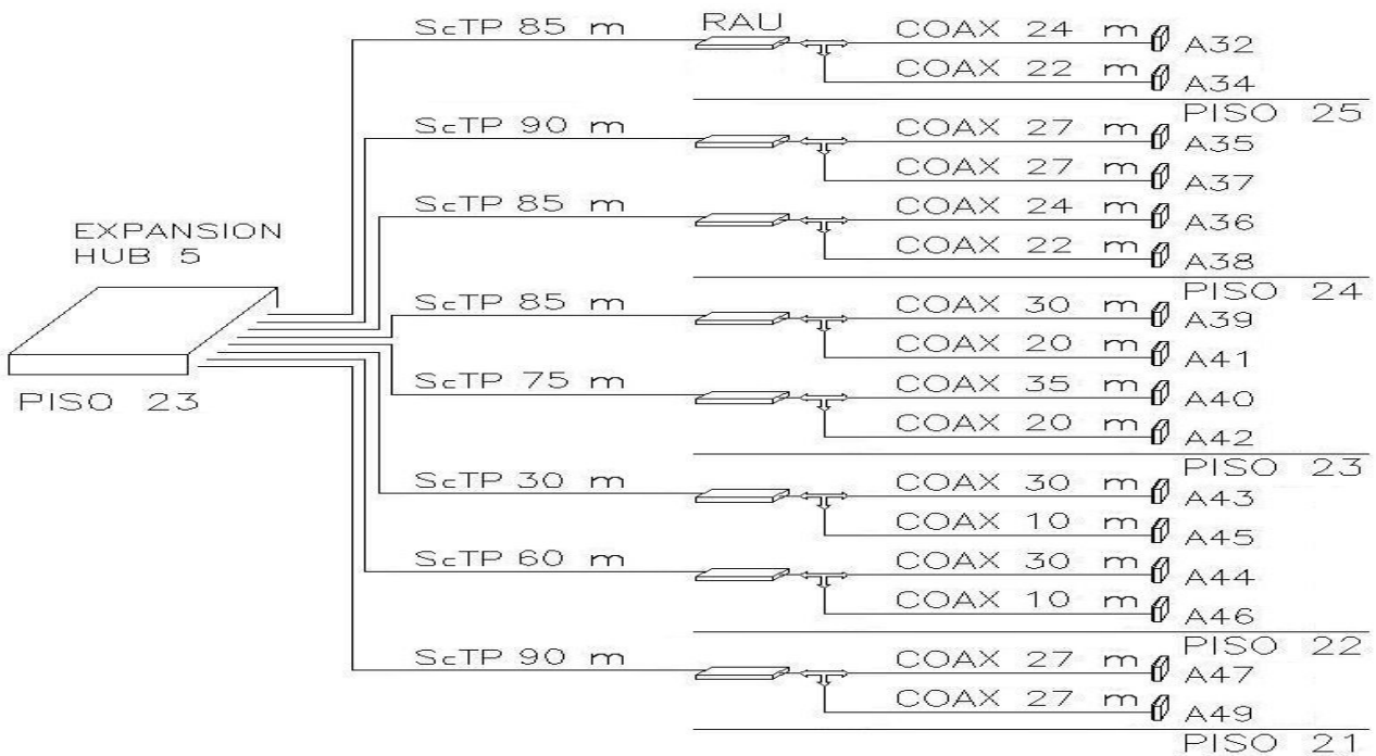
Figura V.7. Distribución de antenas conectadas al EXPANSION HUB 5.
