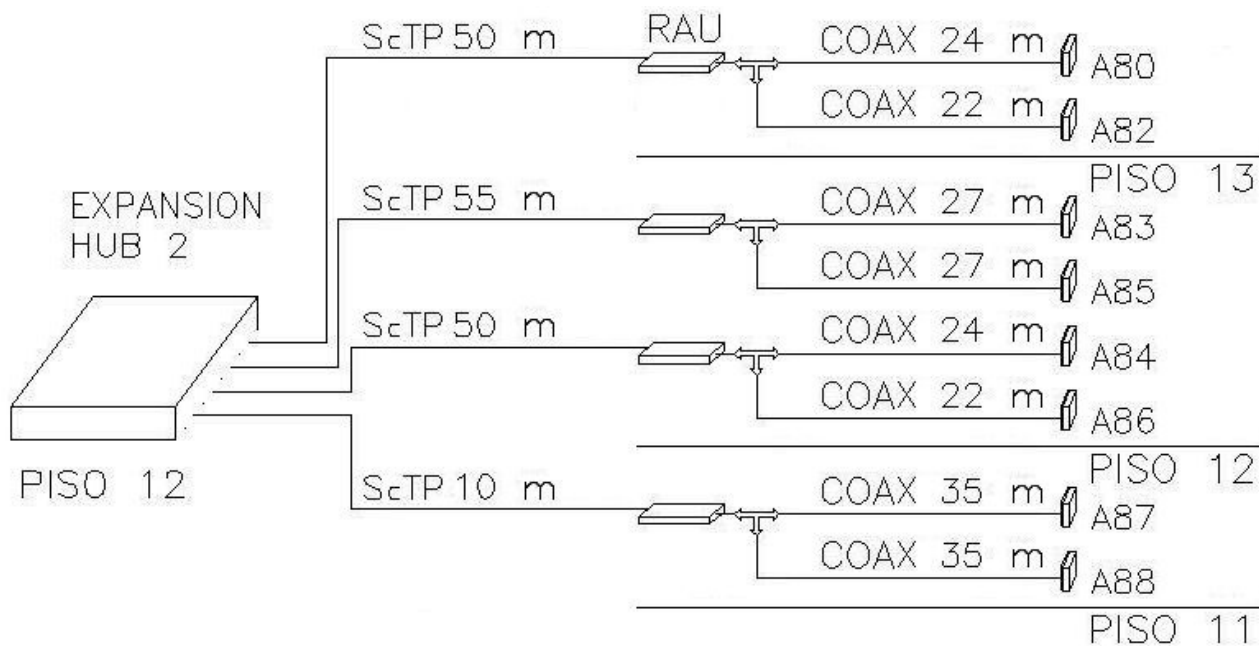
Figura V.4. Distribución de antenas conectadas al EXPANSION HUB 2.
