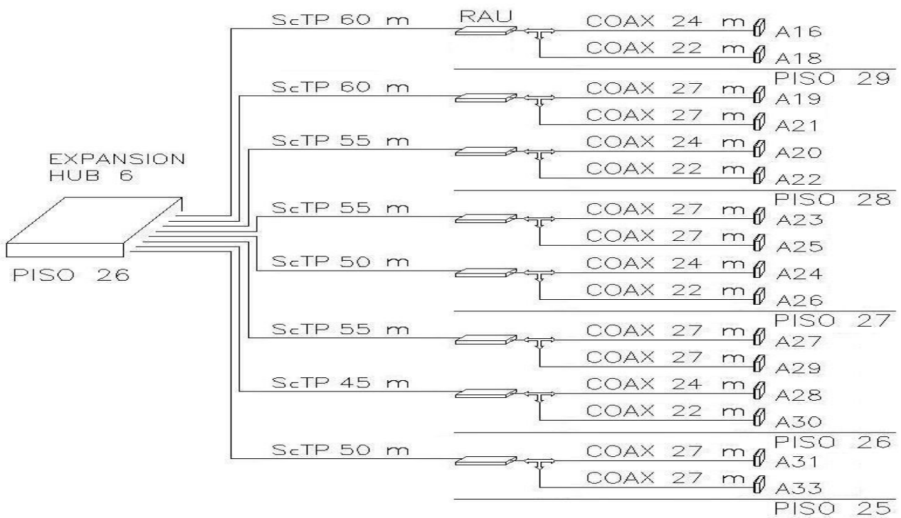
Figura V.8. Distribución de antenas conectadas al EXPANSION HUB 6.
