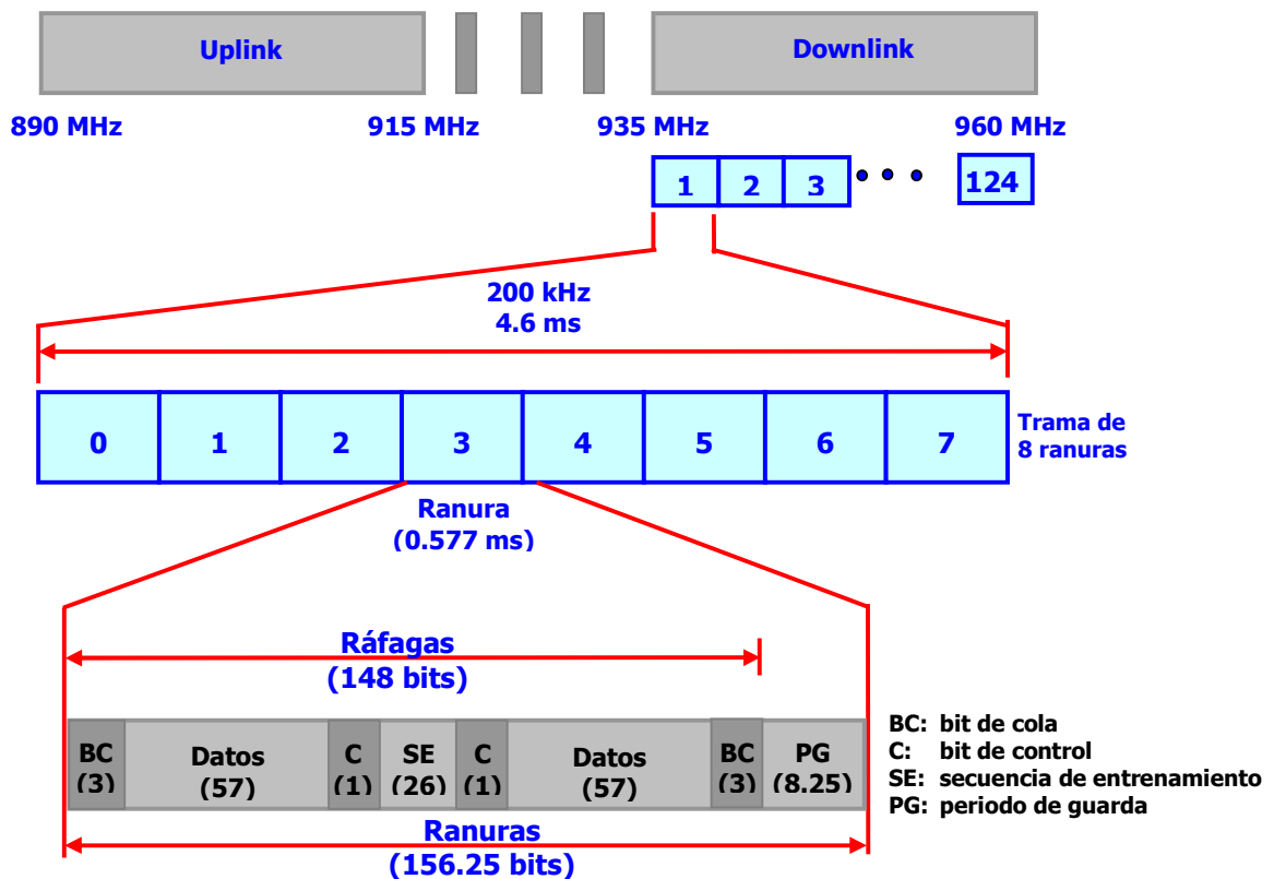
Figura II.9. FDMA y TDMA en GSM.
