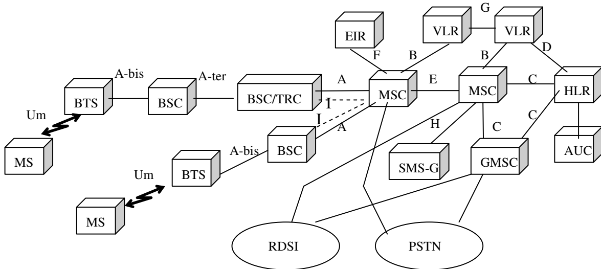
Figura II.5. Interfaces en GSM.
