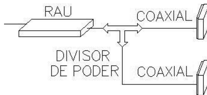
Figura V.2. Conexión típica de antenas a los RAUs.
