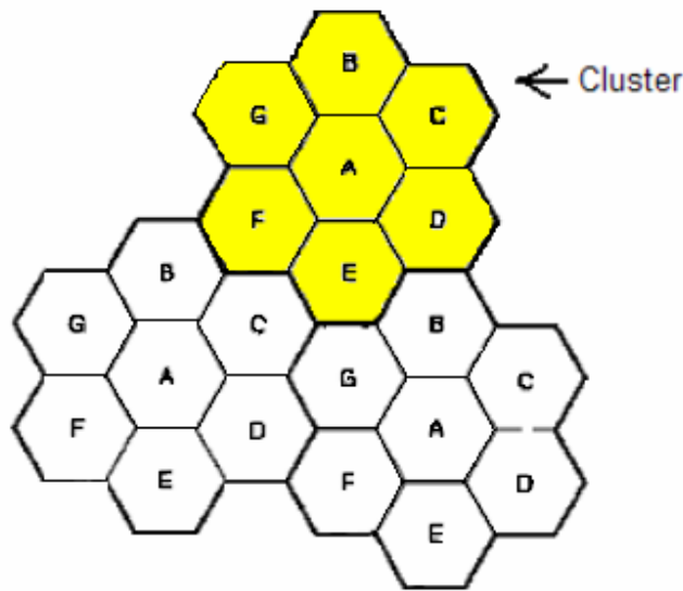
Figura 1.7. Concepto de reutilización celular de frecuencias.
