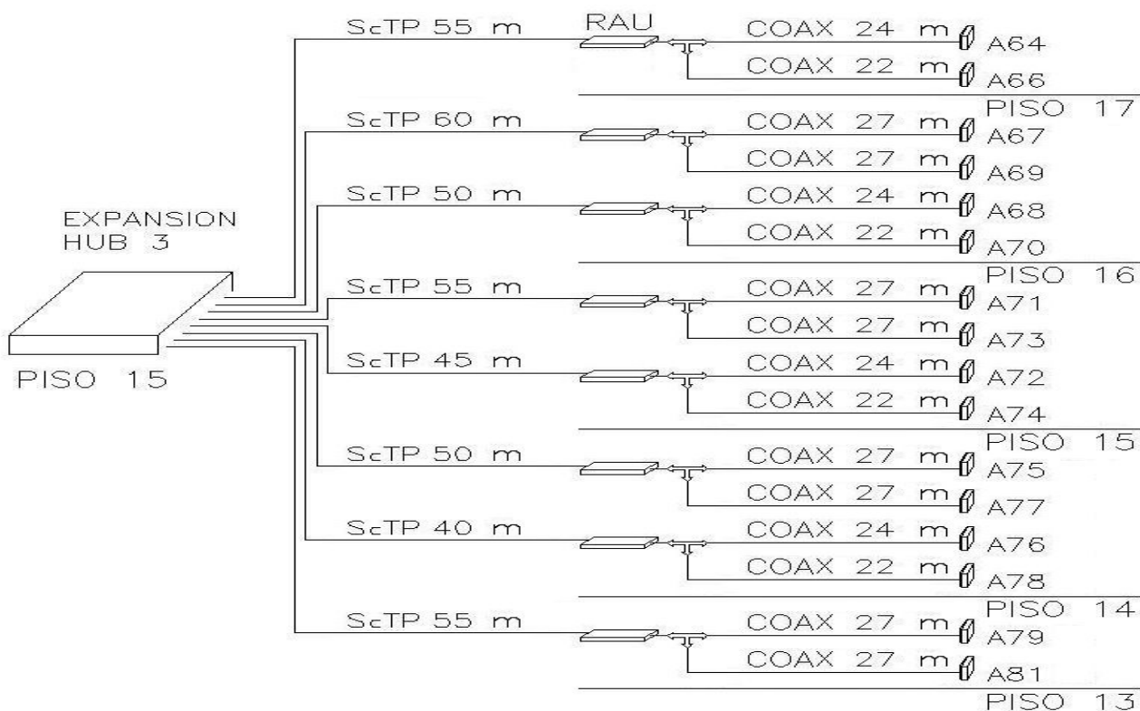
Figura V.5. Distribución de antenas conectadas al EXPANSION HUB 3.
