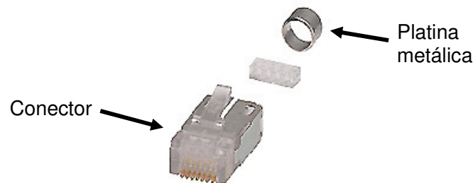
Figura IV.21. Conector RJ-49.
