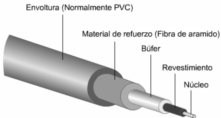
Figura IV.18. Fibra óptica.
