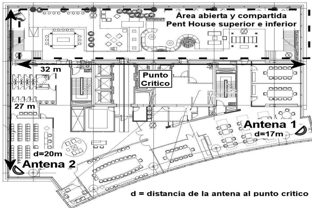
Figura IV.24. Diagrama de ubicación para 2 antenas.
