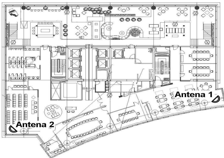
Figura V.14. Posición de 2 antenas para pisos tipo penthouse.
