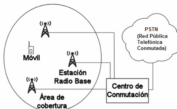
Figura I.5. Diagrama básico de una red celular.
