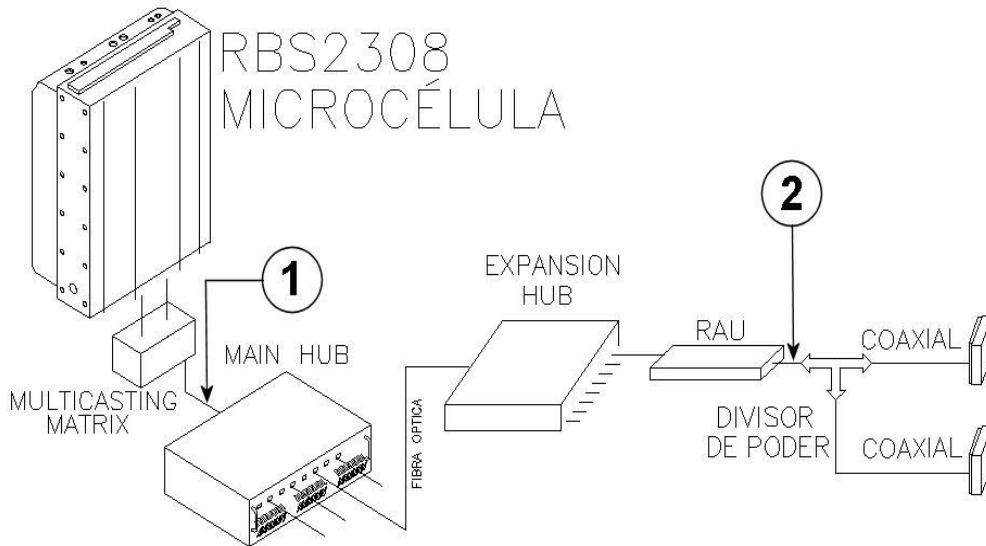
Figura V.16. Puntos de medición de potencia.
