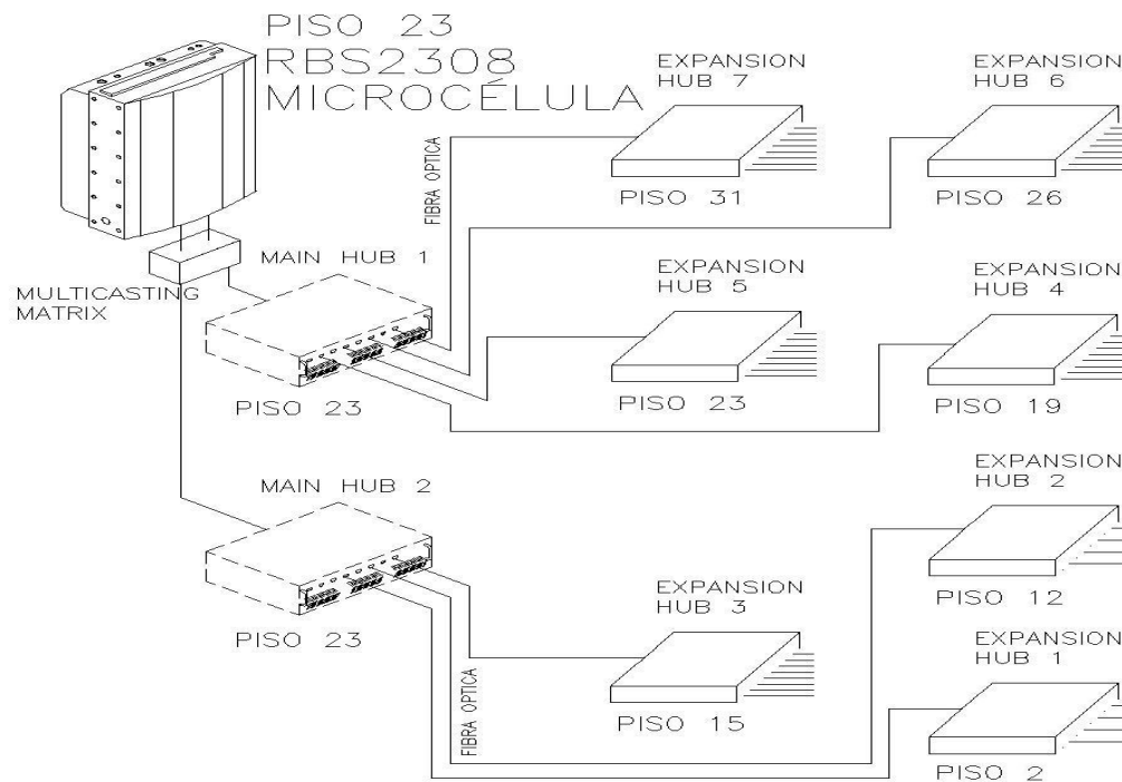
Figura V.1. Diagrama a bloques de distribución del equipo.
