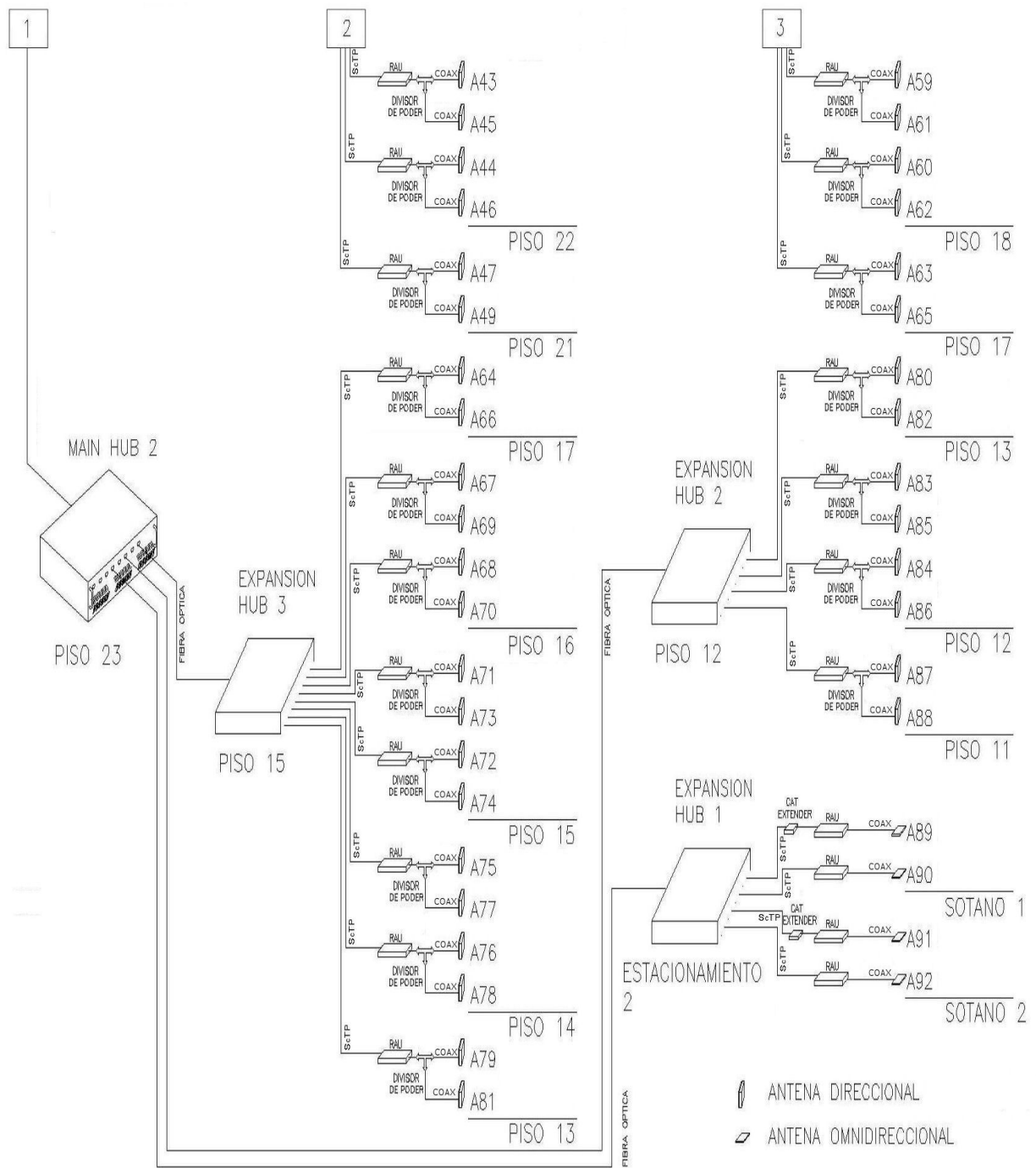
Figura IV.26. Diagrama a bloques para la implementación de la microcélula.
