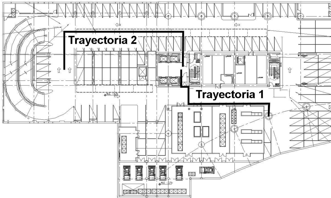
Figura V.12. Distribución de cableado para sótanos.
