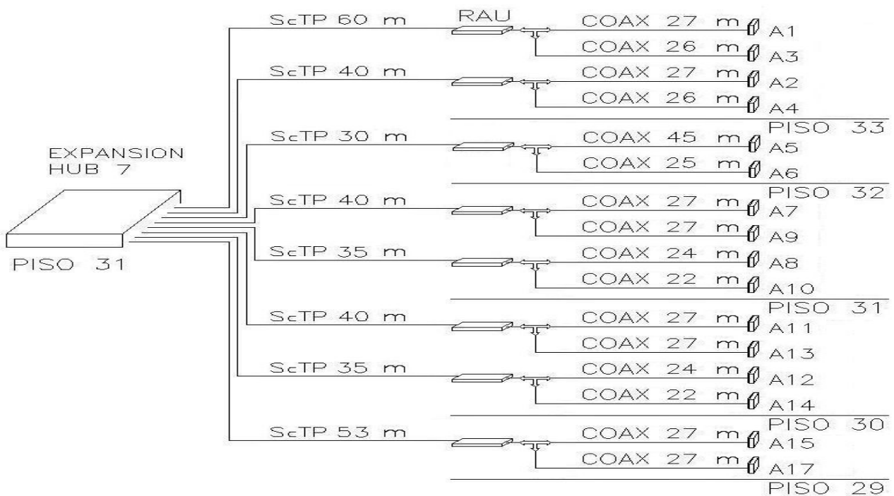
Figura V.9. Distribución de antenas conectadas al EXPANSION HUB 7.
