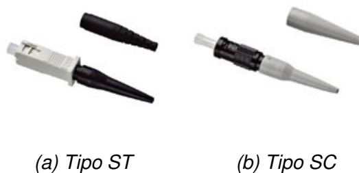
Figura IV.19. Tipos de conectores para fibra óptica.
