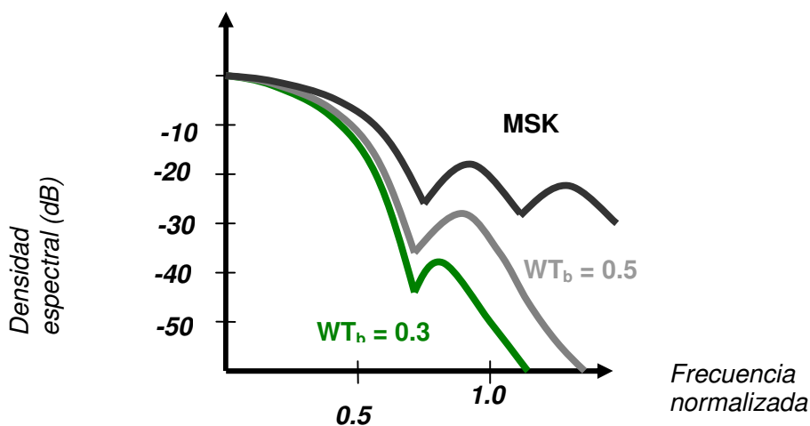
Figura II.8. Gráfica Frecuencia - Densidad espectral.
