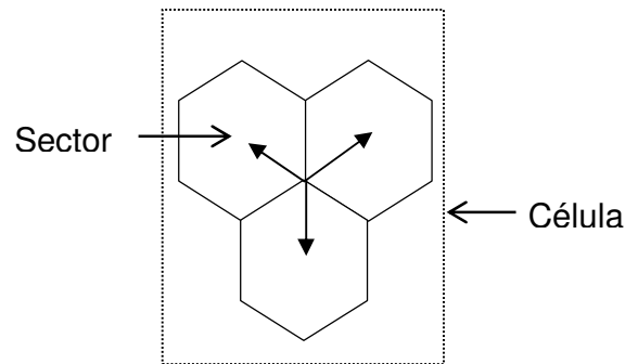
Figura I.11. Célula dividida en tres sectores de 120 grados.
