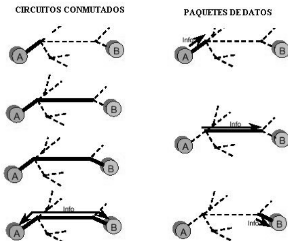
Figura 4.16. Circuitos conmutados y paquetes de datos.
