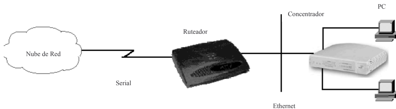
Figura 4.14. Equipos de interconexión físicos.
