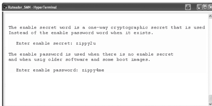
Figura 5.20. Contraseña enable secret y enable password .
