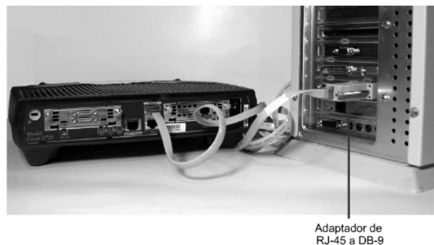
Figura 5.13. Conexión de una computadora al puerto de consola del router.
