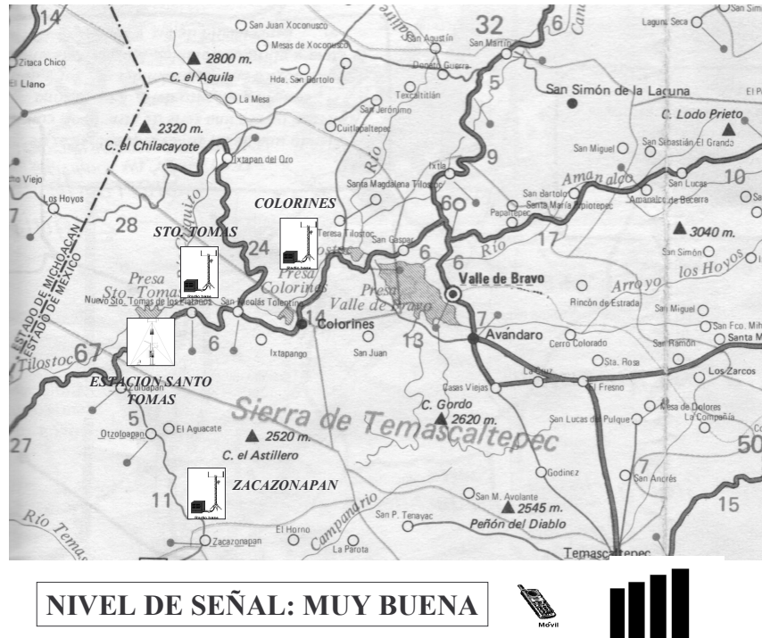
Figura 5.5. Ubicación y cobertura de la estación Santo Tomás.
