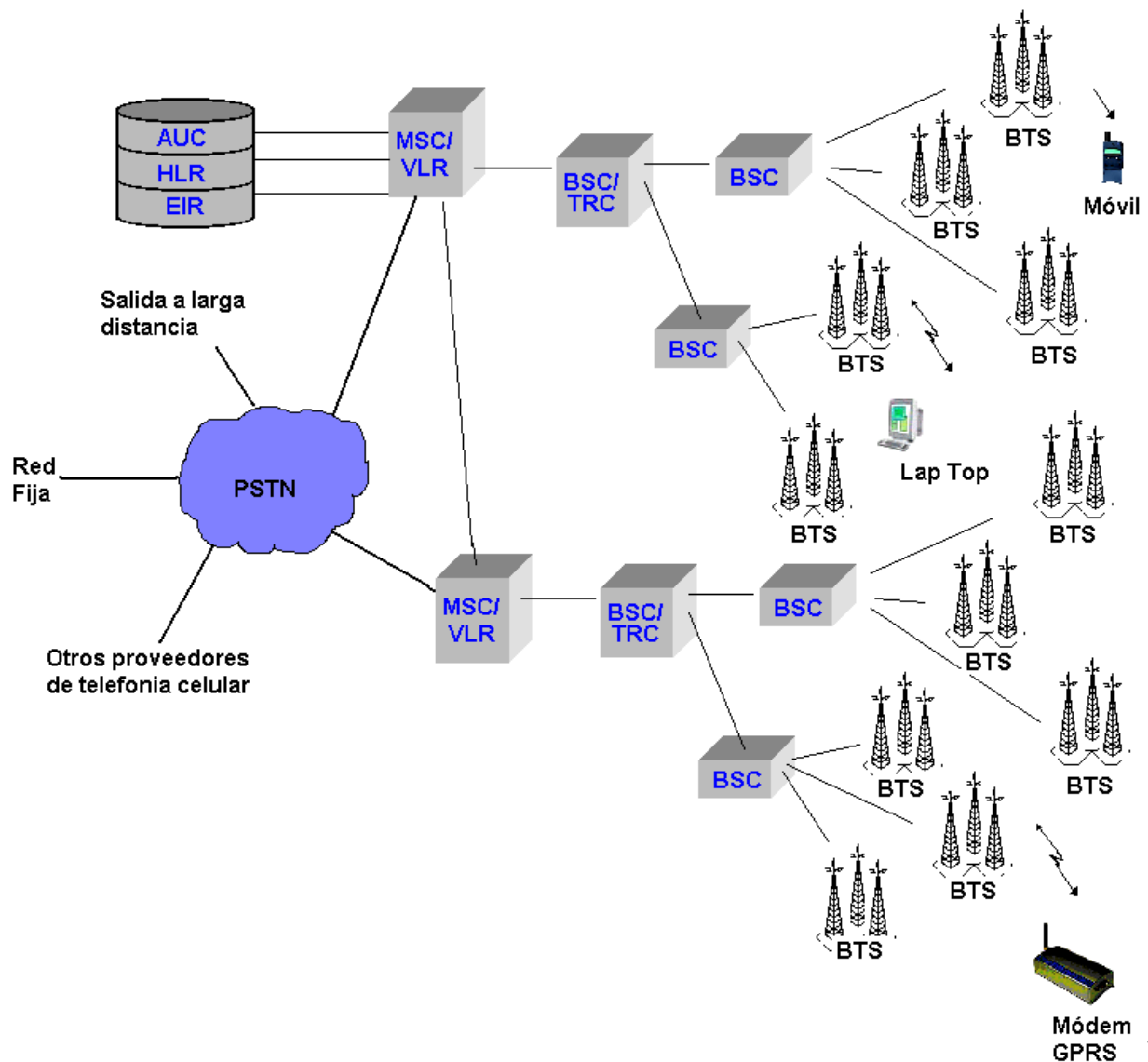
Figura 2.6. Diagrama de los elementos de registro para validación de usuario.
