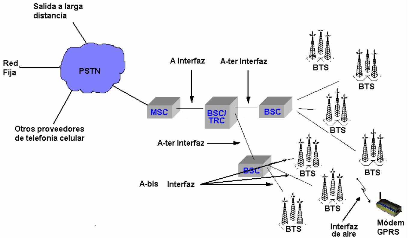
Figura 2.5. Interfaces para interconexión de GSM.
