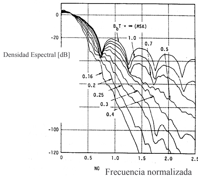
Figura B.3 . Densidad de potencia espectral de una señal.
