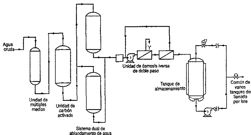
Figura 2.1 Sistema tradicional de distribución de agua.
