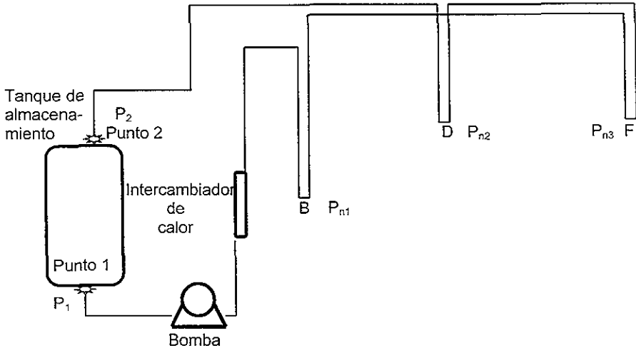
Figura 4.4 Sistema de distribución propuesto (ver Anexo B).
