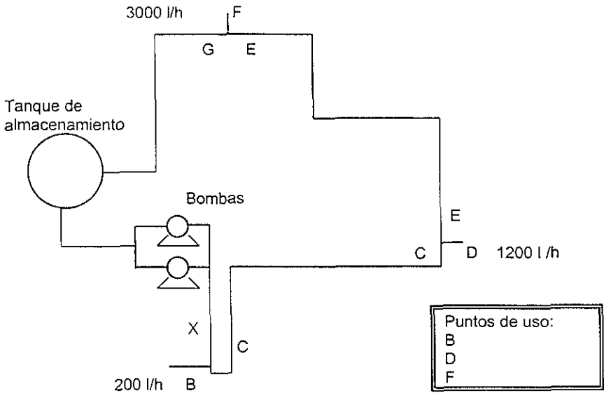
Figura 4.3 Selección de tubería.
