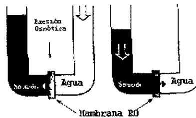
Figura 1.7 Ósmosis inversa.
