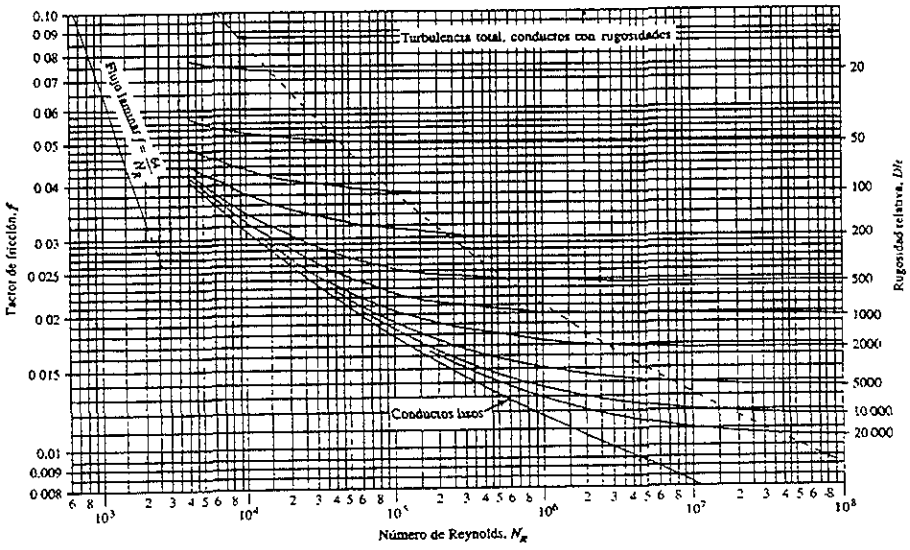
Gráfica 2 Diagrama de Moody.
