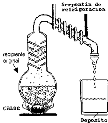
Figura 1.1 Destilación.
