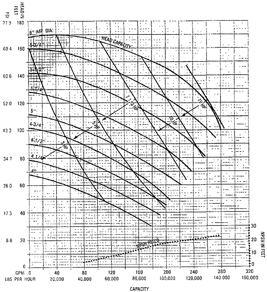
Gráfica 1 Curva de comportamiento de la bomba.
