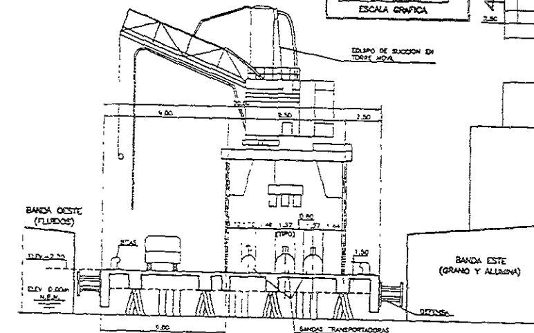
MUELLE EN ESPIGON CORTE A - A
