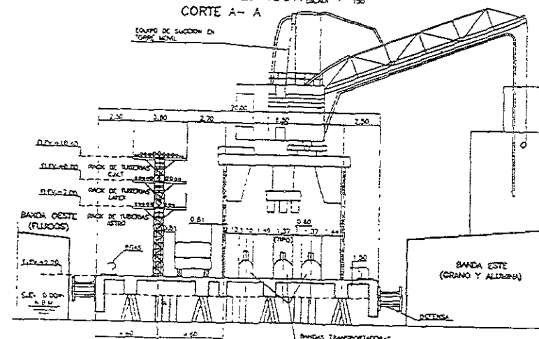
MUELLE EN ESPIGON CORTE B - B
