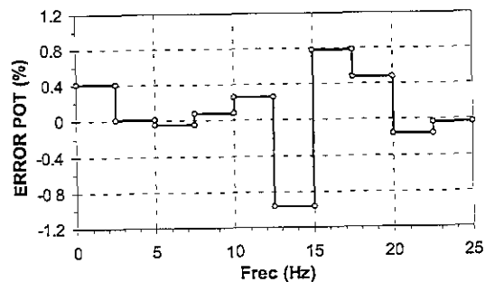
d) Variación de ERROR POT con la frecuencia.
