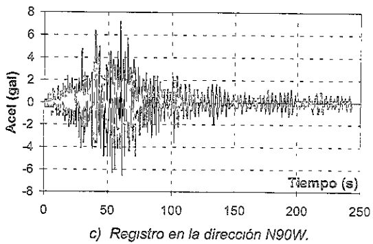
Figura 4.17 Registros a z=30 m del sismo del 24/10/93.
