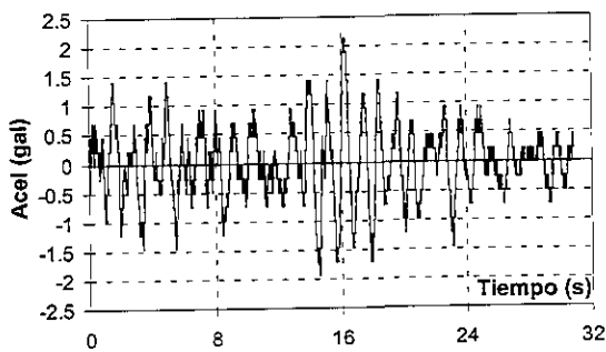
a) Registro en la dirección N00E.
