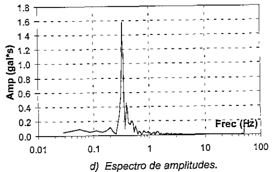
Figura 4.11 Registros a z=12 m del sismo del 10/09/93.
