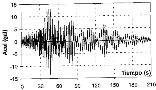
c) Registro en la dirección N90W.
