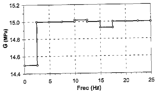
a) Variación de G con la frecuencia.
