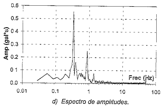
Figura 4.16 Registros a z=30 m del sismo del 10/09/93.
