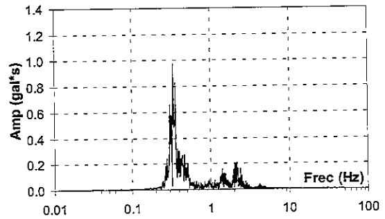
b) Espectro de amplitudes.
