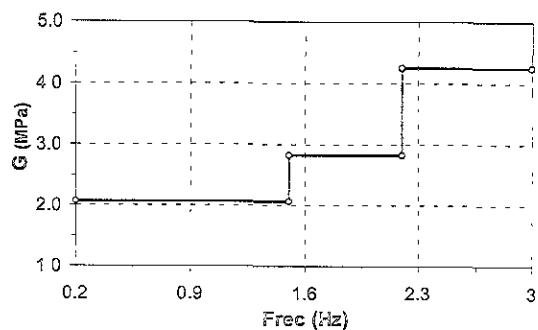
a) G vs Frec en 23/05/94 - N00E.
