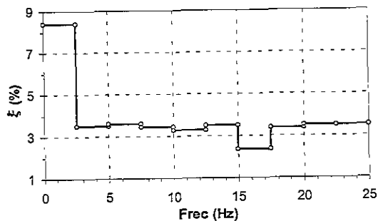
b) Variación de xi con la frecuencia.
