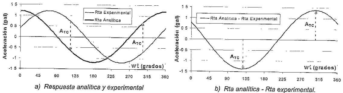
Figura 3.7 Interpretación matemática de la Ecuación 3.1.
