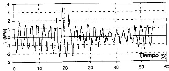
g) Esfuerzo cortante a h=12 m.
