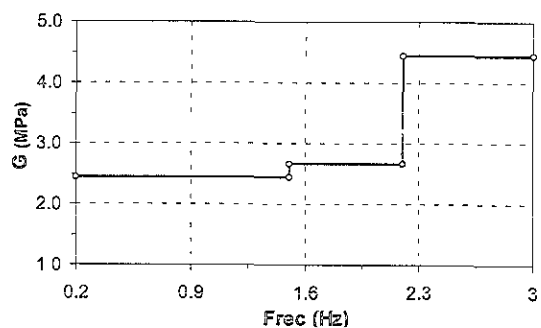
c) G vs Frec en 23/05/94 - N90W.
