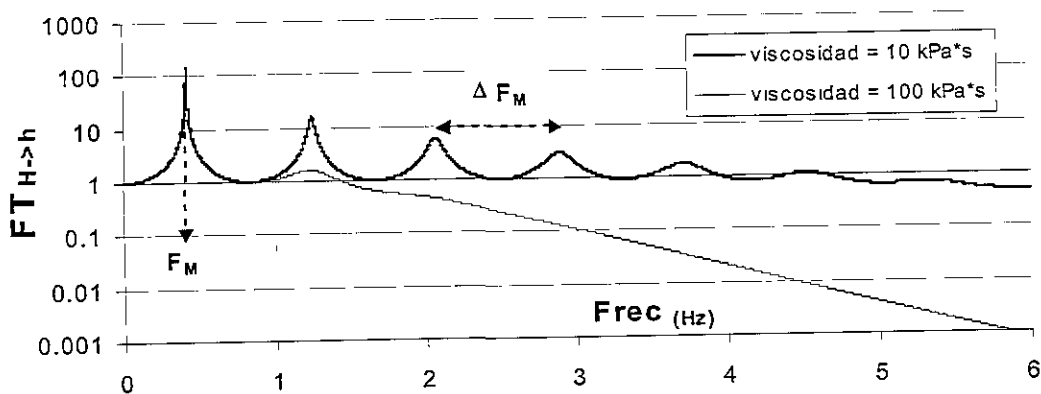
Figura 2.23 Topología de FT_{H \rightarrow h} entre H=30 m y h=0 m para diferentes \eta .
