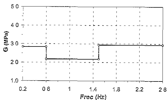
e) G vs Frec en 10/12/94 - N00E.
