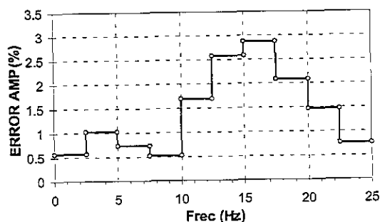
c) Variación de ERROR AMP con la frecuencia.
