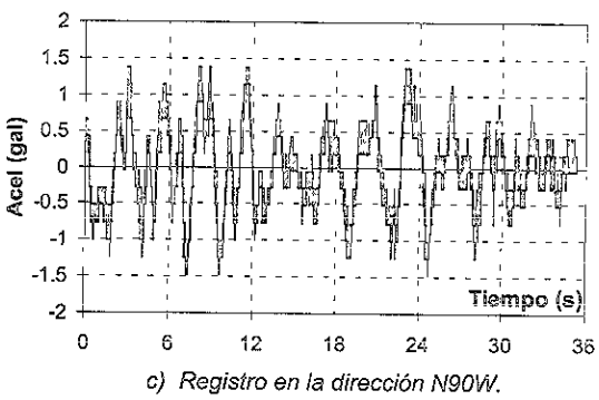
Figura 4.16 Registros a z=30 m del sismo del 10/09/93.
