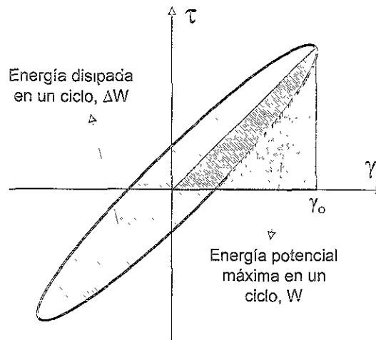
Figura 2.7 Interpretación gráfica del amortiguamiento viscoso (Ecuación 2.6).
