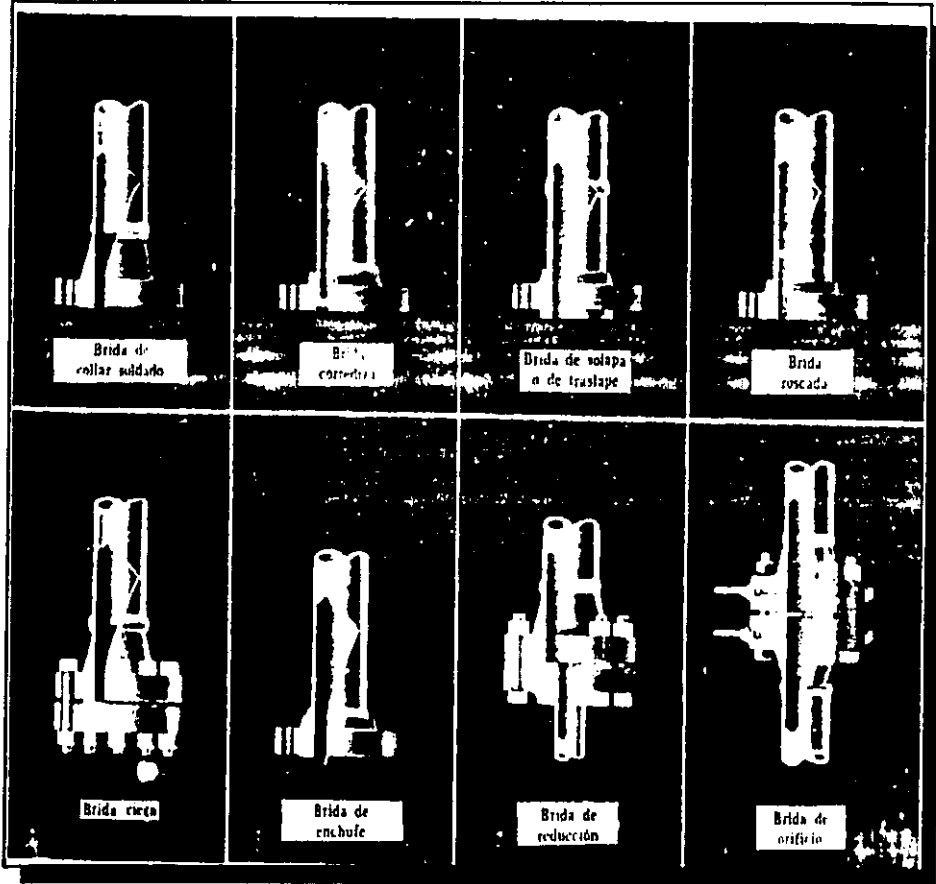
FIGURA 3.4 VARIOS TIPOS TÍPICOS DE BRIDAS
