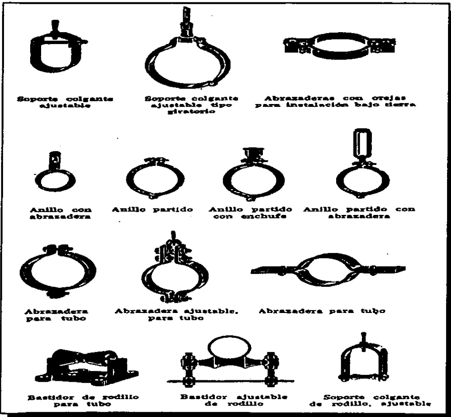
FIGURA 3.20 ALGUNOS TIPOS DE SOPORTES Y COLGANTES PARA TUBOS
