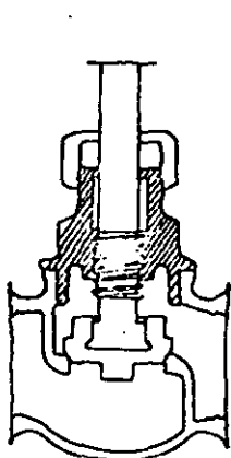
BONETE ROSCADO
