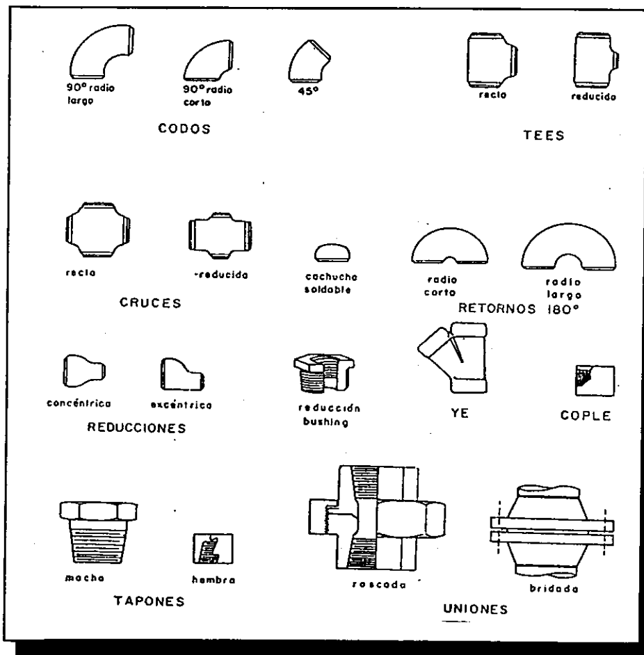
FIGURA 3.3 ALGUNOS DE LOS DIFERENTES TIPOS DE ACCESORIOS
