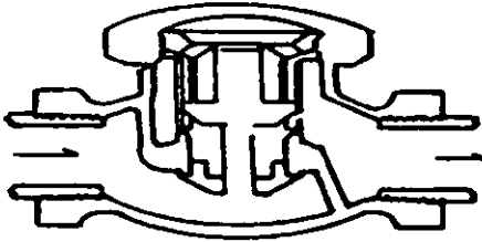
TIPO PISTON
