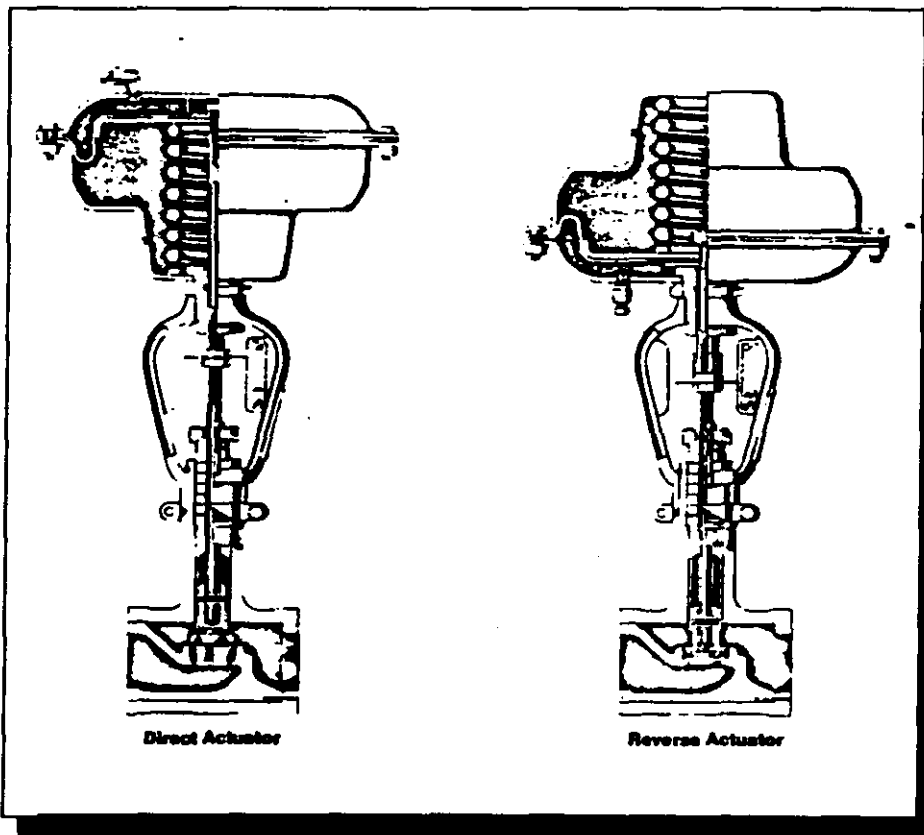
FIGURA 3.5 Actuadores (tipo directo e invertido)
