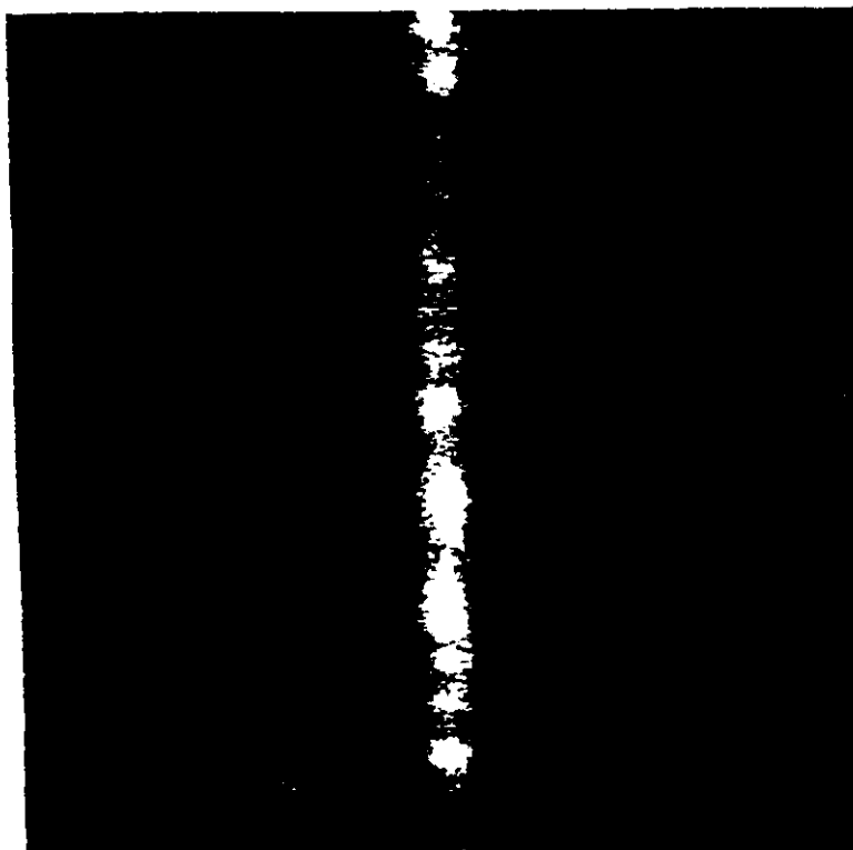
FALTA DE FUSION DE LA PARED LATERAL (LOF) Vacíos alargados entre los cordones de la soldadura y las superficies de las juntas.
