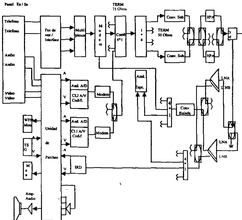
Figura 6.1. Diagrama general de la estación terrena móvil transportable.
