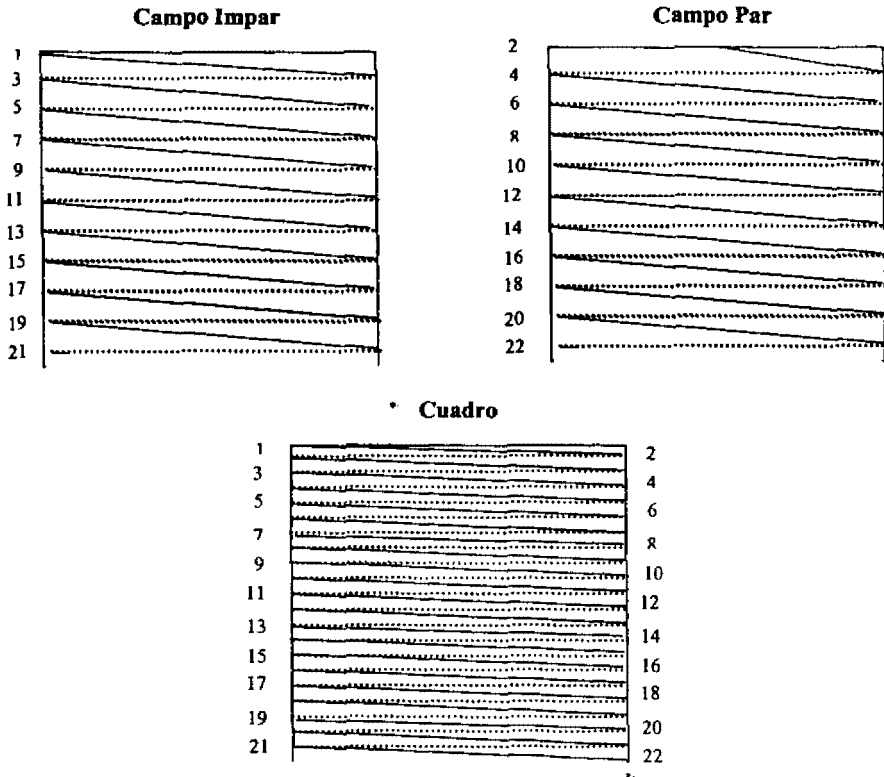
Figura 2.6. Barrido entrelazado en el sistema de TV NTSC.
