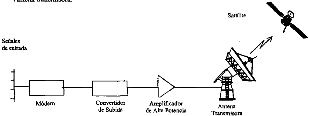
Figura 4.1. Configuración de una Estación Terrena Transmisora.
