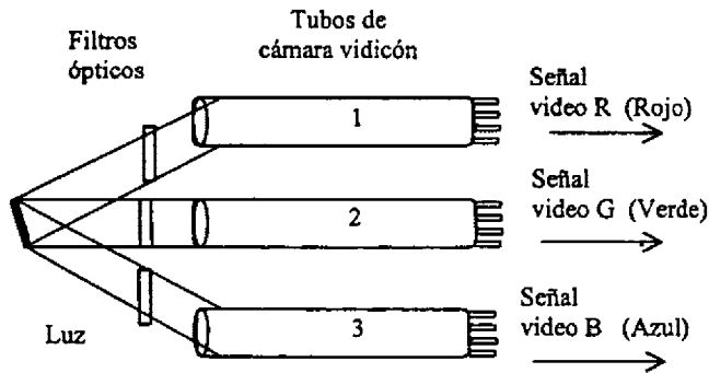
Figura 2.8. Tres tubos de cámara vidicon produciendo las señales video R, G y B para los colores rojo, verde y azul de la imagen.
