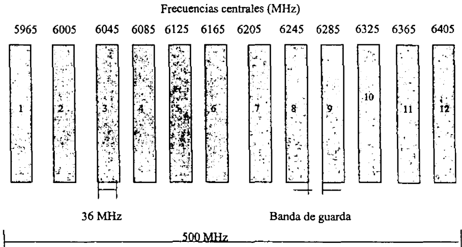
Figura 3.13. Configuración del espacio de frecuencia de un transponder de 36 MHz.
