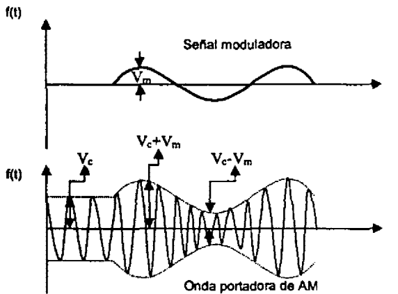
Figura 2.12. Característica de una onda de AM.
