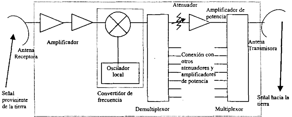
Figura 3.12. Subsistema de comunicaciones.
