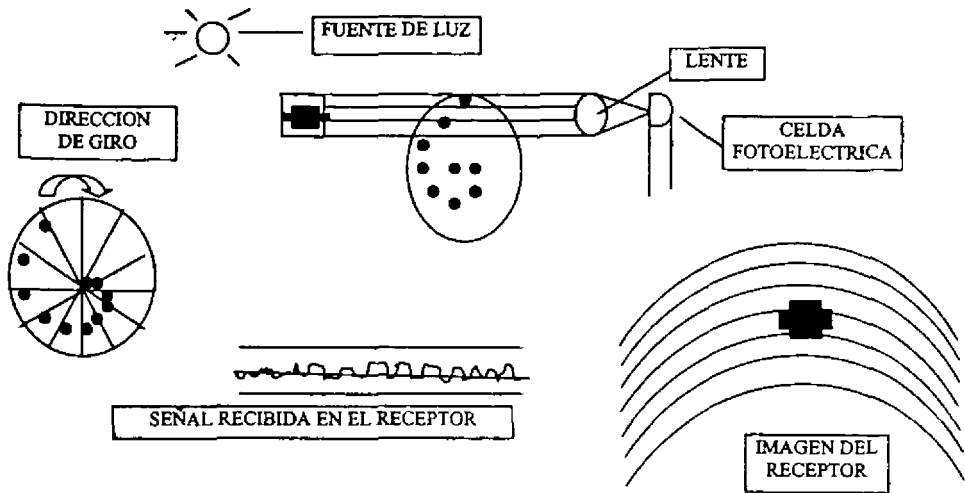
Figura 2.2. Analizador mecánico de Nipkow.
