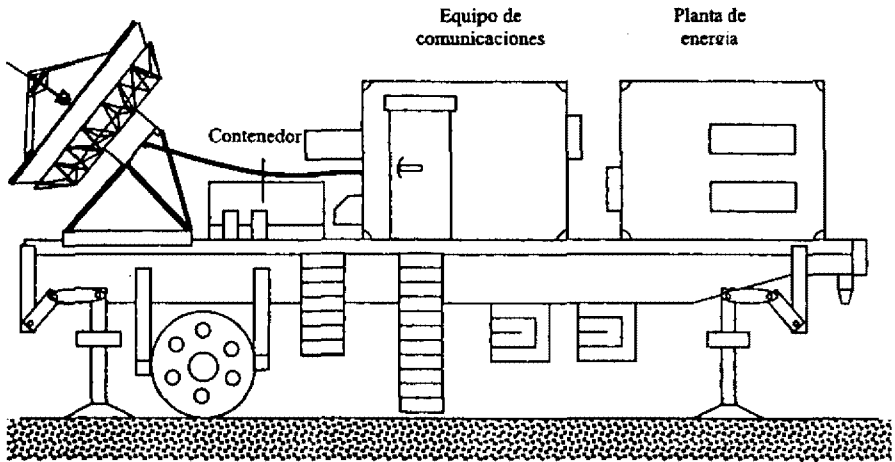
Figura 5.2. Primera generación de E/T móviles transportables.
