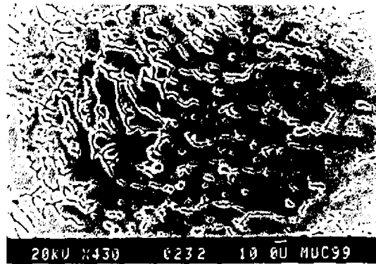
Foto 5.7: Baño fundido, zona de penetración y ZAC.
