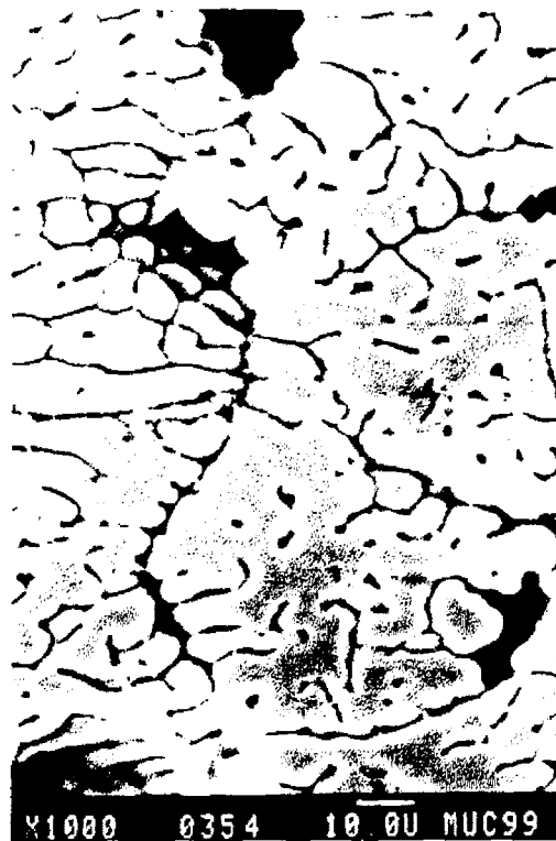
Foto 5.41: Crecimiento de una grieta en los espacios interdentriticos.
