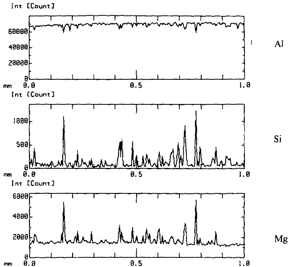
Gráfico 5.8: Perfil de concentraciones de Al, Si y Mg en el baño fundido, barrido en 1 mm de longitud sobre su superficie.
