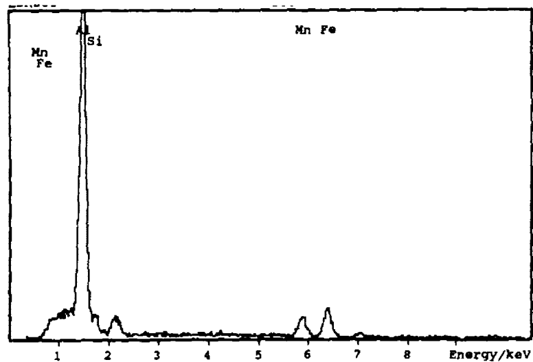
Gráfico 5.11: Intermetálico detectado de Al-Si-Mn-Fe por EDS en el material base.
