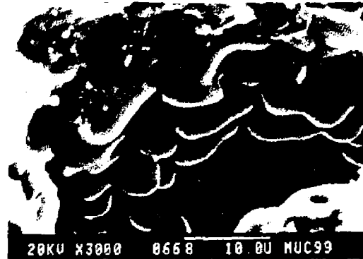
Foto 5.36: Superficie interior dendrítica de los poros.
