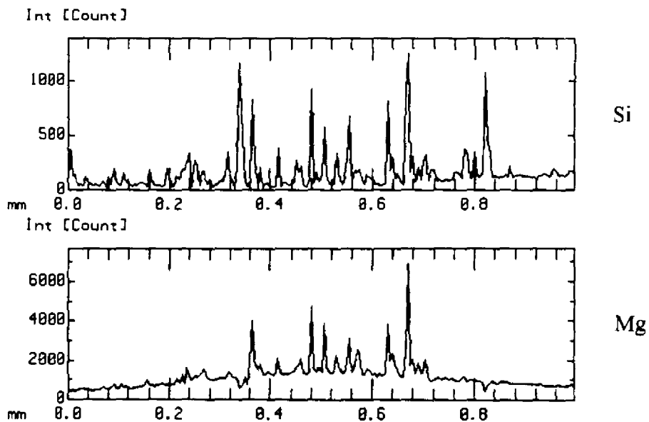
Gráfico 5.9: Perfil de concentraciones entre la ZAC y la línea de fusión.
