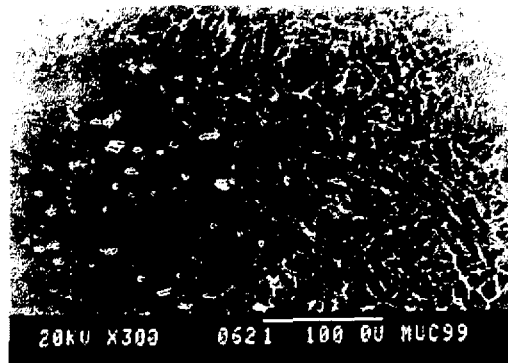
Foto 5.22: Zona de unión de ambos cordones (cara y raíz).
