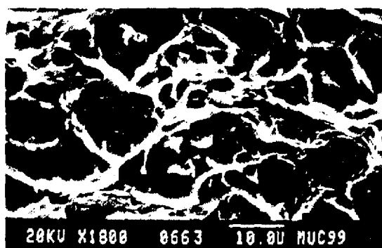
Foto 5.33: Precipitados de Mg_2Si .
