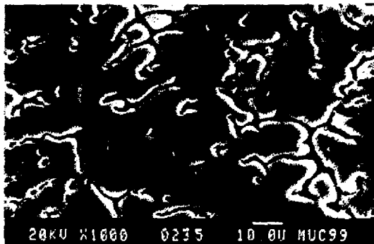
Foto 5.5: Detalle del baño fundido.
