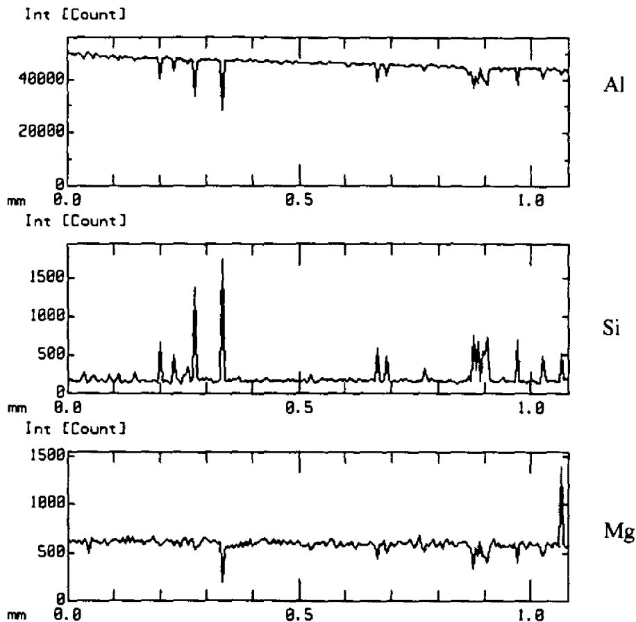
Gráfico 5.10: Perfil de concentraciones del material base AA6082.
