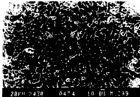
Foto 5.16: Baño fundido, fotografía tomada de SEM.
