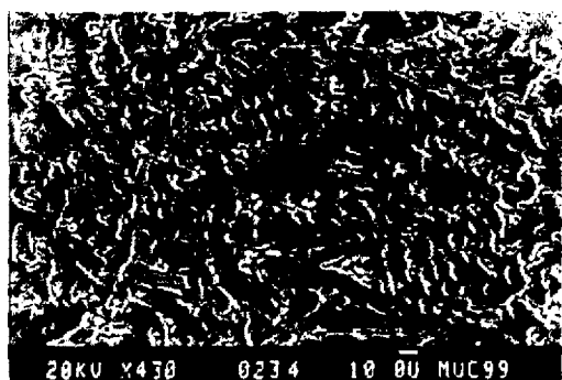
Foto 5.4: Baño fundido, zona central del cordón de soldadura.
