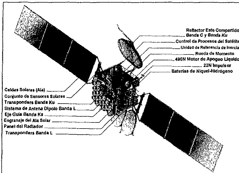
Ilustración 4.4.1 Estructura básica del satélite Solidaridad (HS-601)
