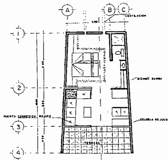
CUARTO TIPO ESC. 1:80
