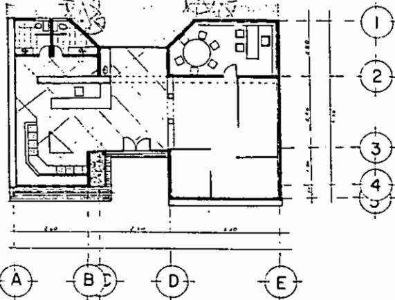
PLANTA AREA ADMINISTRATIVA
