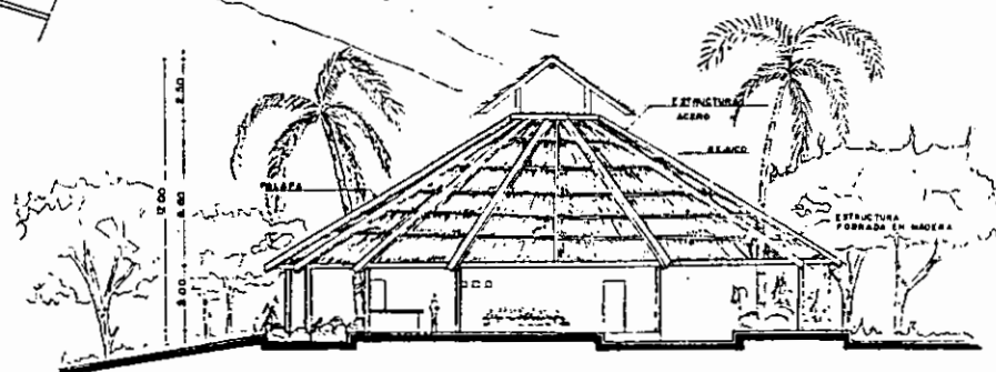
CORTE X-X
