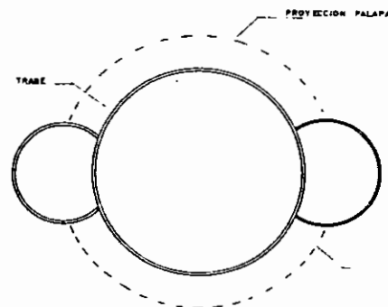
PLANTA ESTRUCTURAL
