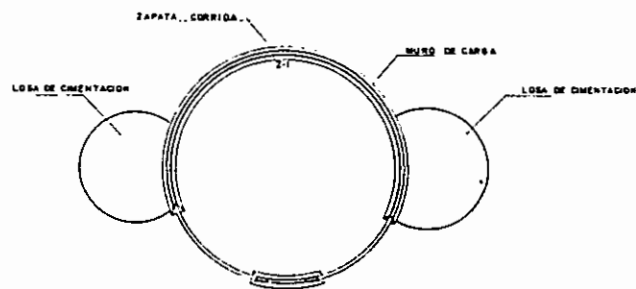
PLANTA CIMENTACION
