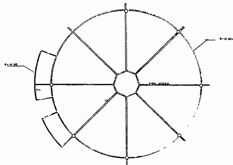
ESTRUCTURAL
