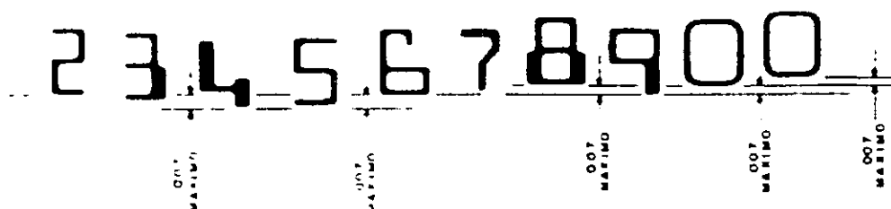
Figura 1.4.2.3.6.1 Alineación de los caracteres.
