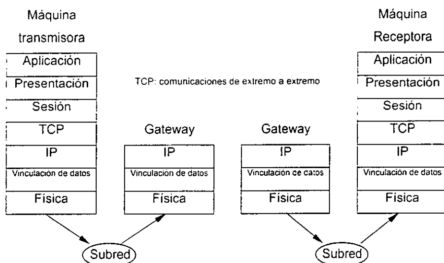
Figura 1.7.5.5.2.1. El TCP proporciona comunicación de extremo a extremo.
