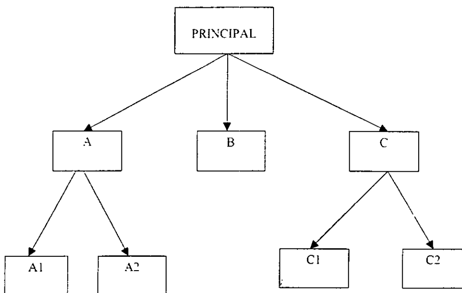
Figura 1.8.2.1.1 Diseño Modular.
