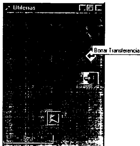
Figura 2.40 Borrar transferencia.
