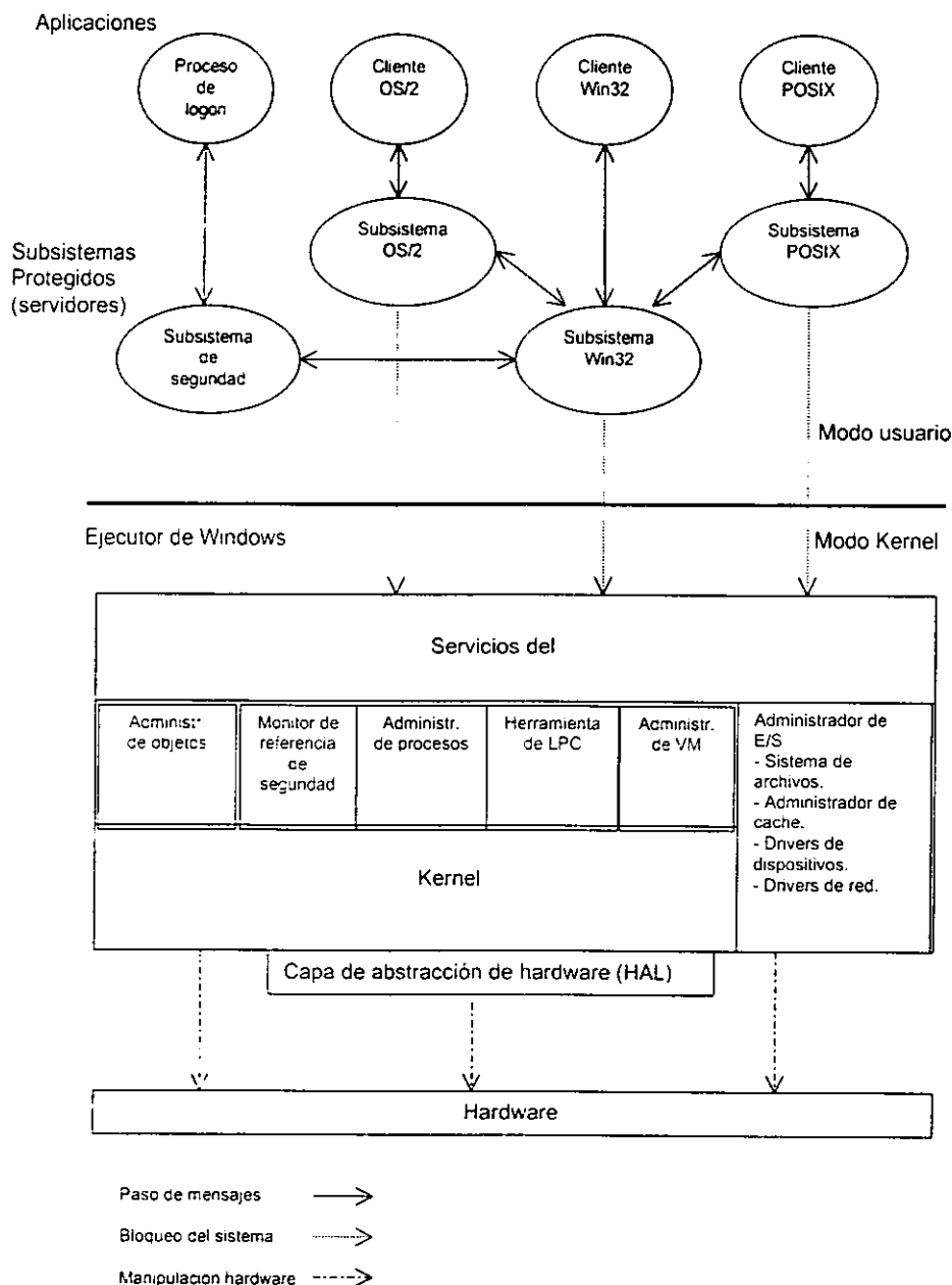
Figura 1.6.2.3.2.1 Estructura de Windows NT.
