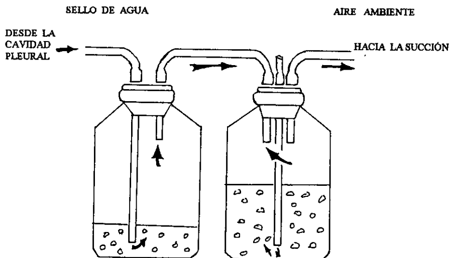
FIG. 2 A: SELLO CON DOS FRASCOS, UNO COLECTOR QUE SE CONECTA AL FRASCO REGULADOR QUE TIENE TRES TUBOS. EL PRIMERO PARA MEDIR LA PRESIÓN (20 cm. DE AGUA), UN SEGUNDO PARA SUCCIÓN Y EL TERCERO PARA EL COLECTOR.
