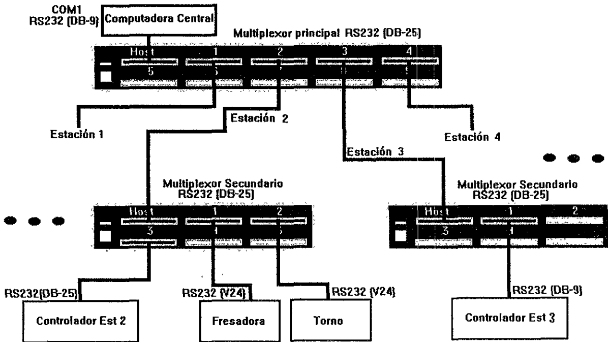
Figura A.4. Diagrama de conexiones entre el multiplexor central y los multiplexores secundarios.
