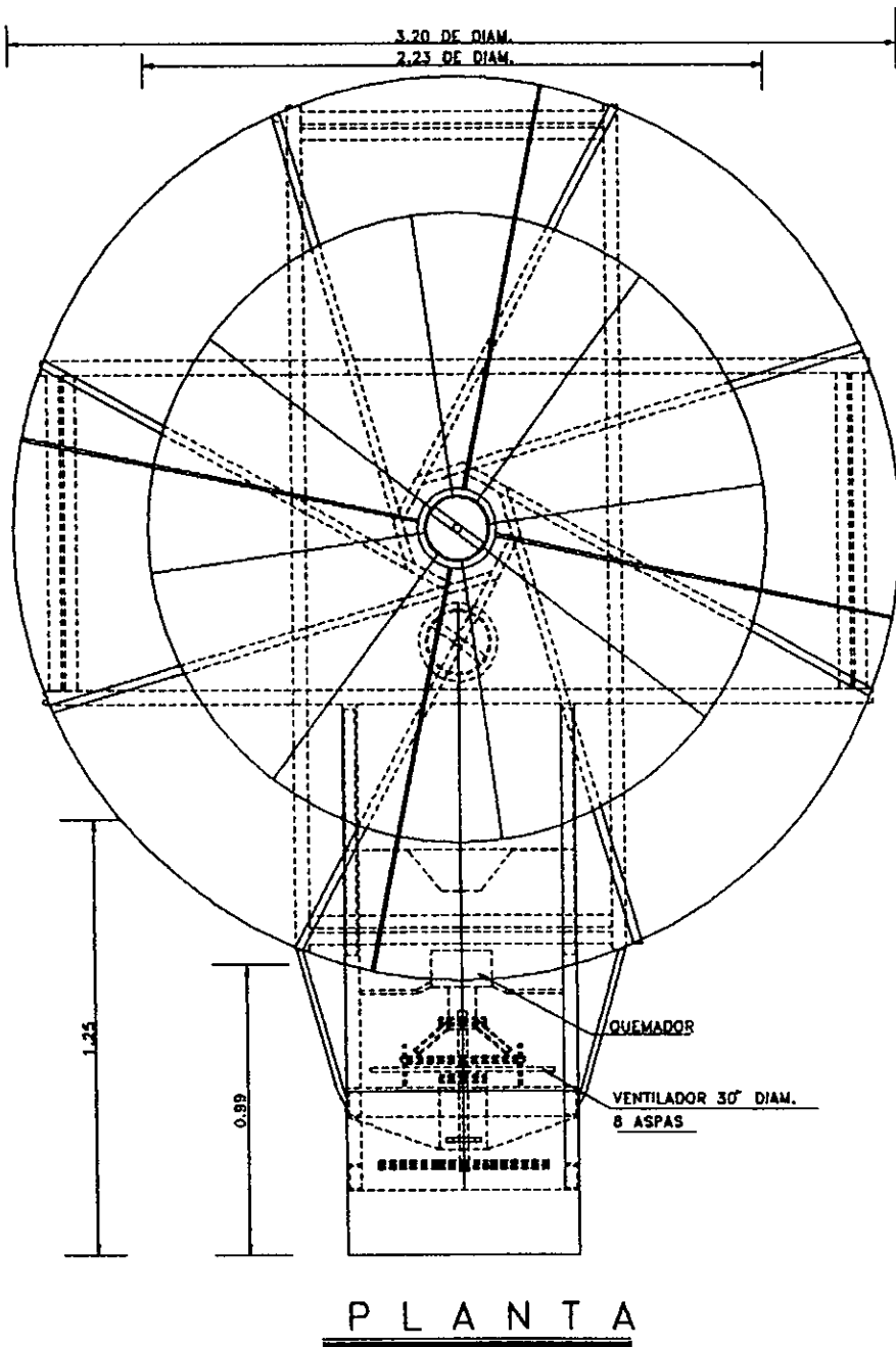
FIGURA 4.5 (b): SECADOR DE FLUJO CRUZADO
