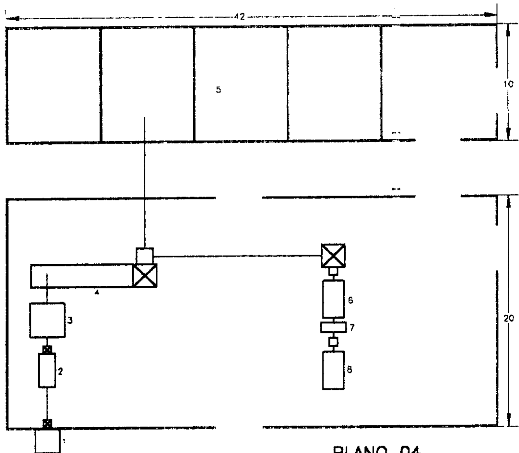
PLANO 04 AREA DE PROCESO
