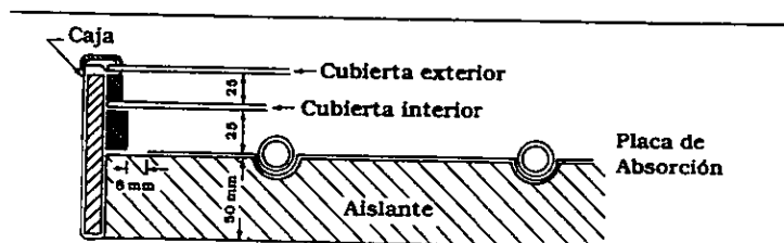
Corte transversal de un colector plano con dos cubiertas de vidrio.
