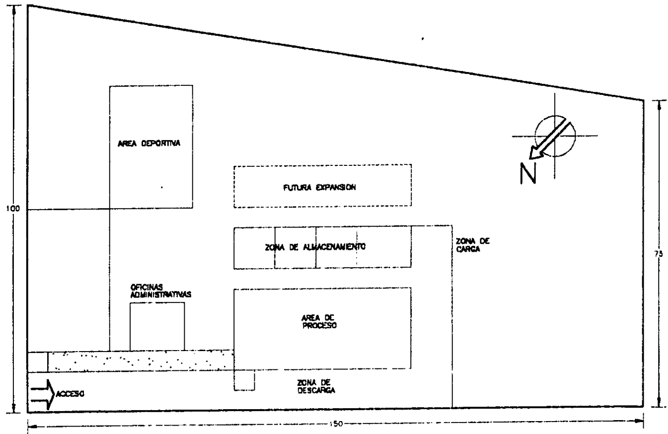
PLANO 03 DISTRIBUCION DE LAS AREAS DE TRABAJO
