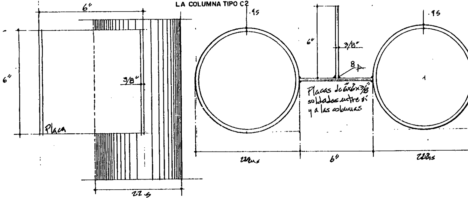
PLANTA Y ALZADO DE LA PLACA DE UNION DE LA COLUMNA TIPO C2
