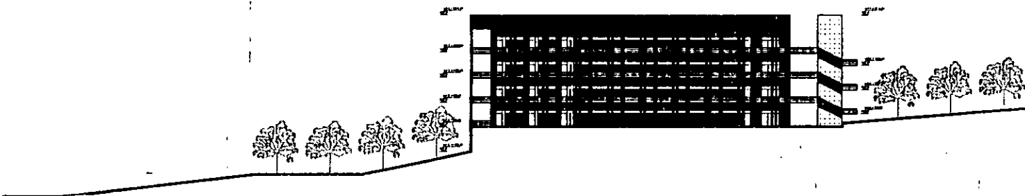
FACHADA ESTE DE LOS LABORATORIOS
